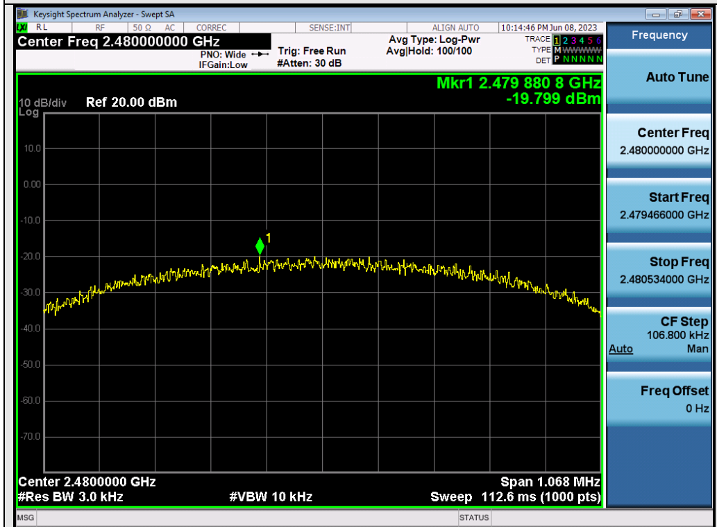
Test_Graph_ANT2_2480_PSD
