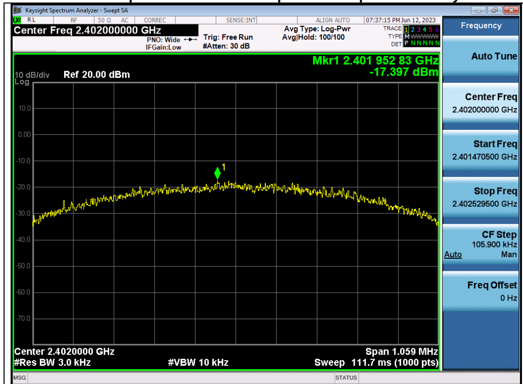
Test_Graph_ANT1_2402_PSD
