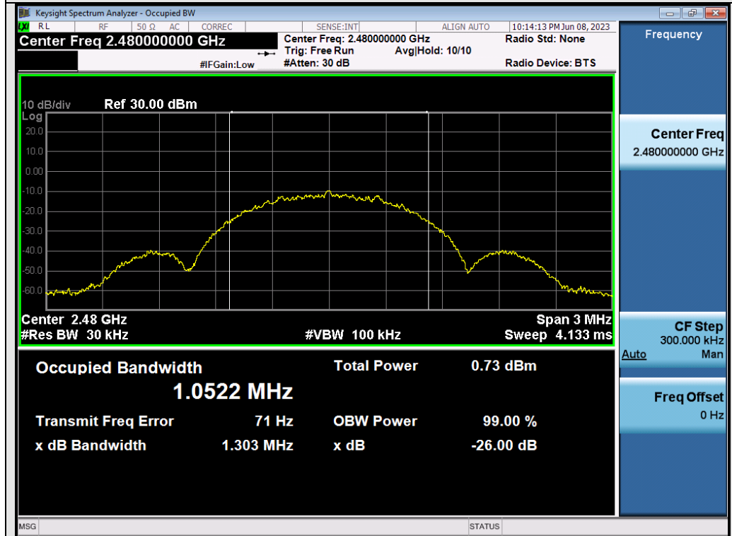
Test_Graph_ANT2_2480_OBW
