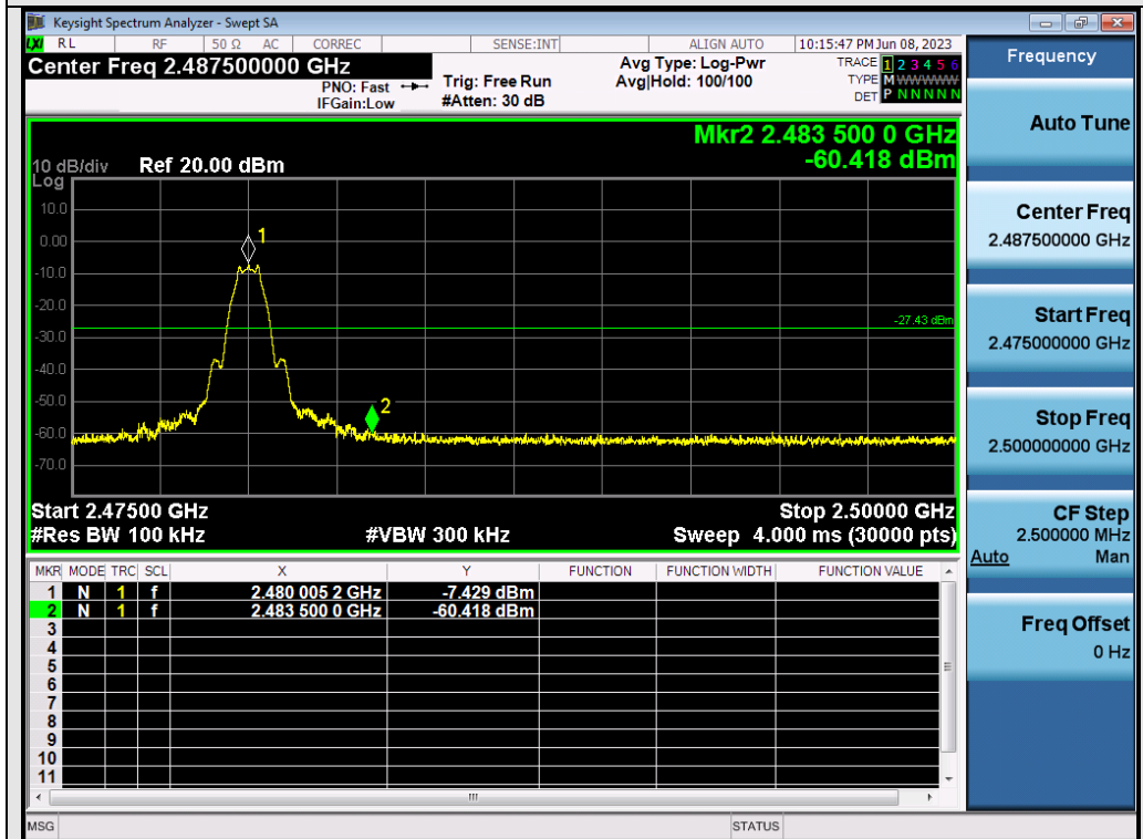
Test_Graph_ANT2_2480_Higher Band Edge Emissions
