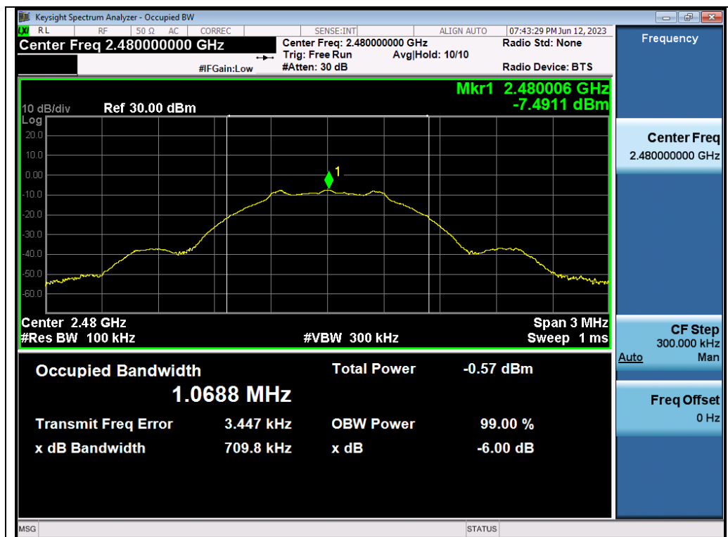
Test_Graph_ANT1_2480_DTSBW
