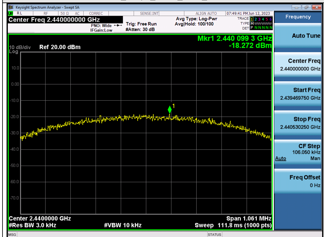
Test_Graph_ANT1_2440_PSD
