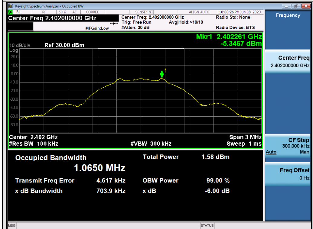
Test_Graph_ANT2_2402_DTSBW
