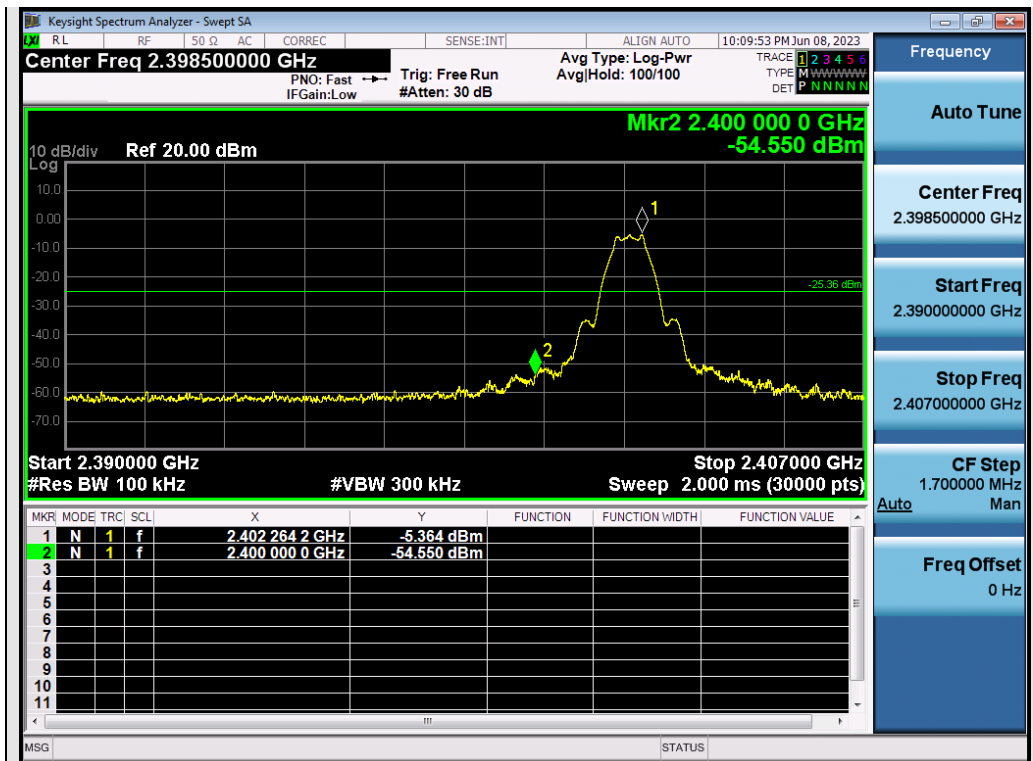
Test_Graph_ANT2_2402_Lower Band Edge Emissions
