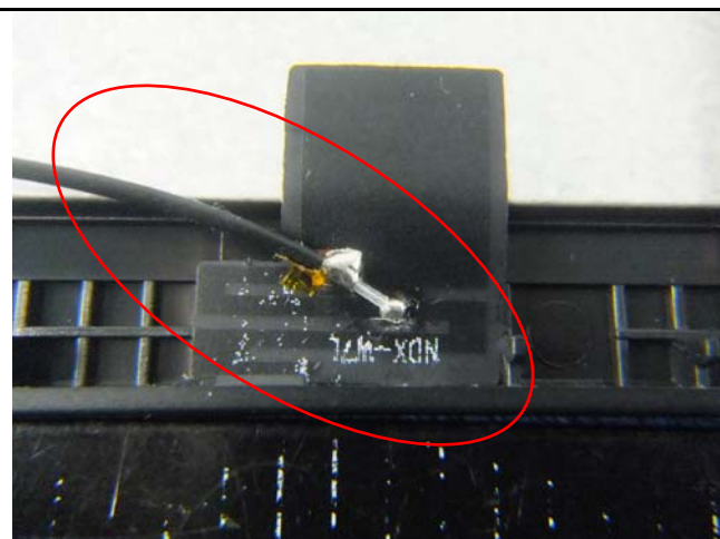
BT/WIFI/BLE Antenna View
