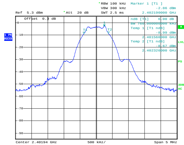
(Channel 37)
