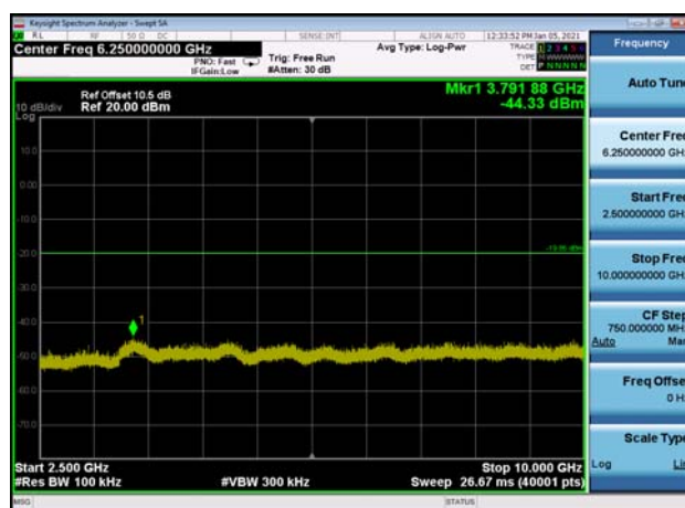
,Plot 4,2500MHz~10000MHz-802.11n(HT20) ,2462MHz
