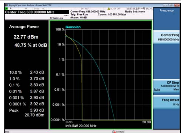
FDD71_HighRange_20MHz_688_fullIRB _Q16
