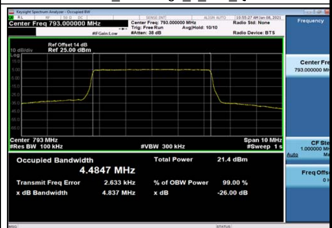
FDD14_MidRange_5_793_Q16
