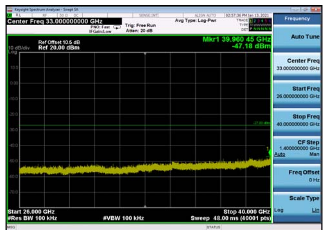
U-NII-3 ,Plot 2,26000MHz~40000MHz-802 .11ac(20MHz),5785MHz
