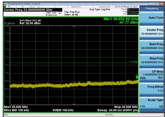
U-NII-3 ,Plot 2,26000MHz~40000MHz-802 .11a(20MHz),5825MHz
