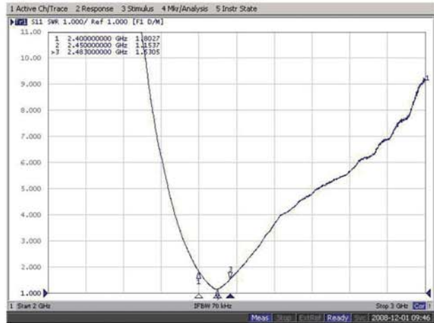
VSWR(S11)
