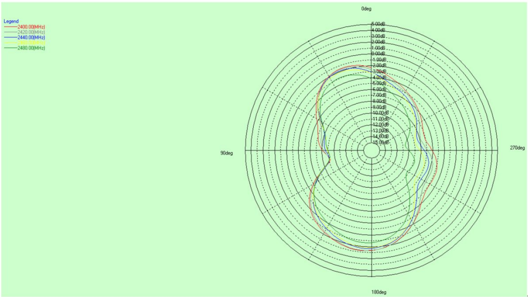
2.4G 俯仰面
