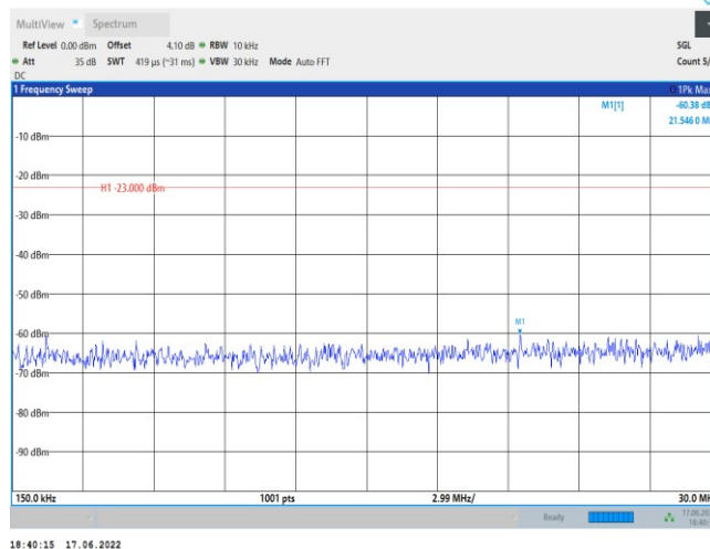
Band25-20MHz-QPSK-26140-1RB#0-Range2:0.15~30MHz
