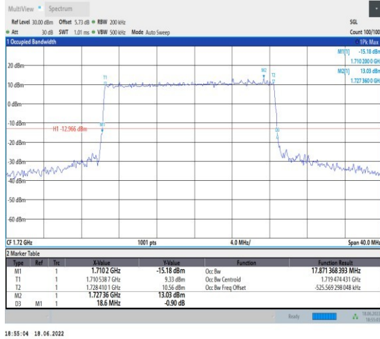
1-N66--15-20-L-4-DFT-64QAM-Outet_Full-100@0-A nt1-17.871-18.600-≤20-PASS
