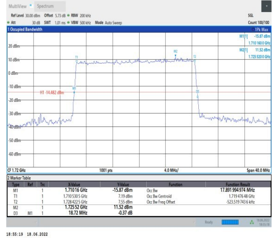
1-N66--15-20-L-5-DFT-256QAM-Outet_Full-100@0-A nt1-17.892-18.720-≤20-PASS
