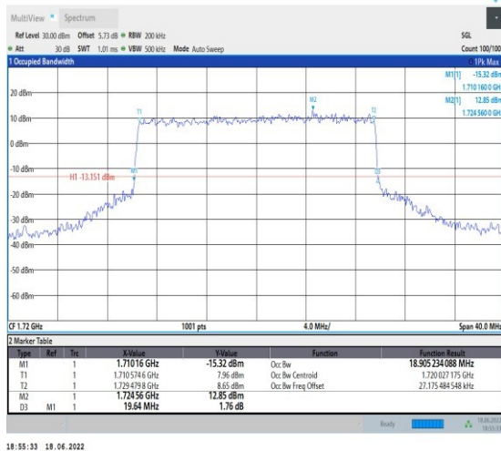
1-N66--15-20-L-6-CP-QPSK-Outet_Full-106@0-A nt1-18.905-19.640-≤20-PASS
