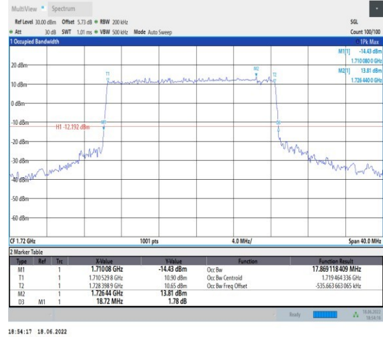
1-N66--15-20-L-1-DFT-QPSK-Outer_Full-100@0-Ant 1-17.869-18.720-≤20-PASS
