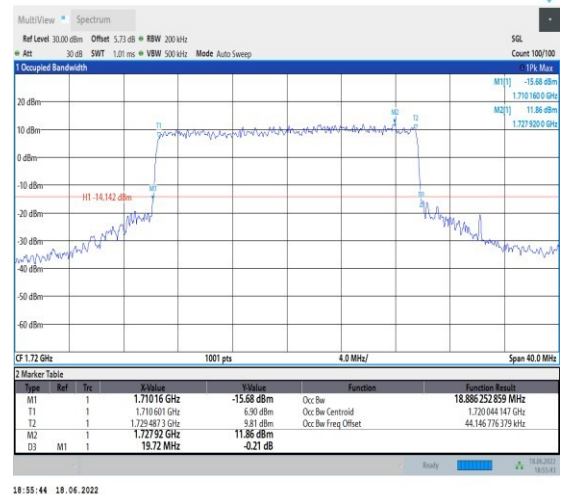
1-N66--15-20-L-7-CP-16QAM-Outet_Full-106@0-A nt1-18.886-19.720-≤20-PASS
