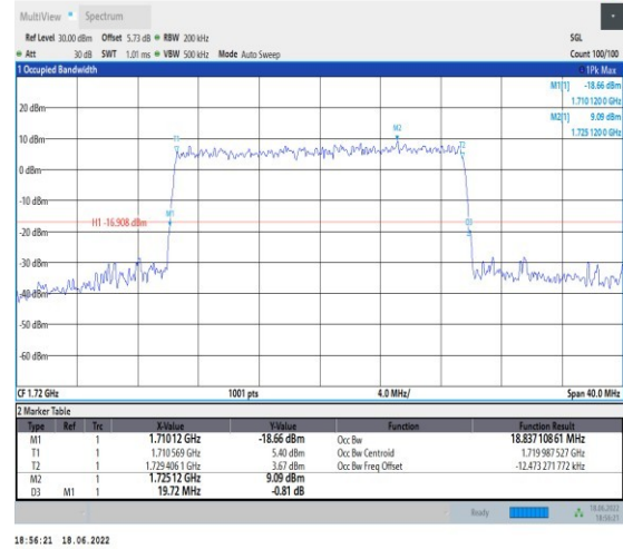
1-N66--15-20-L-9-CP-256QAM-Outer_Full-106@0-A nt1-18.837-19.720-≤20-PASS
