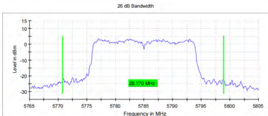
11N20_Ant0_5785
