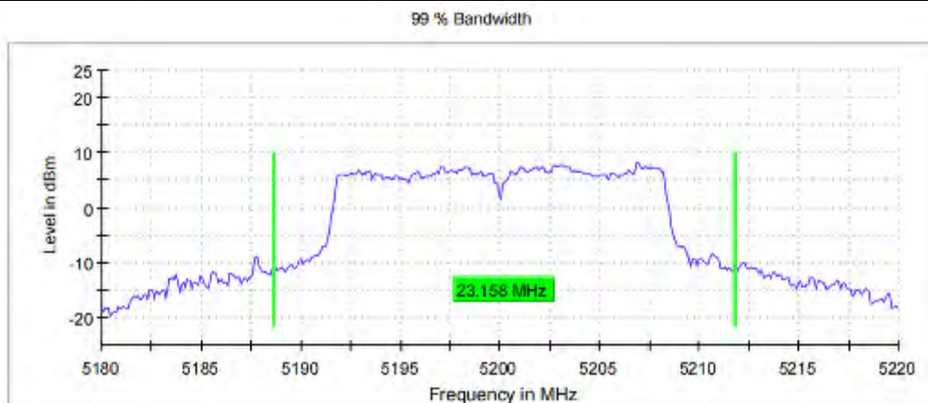
11A_Ant0_5200
