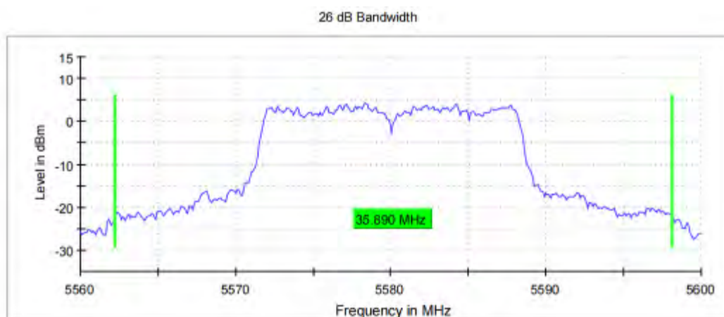
11A_Ant1_5580
