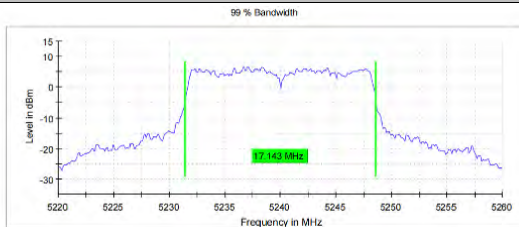
11A_Ant1_5240
