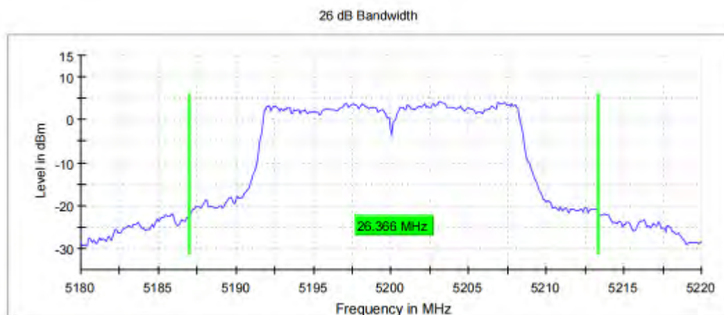
11A_Ant1_5200
