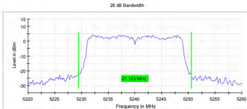
11N20_Ant1_5240
