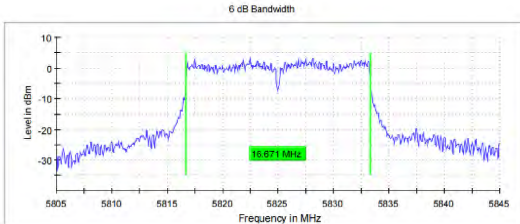
11A_Ant1_5825
