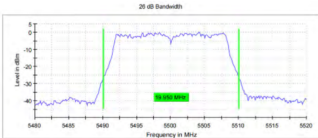
11A_Ant1_5500
