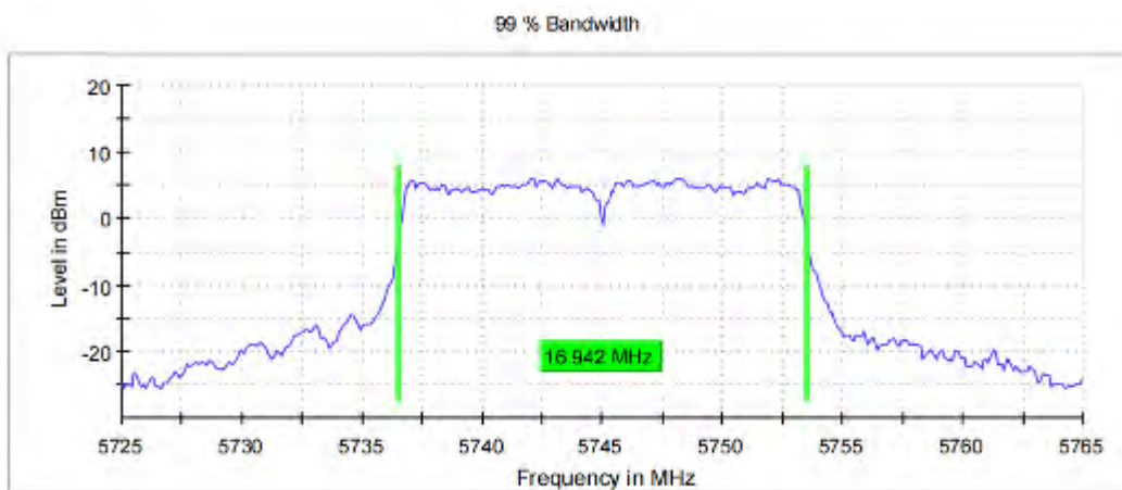
11A_Ant0_5745
