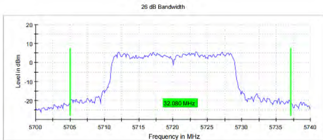
11N20_Ant1_5720
