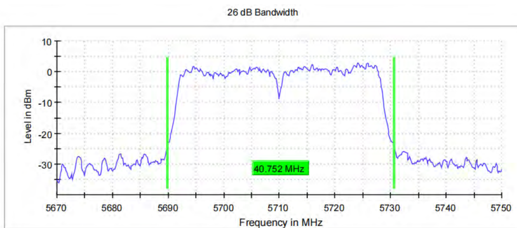
11N40_Ant1_5710
