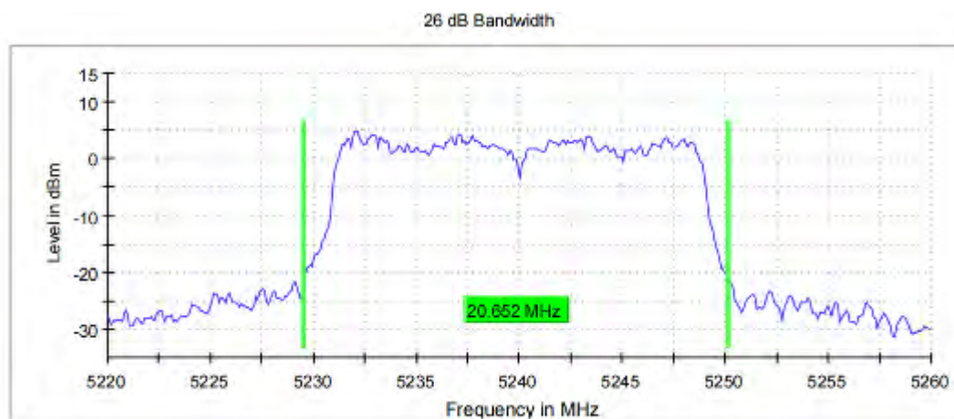
11N20_Ant1_5240
