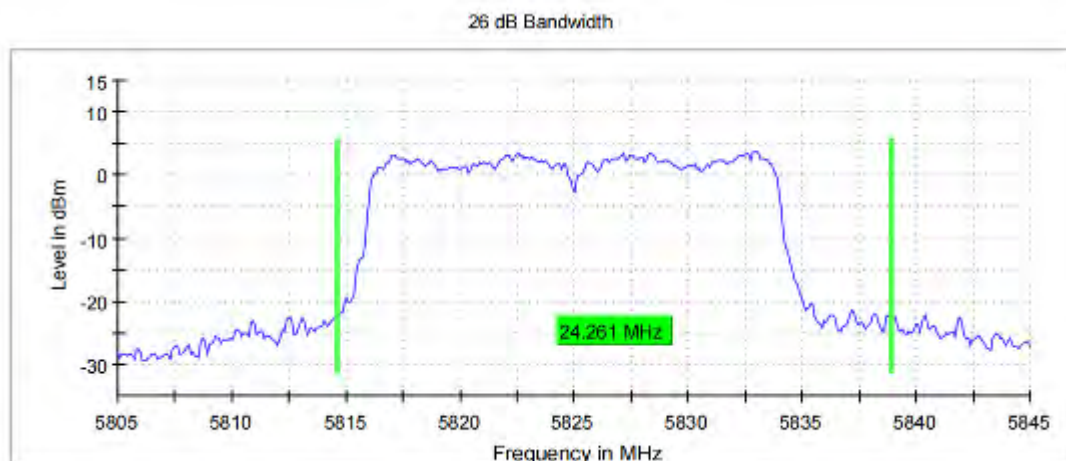
11N20_Ant1_5825
