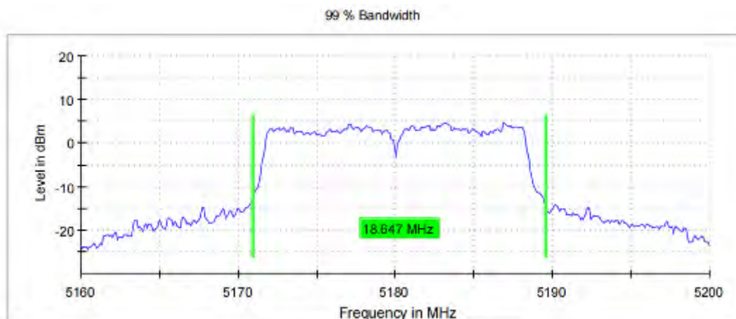
11A_Ant1_5180
