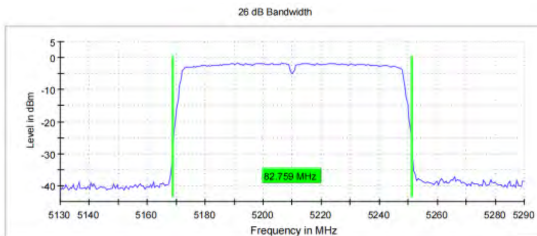
11AC80_Ant1_5210
