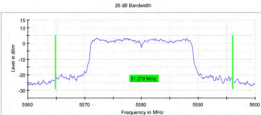
11N20_Ant0_5580
