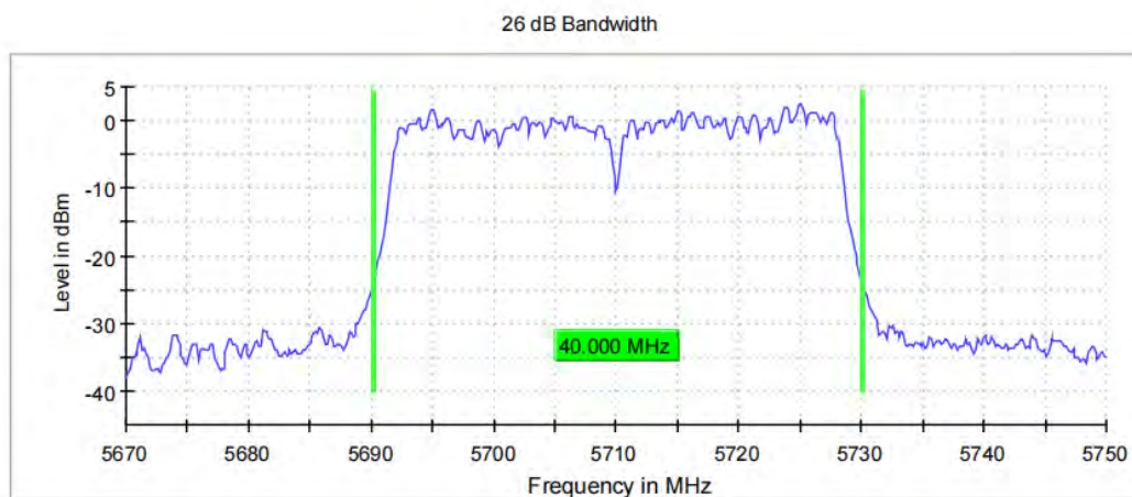
11N40_Ant0_5710
