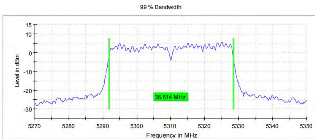
11N40_Ant0_5310
