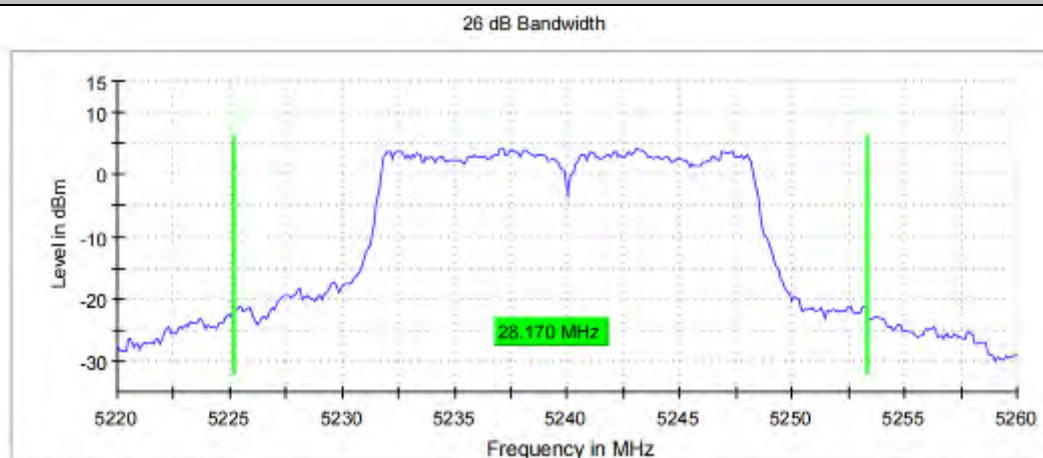
11A_Ant1_5240
