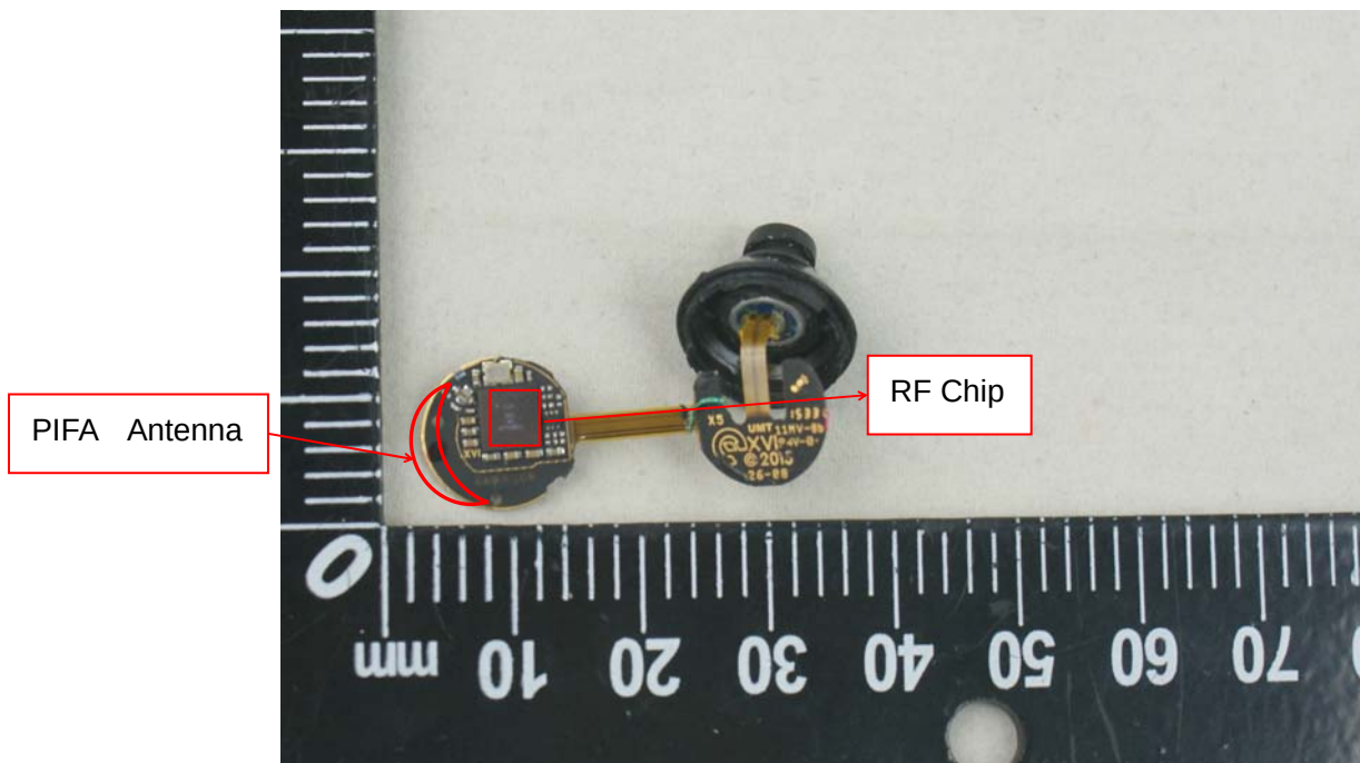
EUT Photo 6
