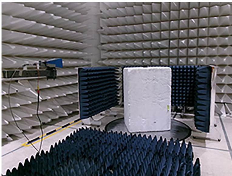
18GHz-26.5GHz
