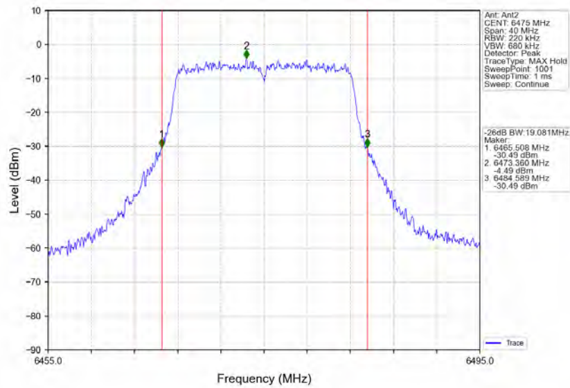
802.11a_MCH_6475MHz_Ant2_NTNV
