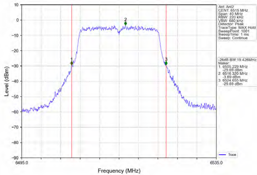
802.11a_HCH_6515MHz_Ant2_NTNV
