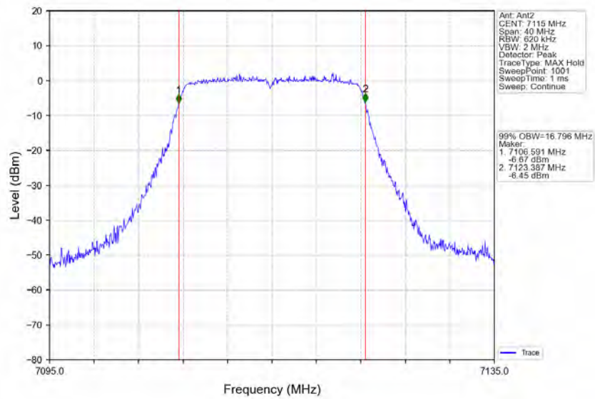
802.11a_HCH_7115MHz_Ant2_NTNV
