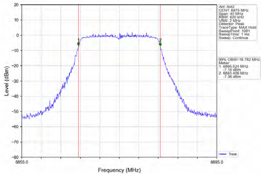
802.11a HCH 6875MHz Ant2 NTVN
