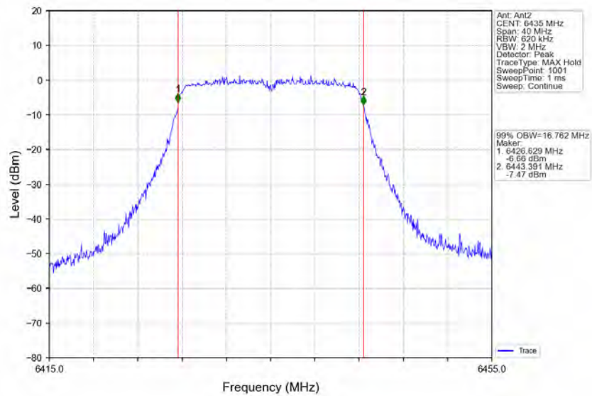
802.11a LCH 6435MHz Ant2 NTN
