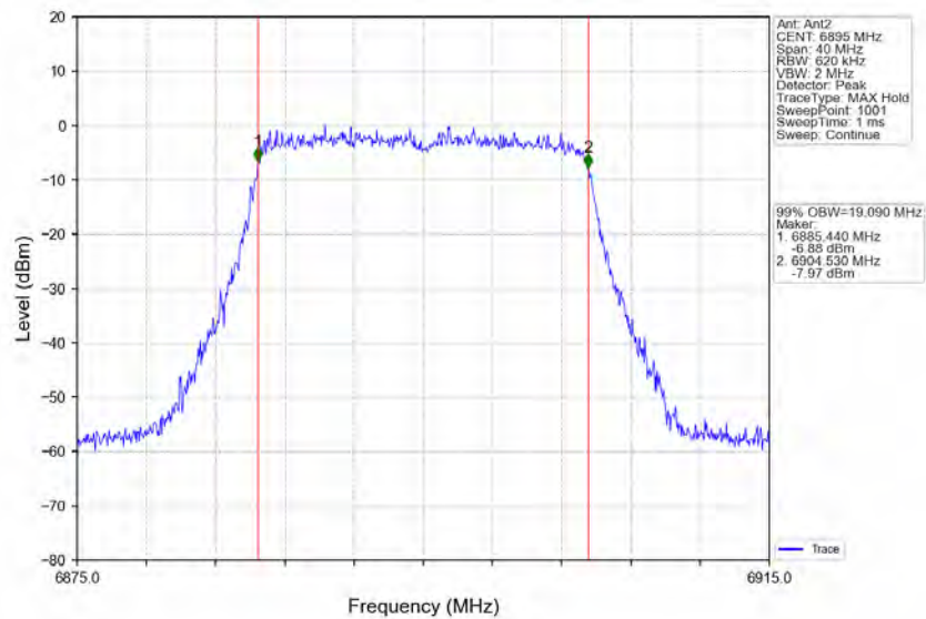
802.11ax(HEW20)_LCH_6895MHz_RU242_Left_Ant2_NTNV
