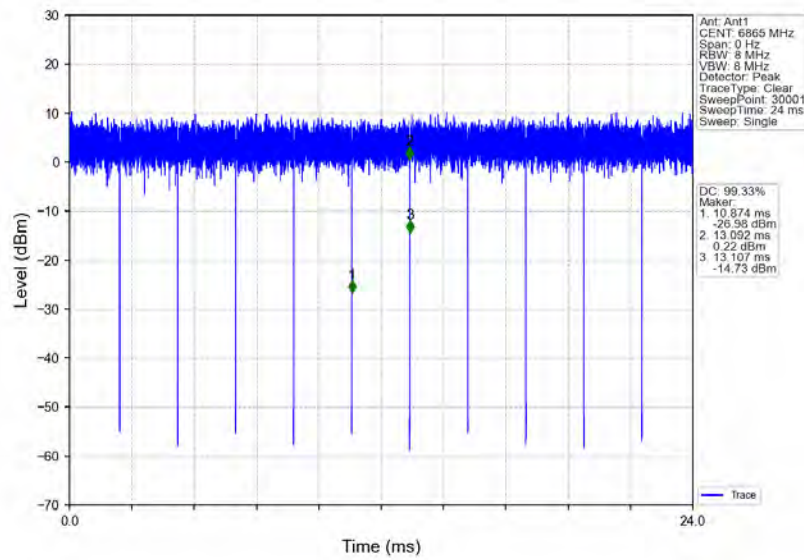
802.11ax(HEW80)_HCH_6865MHz_RU996_Left_Ant1_NTNV
