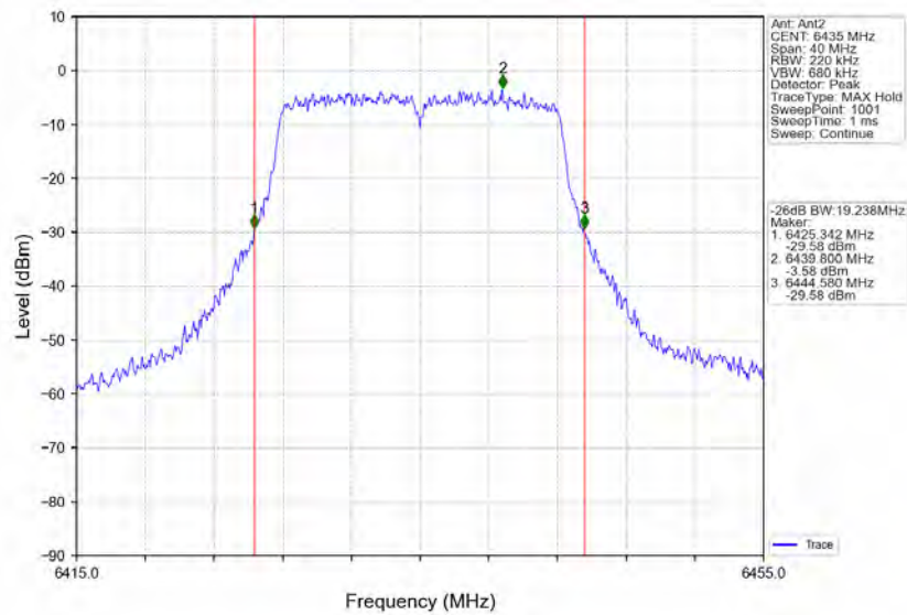
802.11a LCH 6435MHz Ant2 NTNV
