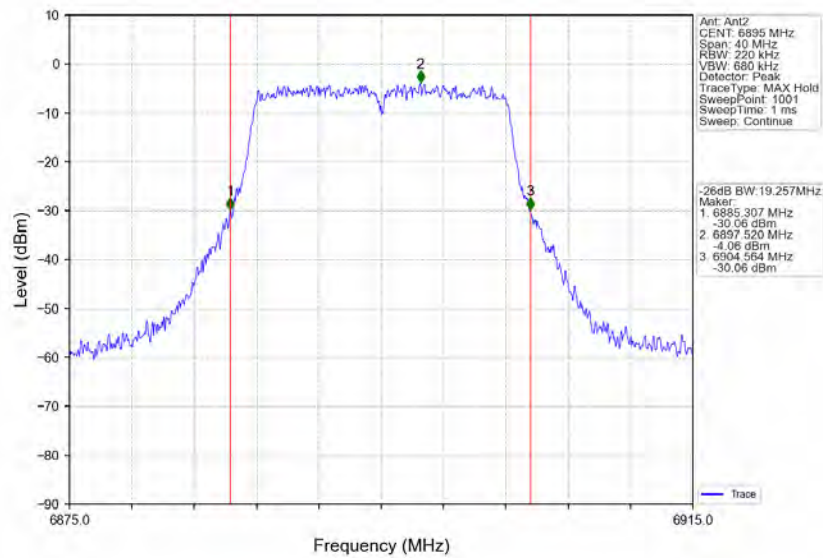
802.11a LCH 6895MHz Ant2 NTNV
