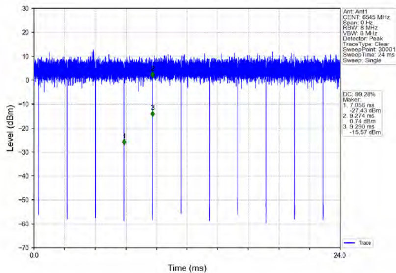
802.11ax(HEW80) HCH 6545MHz RU996 Left Ant1 NTNv
