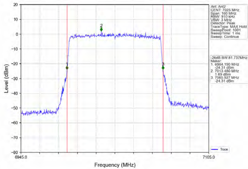
802.11ax(HEW80)_HCH_7025MHz_RU996_Left_Ant2_NTNV
