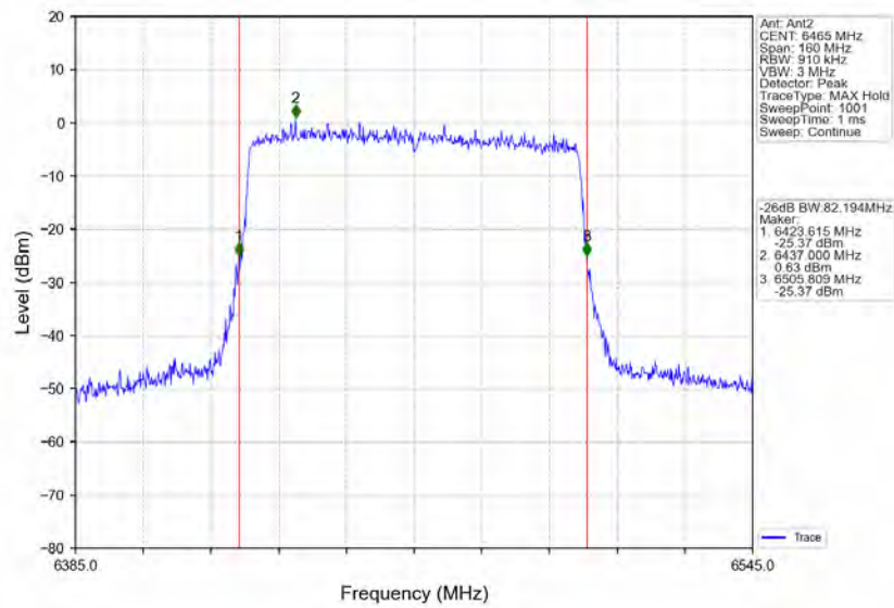
802.11ax(HEW80)_LCH_6465MHz_RU996_Left_Ant2_NTNV
