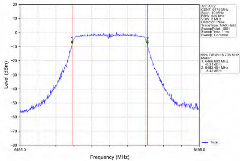
802.11a_MCH_6475MHz_Ant2_NTNV
