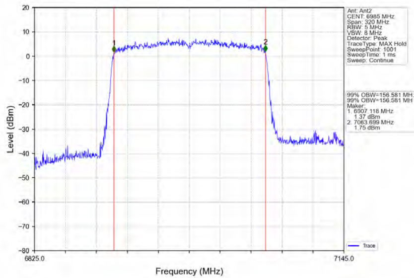
802.11ax(HEW160)_MCH_6985MHz_2xRU996_Left_Ant2_NTNV
