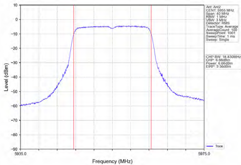
802.11a LCH 5955MHz Ant2 NTN
