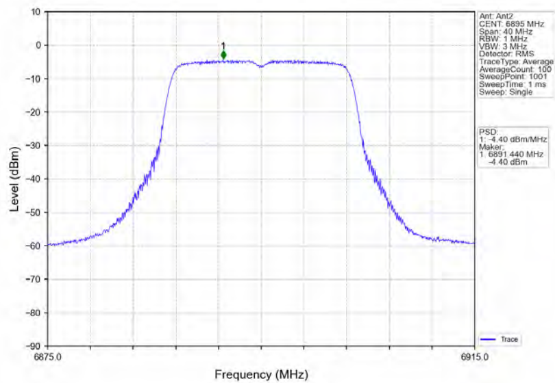
802.11a LCH 6895MHz Ant2 NTNV
