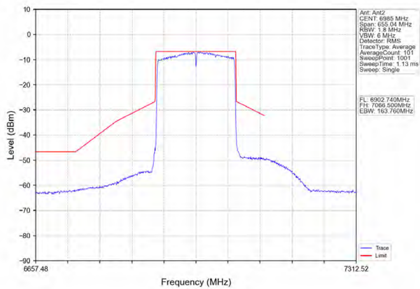
802.11ax(HEW160)_MCH_6985MHz_2xRU996_Left_Ant2_NTNV
