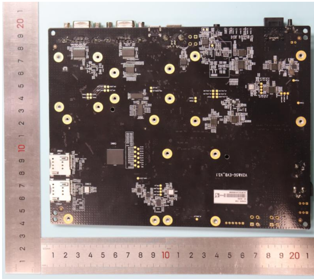
TAG555Q-GL + EVB _Bottom
