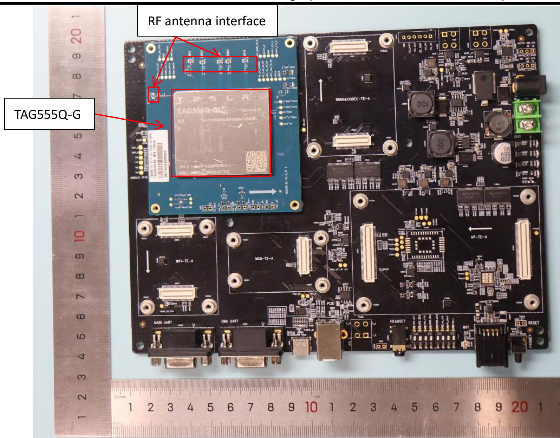
TAG555Q-GL + EVB_Top
