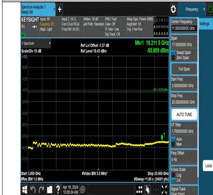
EGPRS1900-512-2-3000~20000MHz-PASS
