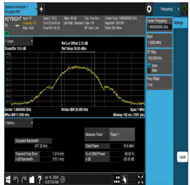
GPRS1900-661-0-PASS
