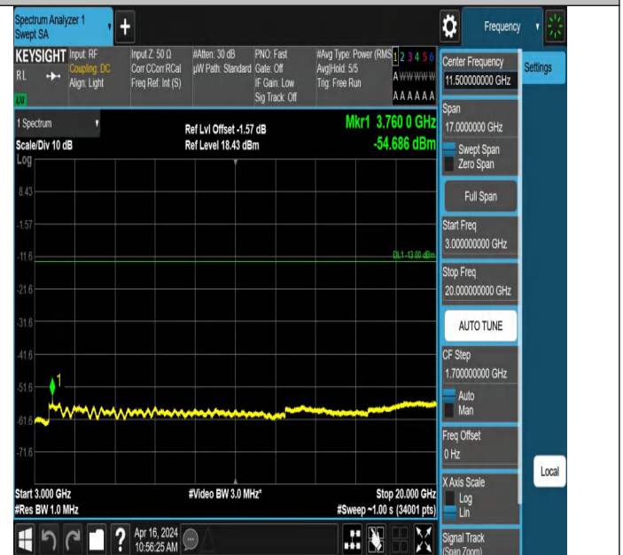
EGPRS1900-661-2-3000~20000MHz-PASS
