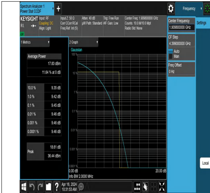
GSM1900-810-0-PASS
