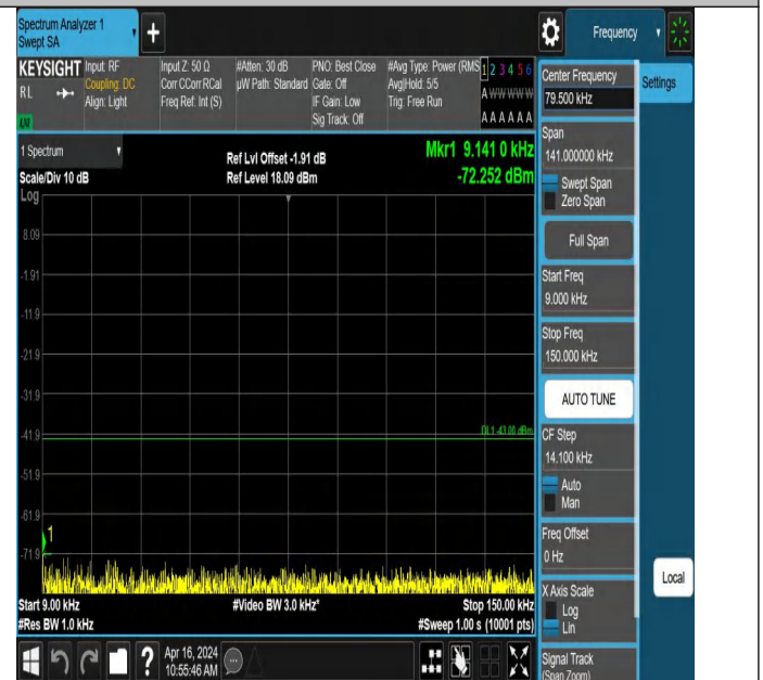
EGPRS1900-661-2-0.009~0.15MHz-PASS
