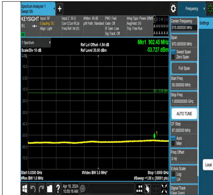
EGPRS1900-512-2-30~1000MHz-PASS
