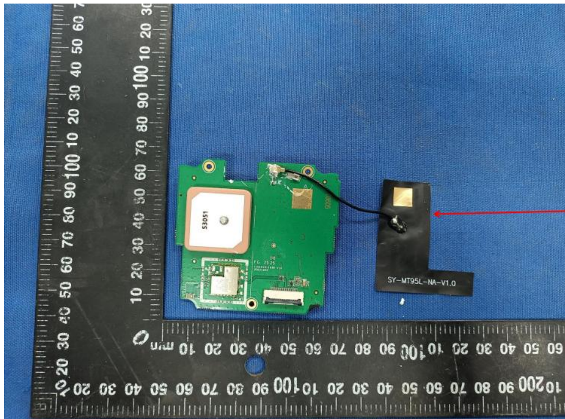
4G Antenna
