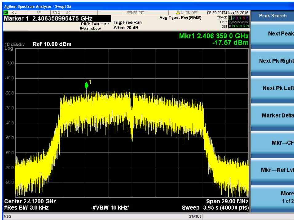
802.11n HT20
