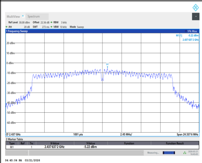
MIMO Ant. 2
