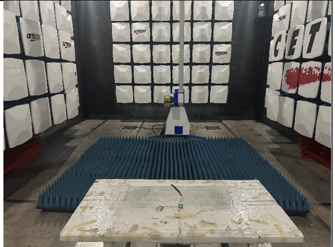
1GHz – 3GHz
