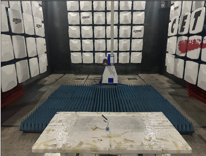
3GHz – 18GHz
