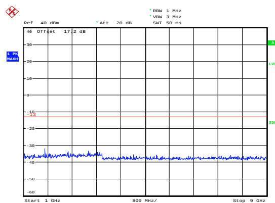
GSM 850 CH-High 1GHz ~ 9GHz
