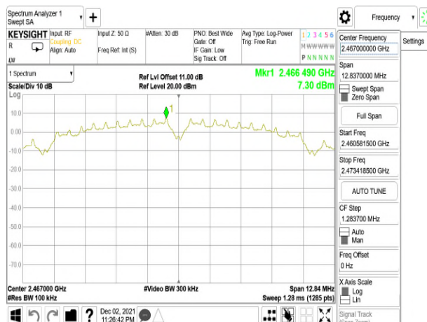
802.11b_20MHz_Chain0_2467MHz
