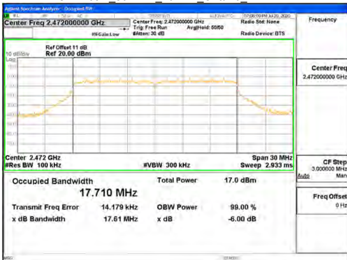
OBW 6dB_802.11n_20MHz_Chain0_2472MHz
