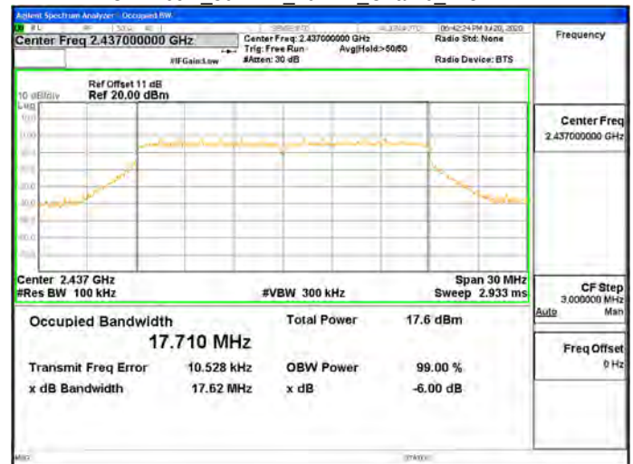
OBW 6dB_802.11n_20MHz_Chain0_2437MHz
