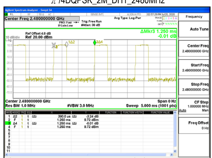
\pi /4DQPSK_2M_DH1_2480MHz
