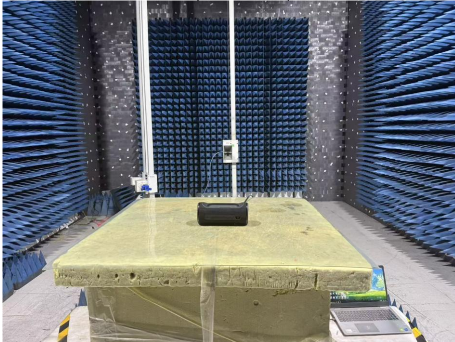
RE (1GHz-18GHz)
