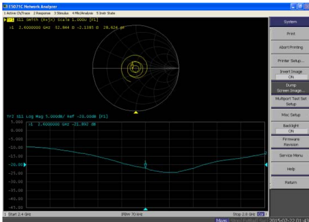
D2600MHz Body
