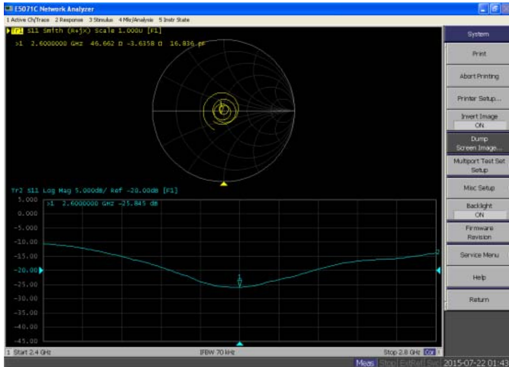
2600MHz head
