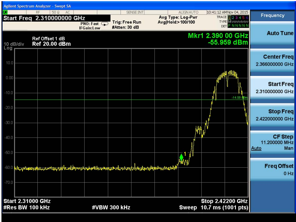
(Plot 4.5.2.1 A: Channel 01: 2412MHz @ 802.11 b )
