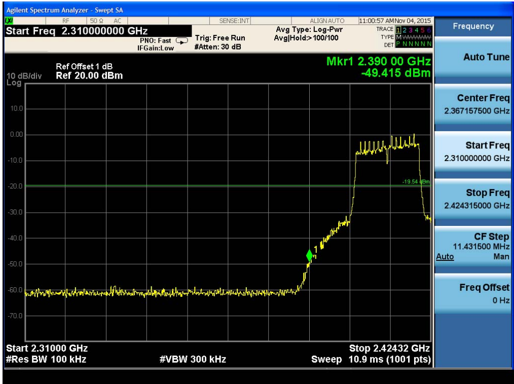
Plot 4.5.2.3 A: Channel 01: 2412MHz @ 802.11n HT20)
