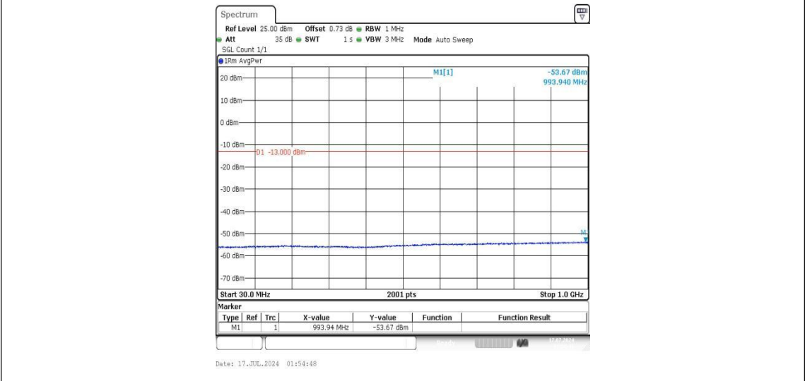
Band4-1513-2-30~1000MHz-PASS
