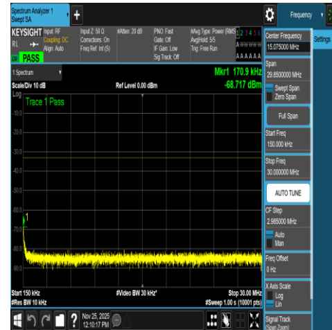
NTNV-N66-PC3-15-10-M-DFT-QPSK-Edge_1RB_ Left-0.15-30-Ant1-PASS
