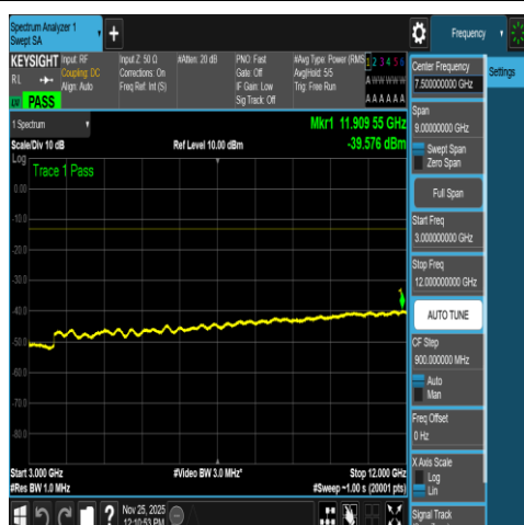
NTNV-N66-PC3-15-10-M-DFT-QPSK-Edge_1RB_ Left-3000-12000-Ant1-PASS
