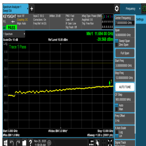
NTNV-N66-PC3-15-5-M-DFT-QPSK-Edge_1RB_L eft-3000-12000-Ant1-PASS
