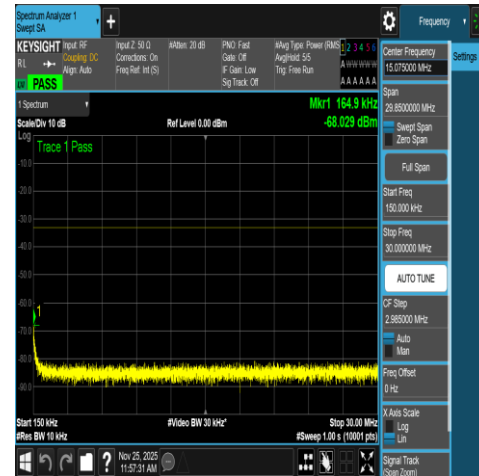
NTNV-N66-PC3-15-5-M-DFT-QPSK-Edge_1RB_L eft-0.15-30-Ant1-PASS
