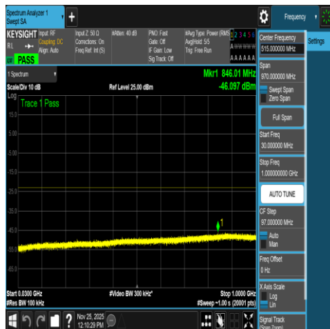
NTNV-N66-PC3-15-10-M-DFT-QPSK-Edge_1RB_ Left-30-1000-Ant1-PASS
