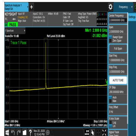
NTNV-N66-PC3-15-10-M-DFT-QPSK-Edge_1RB_ Left-1000-3000-Ant1-PASS
