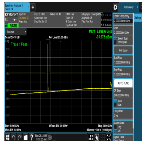
NTNV-N66-PC3-15-5-M-DFT-QPSK-Edge_1RB_L eft-1000-3000-Ant1-PASS
