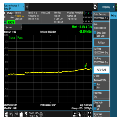
NTNV-N66-PC3-15-5-M-DFT-QPSK-Edge_1RB_L eft-12000-20000-Ant1-PASS
