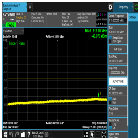
NTNV-N66-PC3-15-5-M-DFT-QPSK-Edge_1RB_L eft-30-1000-Ant1-PASS
