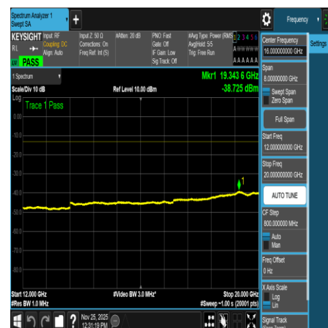
NTNV-N66-PC3-15-20-L-DFT-QPSK-Outter_Full-1 2000-20000-Ant1-PASS
