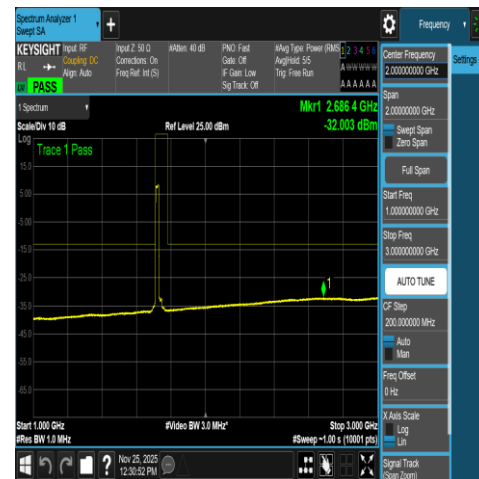
NTNV-N66-PC3-15-20-L-DFT-QPSK-Outter_Full-1 000-3000-Ant1-PASS
