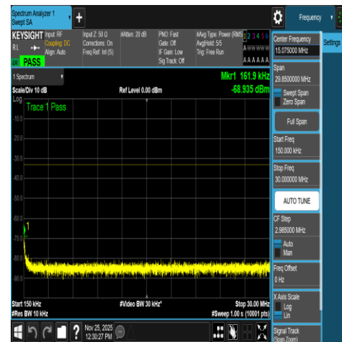
NTNV-N66-PC3-15-20-L-DFT-QPSK-Outter_Full-0. 15-30-Ant1-PASS
