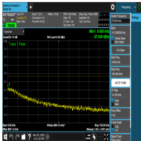
NTNV-N66-PC3-15-20-L-DFT-QPSK-Edge_1RB_ Left-0.009-0.15-Ant1-PASS
