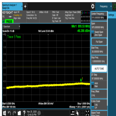
NTNV-N66-PC3-15-20-H-DFT-QPSK-Edge_1RB_ Left-30-1000-Ant1-PASS
