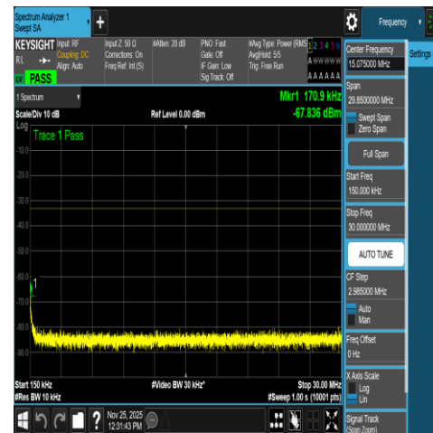
NTNV-N66-PC3-15-20-L-DFT-QPSK-Edge_1RB_ Left-0.15-30-Ant1-PASS
