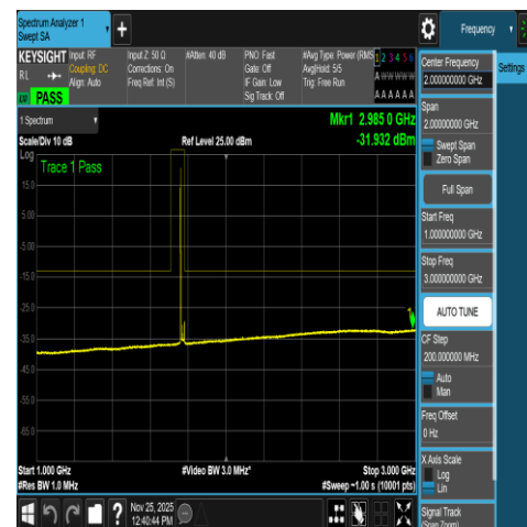
NTNV-N66-PC3-15-20-H-DFT-QPSK-Edge_1RB_ Left-1000-3000-Ant1-PASS
