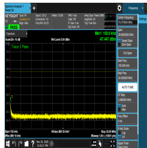
NTNV-N66-PC3-15-20-H-DFT-QPSK-Edge_1RB_ Left-0.15-30-Ant1-PASS
