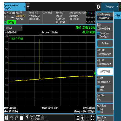
NTNV-N66-PC3-15-20-L-DFT-QPSK-Edge_1RB_ Left-1000-3000-Ant1-PASS
