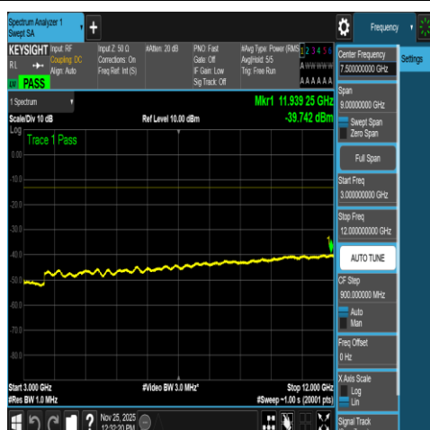
NTNV-N66-PC3-15-20-L-DFT-QPSK-Edge_1RB_ Left-3000-12000-Ant1-PASS
