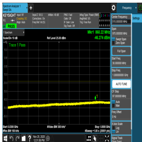
NTNV-N66-PC3-15-20-L-DFT-QPSK-Edge_1RB_ Left-30-1000-Ant1-PASS
