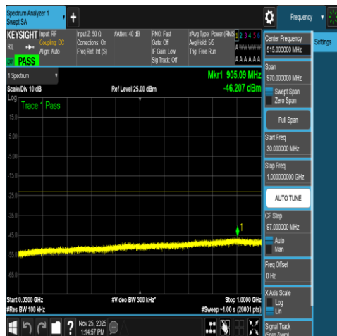
NTNV-N66-PC3-15-40-M-DFT-QPSK-Edge_1RB_ Left-30-1000-Ant1-PASS
