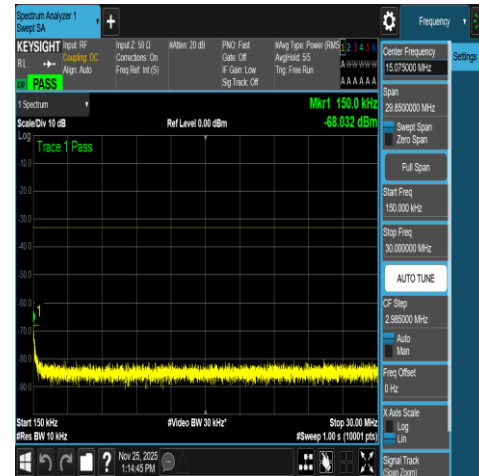
NTNV-N66-PC3-15-40-M-DFT-QPSK-Edge_1RB_ Left-0.15-30-Ant1-PASS
