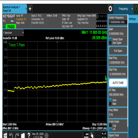
NTNV-N66-PC3-15-40-M-DFT-QPSK-Edge_1RB_ Left-3000-12000-Ant1-PASS
