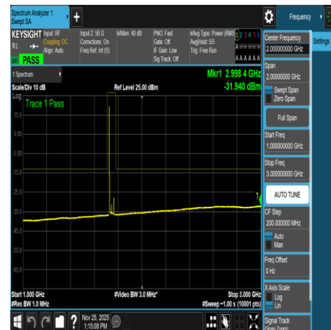
NTNV-N66-PC3-15-40-M-DFT-QPSK-Edge_1RB_ Left-1000-3000-Ant1-PASS
