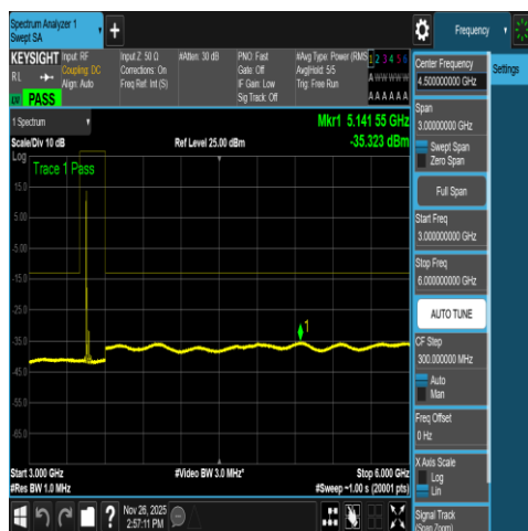
NTNV-DC_66A_n78A-3450-3550-PC2-30-5+40-M +L-N/A-N/A-DFT-QPSK-Edge_1RB_Left-3000-600 O-PASS
