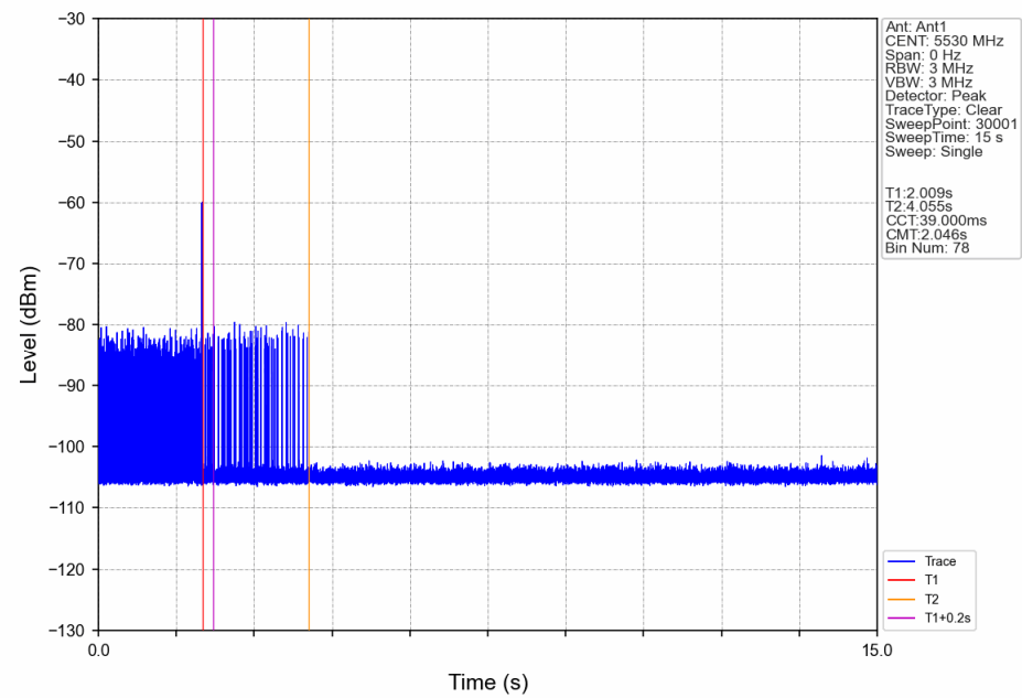
802.11ac80 channel 106 5530MHz
