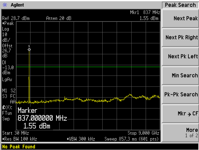
LTE 1.4MHz 16QAM
