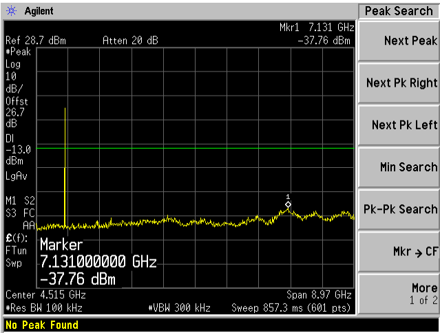
LTE 5MHz 64QAM
