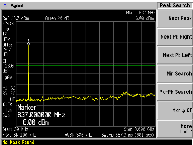
UL Middle 30MHz-9GHz
