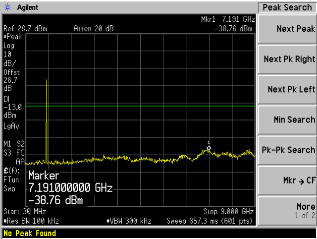
UL High 30MHz-9GHz
