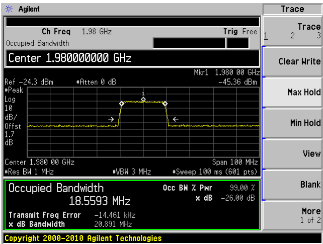
LTE 20MHz 64QAM UL
