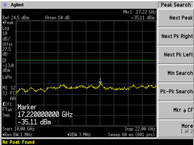
Middle 10MHz-22GHz
