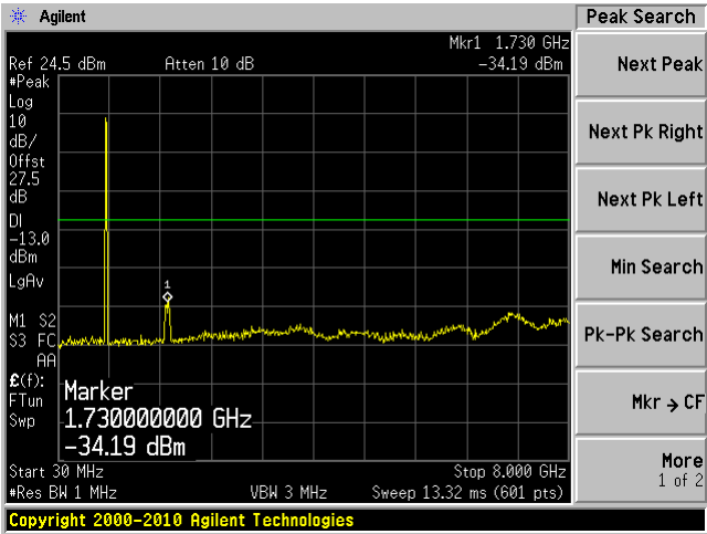
Low 30MHz-8GHz UL
