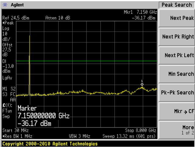
High 30MHz-8GHz UL
