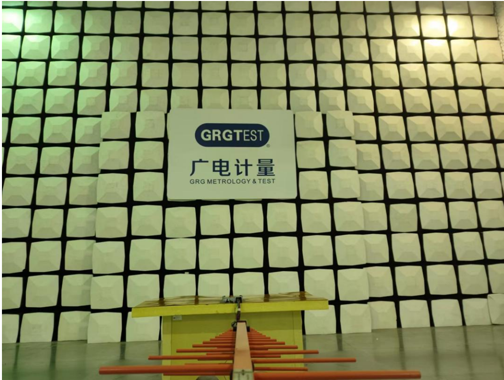
30MHz ~ 1GHz
