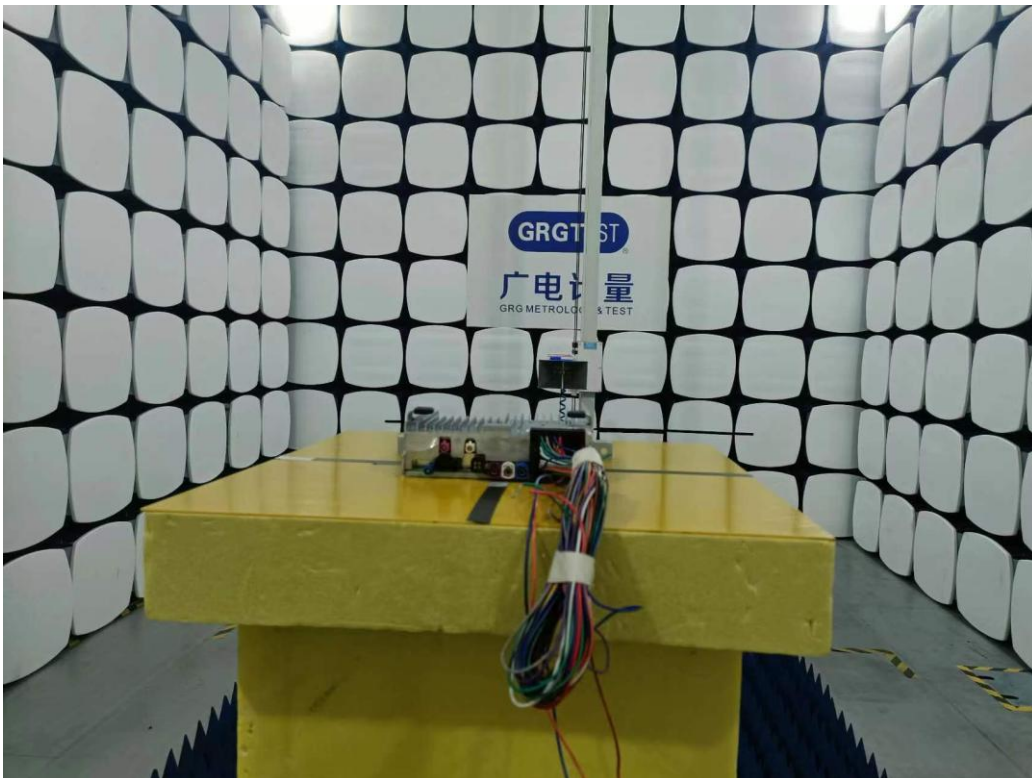
1GHz ~18GHz
