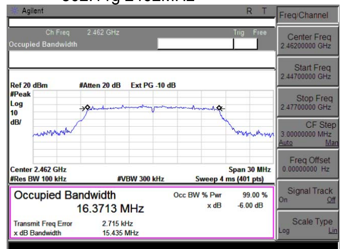
802.11g 2462MHz
