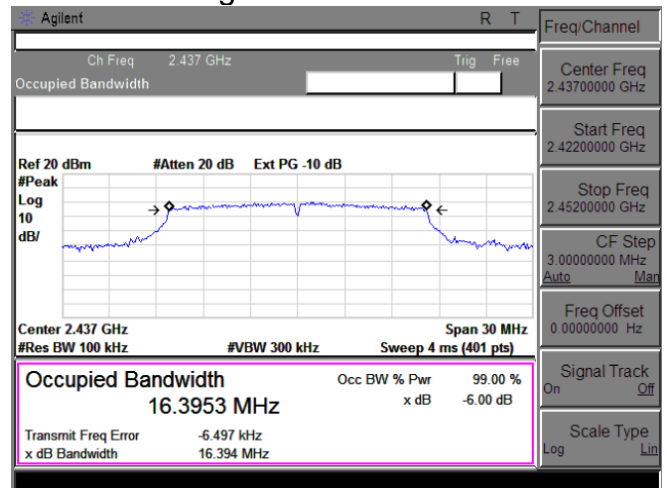
802.11g 2437MHz
