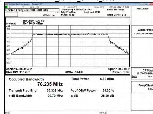
802.11ac 80MHz Chain0 6385MHz
