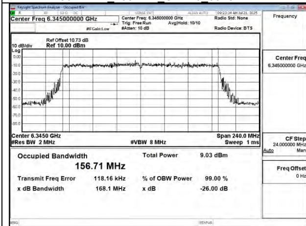
802.11be 160MHz Chain0 6345MHz
