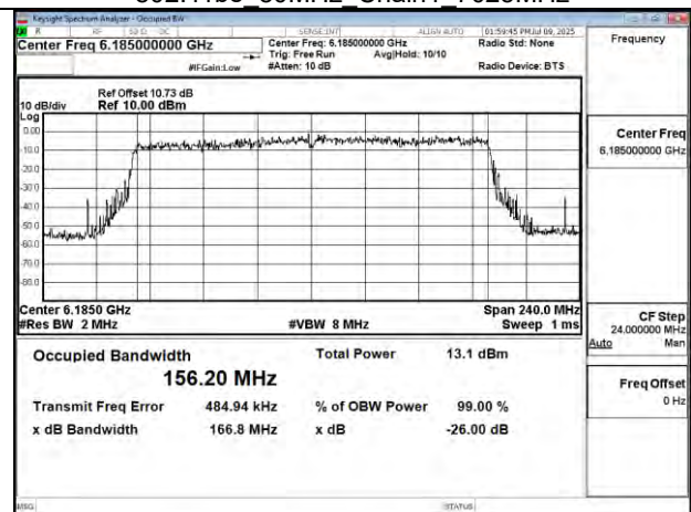
802.11be 160MHz Chain0 6185MHz
