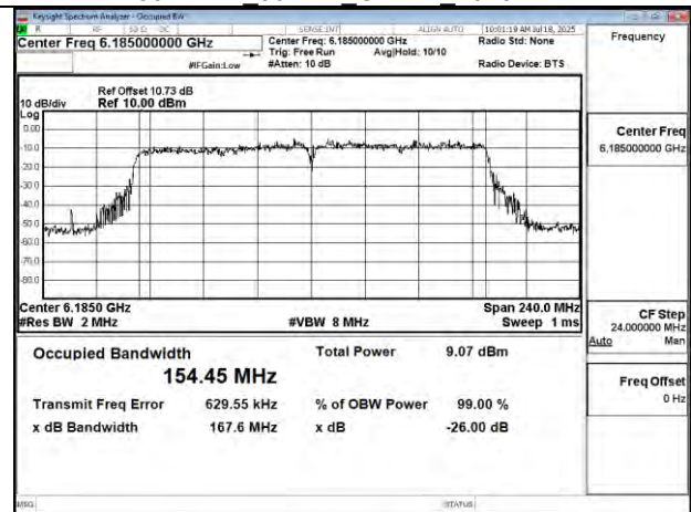
802.11ac 160MHz Chain0 6185MHz
