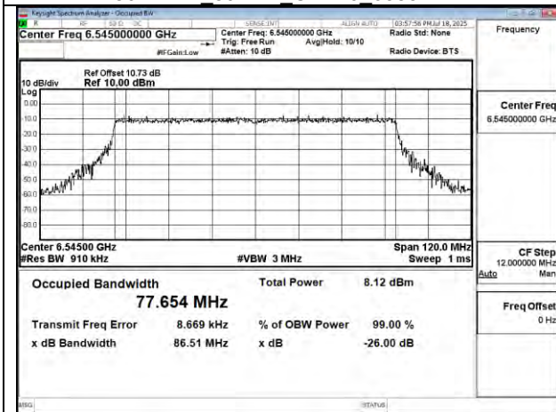
802.11be 80MHz Chain0 6545MHz
