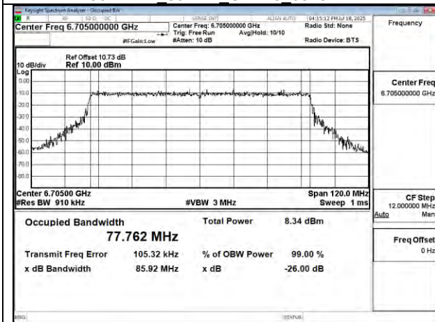
802.11be 80MHz Chain0 6705MHz
