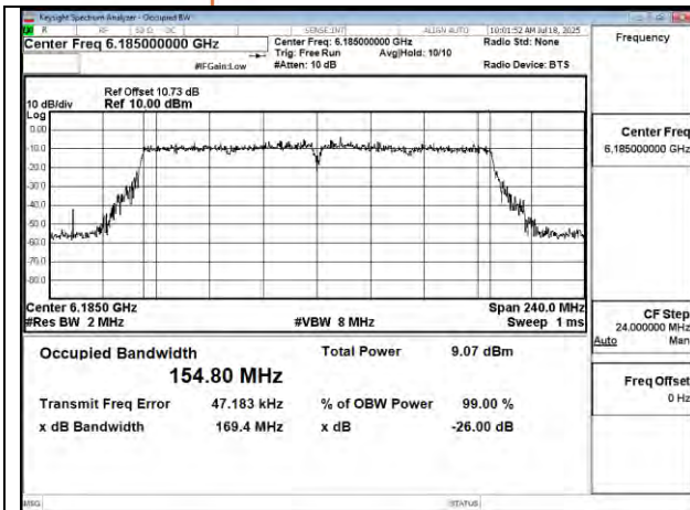
802.11ac 160MHz Chain1 6185MHz
