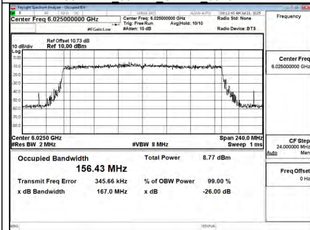
802.11be 160MHz Chain0 6025MHz
