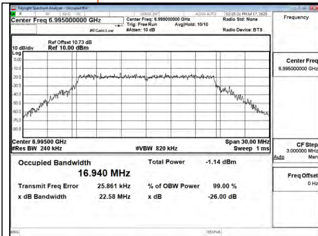
802.11a 20MHz Chain1 6995MHz
