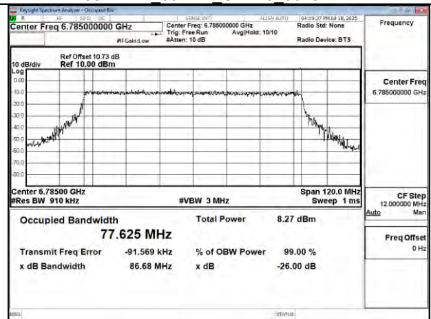
802.11be 80MHz Chain0 6785MHz
