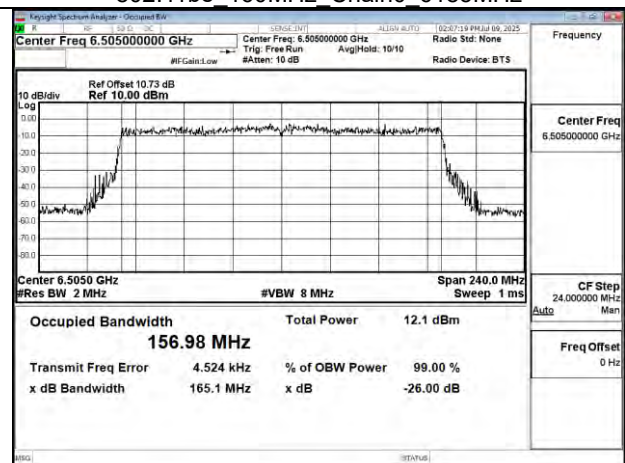
802.11be 160MHz Chain0 6505MHz
