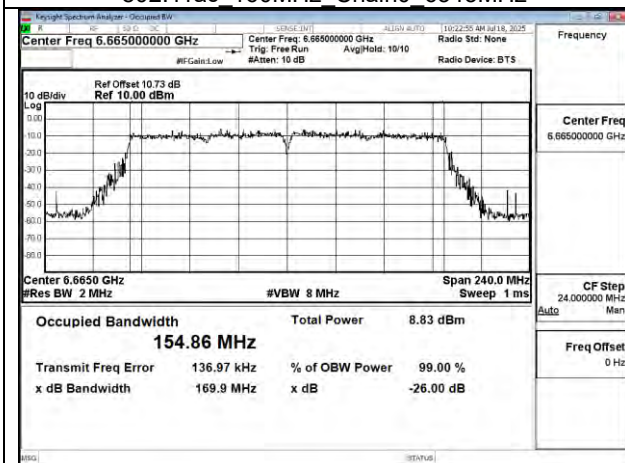
802.11ac 160MHz Chain0 6665MHz
