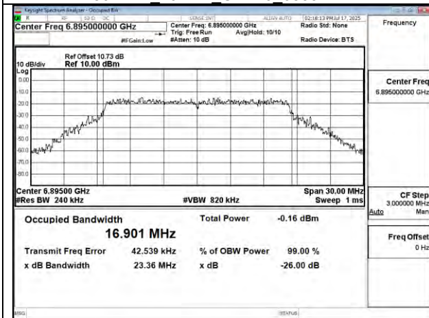
802.11a 20MHz Chain0 6895MHz
