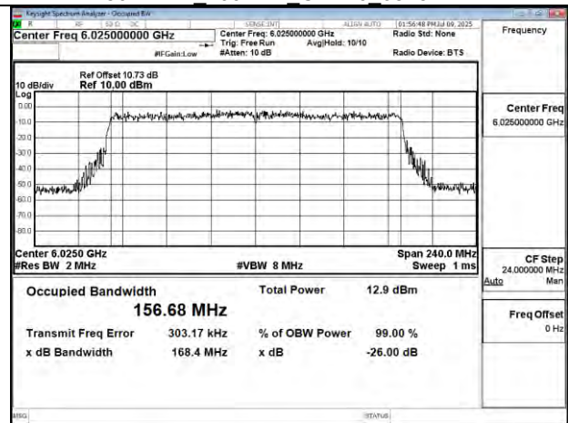
802.11be 160MHz Chain1 6025MHz
