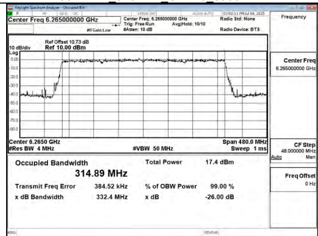
802.11be 320MHz Chain1 6265MHz
