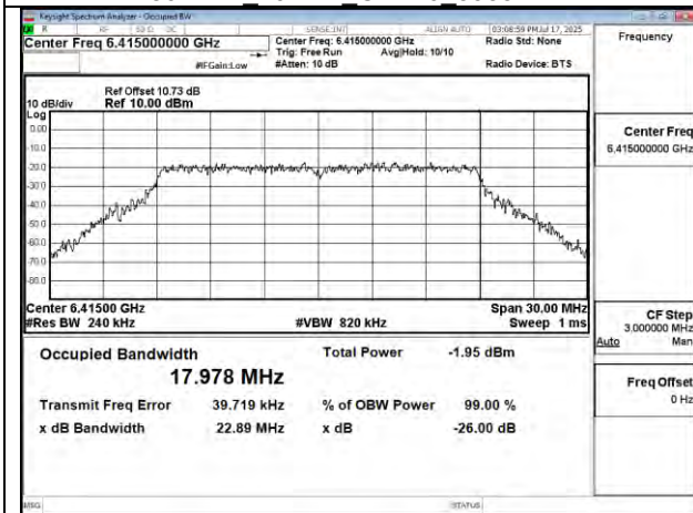
802.11n 20MHz Chain0 6415MHz
