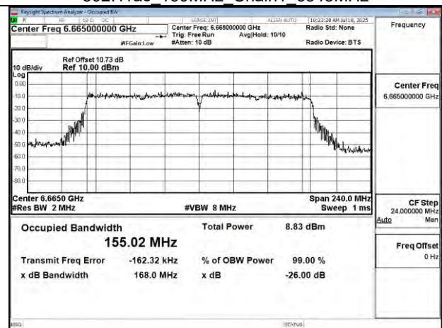
802.11ac 160MHz Chain1 6665MHz
