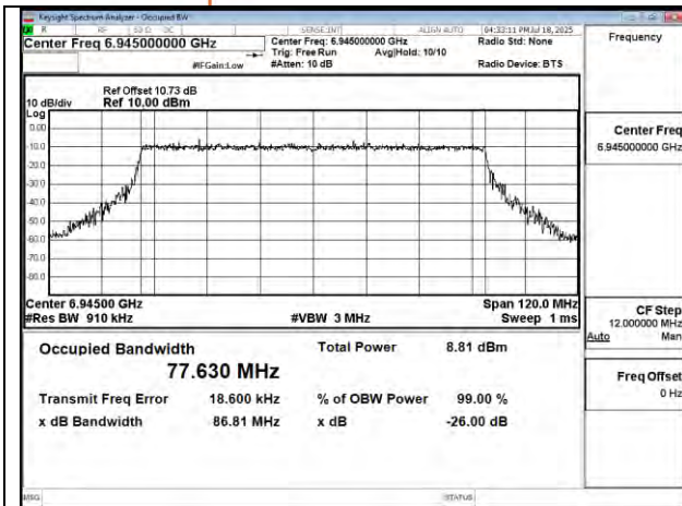
802.11be 80MHz Chain1 6945MHz
