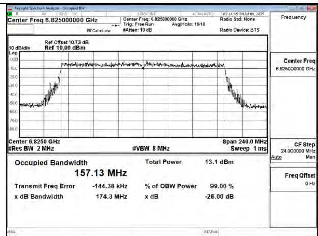
802.11be 160MHz Chain0 6825MHz
