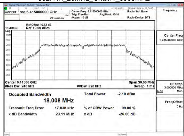
802.11n 20MHz Chain1 6415MHz
