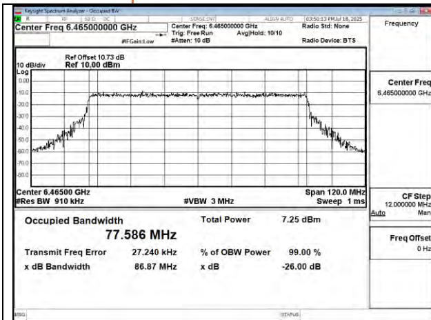
802.11be 80MHz Chain1 6465MHz
