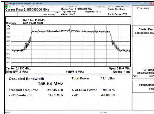
802.11be 160MHz Chain1 6185MHz
