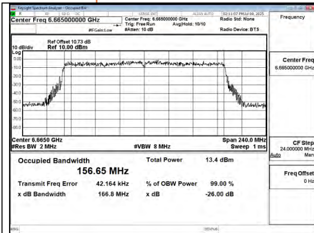
802.11be 160MHz Chain0 6665MHz
