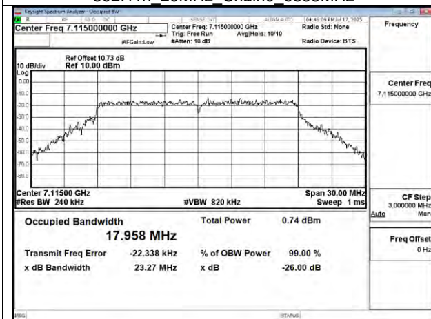
802.11n 20MHz Chain0 7115MHz
