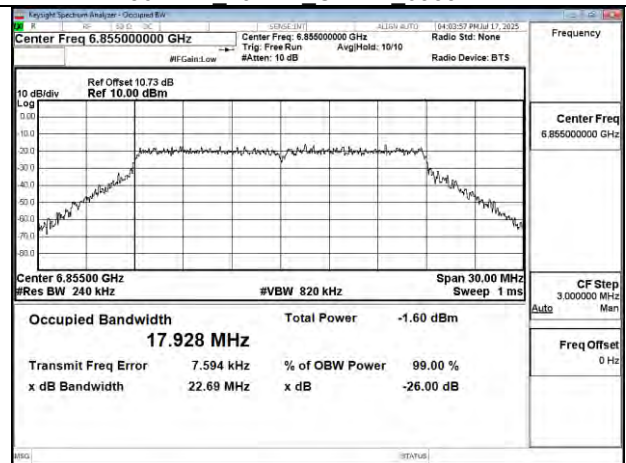
802.11n 20MHz Chain1 6855MHz
