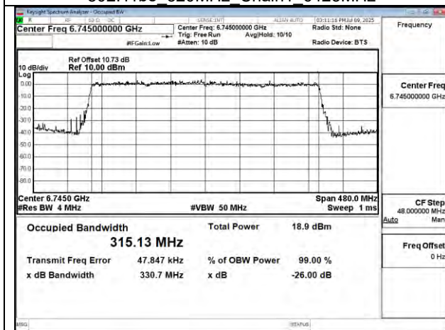
802.11be 320MHz Chain1 6745MHz
