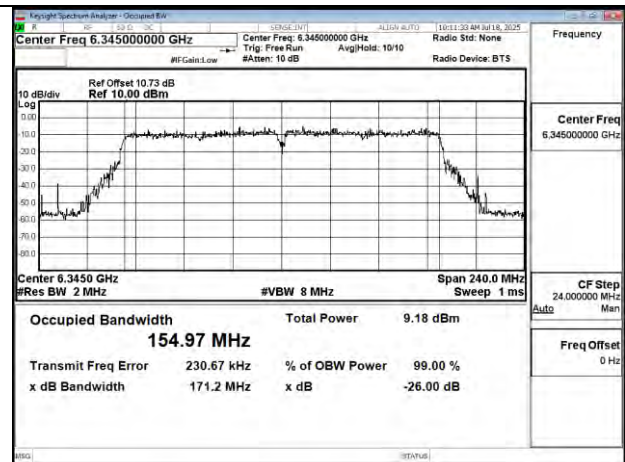
802.11ac 160MHz Chain1 6345MHz
