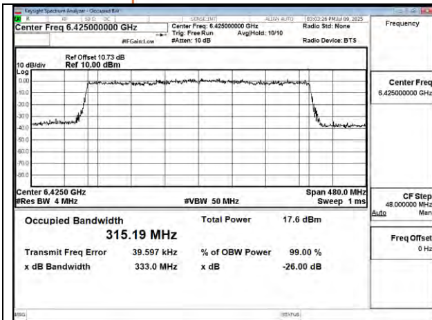
802.11be 320MHz Chain0 6425MHz
