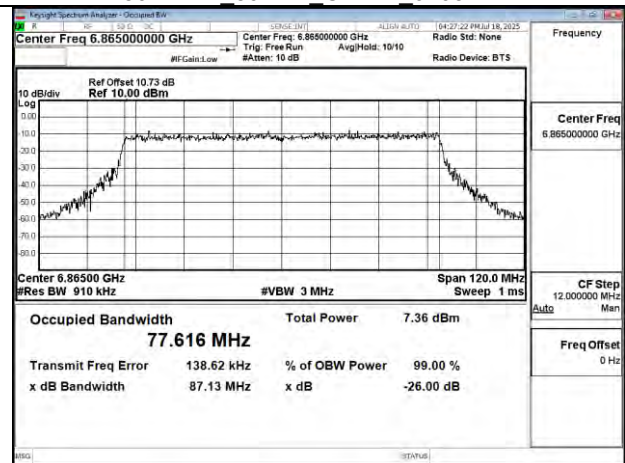
802.11be 80MHz Chain1 6865MHz
