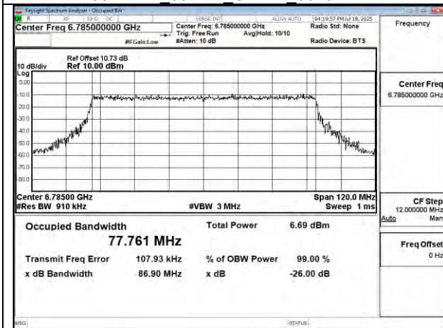
802.11be 80MHz Chain1 6785MHz
