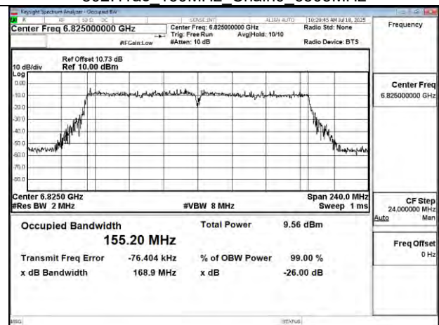
802.11ac 160MHz Chain0 6825MHz
