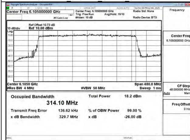
802.11be 320MHz Chain1 6105MHz
