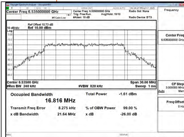
802.11a 20MHz Chain0 6535MHz
