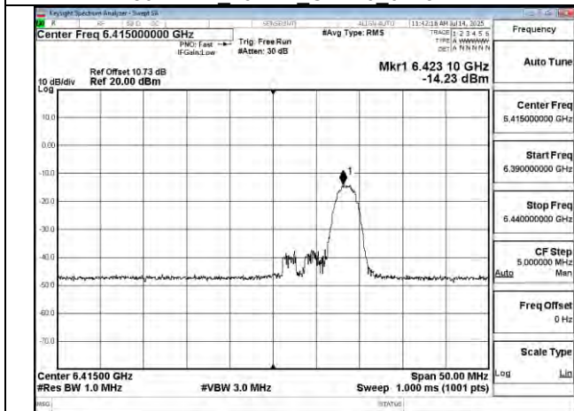
802.11be 20MHz Chain0 6415MHz RU26 8
