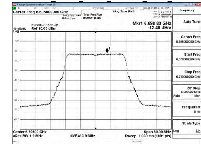
802.11be 20MHz Chain0 6695MHz
