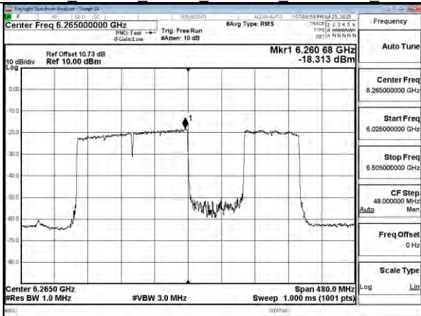
802.11be 320MHz Chain1 6265MHz 3x996 MRU3
