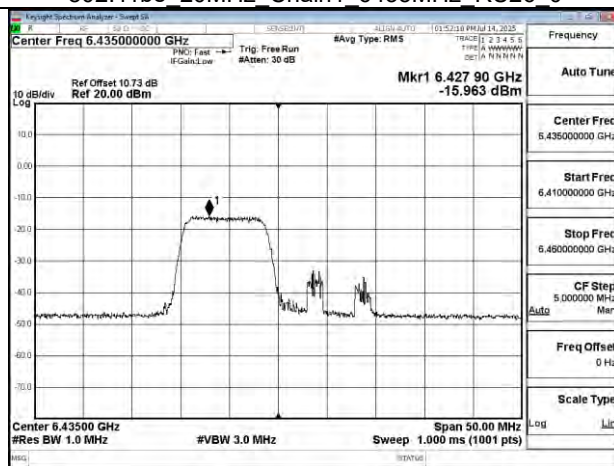
802.11be 20MHz Chain1 6435MHz RU106 53
