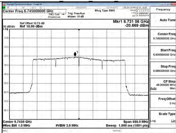
802.11be 320MHz Chain0 6745MHz
