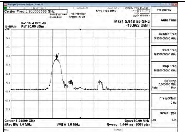
802.11be 20MHz Chain0 5955MHz RU26 0
