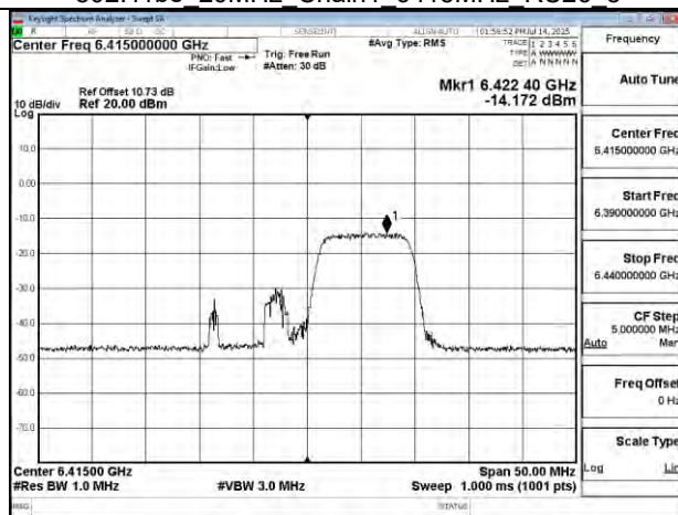
802.11be 20MHz Chain1 6415MHz RU106 54
