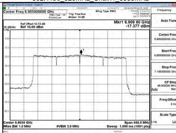
802.11be 320MHz Chain1 6905MHz
