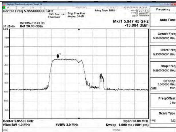
802.11be 20MHz Chain1 5955MHz 106+26 MRU1
