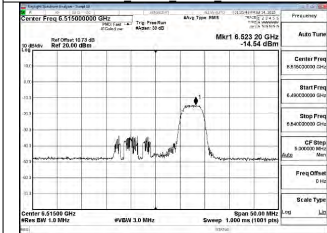
802.11be 20MHz Chain0 6515MHz RU52 40
