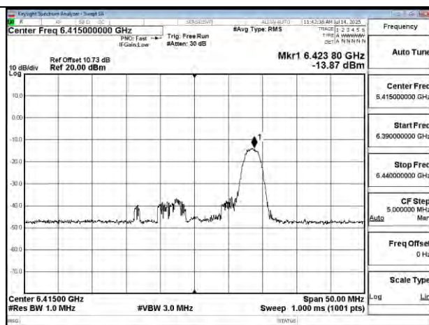
802.11be 20MHz Chain1 6415MHz RU26 8
