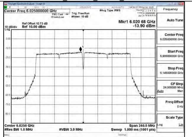
802.11ac 160MHz Chain1 6025MHz
