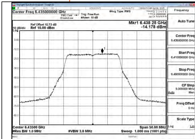
802.11n 20MHz Chain1 6435MHz
