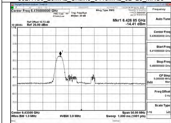
802.11be 20MHz Chain0 6435MHz RU26_0
