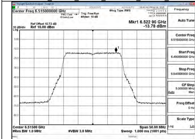
802.11be 20MHz Chain0 6515MHz
