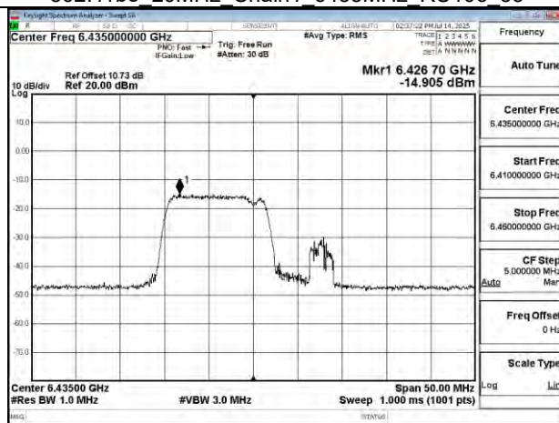
802.11be 20MHz Chain1 6435MHz 106+26 MRU1
