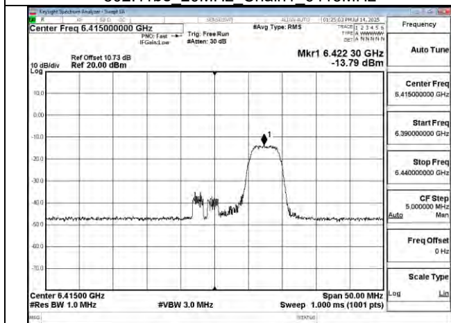
802.11be 20MHz Chain1 6415MHz RU52 40
