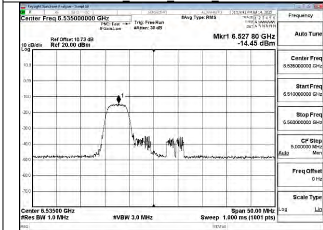
802.11be 20MHz Chain0 6535MHz RU52 37
