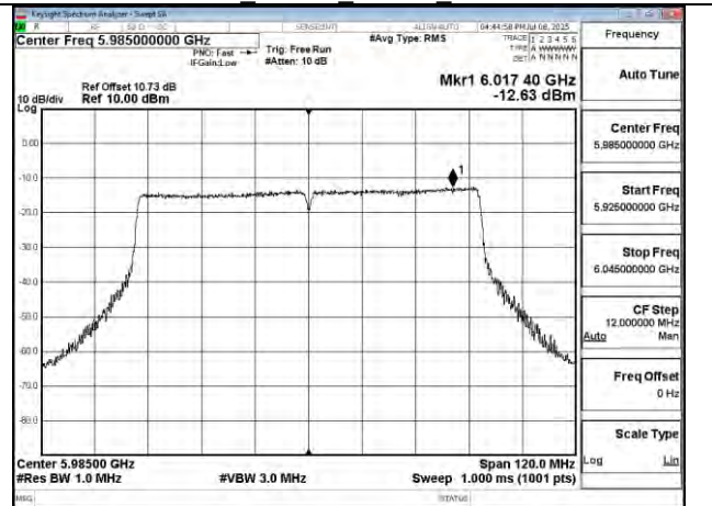
802.11ac 80MHz Chain1 5985MHz
