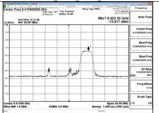
802.11be 20MHz Chain0 6415MHz RU52 40
