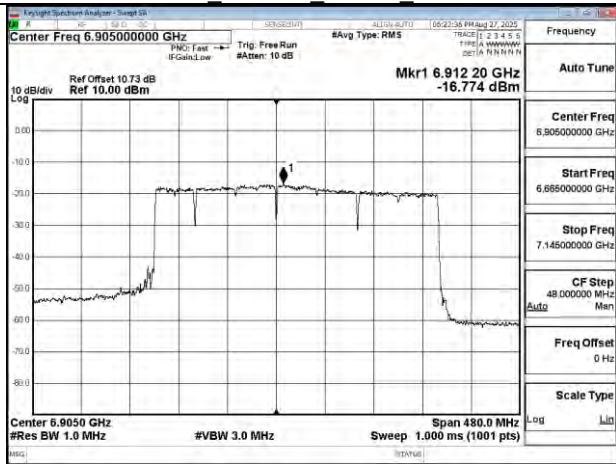
802.11be 320MHz Chain0 6905MHz 3x996+484 MRU1
