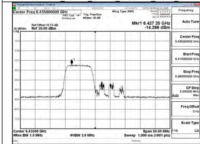
802.11be 20MHz Chain0 6435MHz RU106_53
