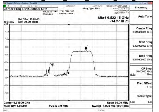
802.11be 20MHz Chain0 6515MHz RU106 54
