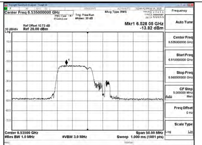
802.11be 20MHz Chain0 6535MHz 106+26 MRU1
