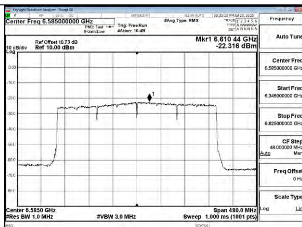
802.11be 320MHz Chain1 6585MHz
