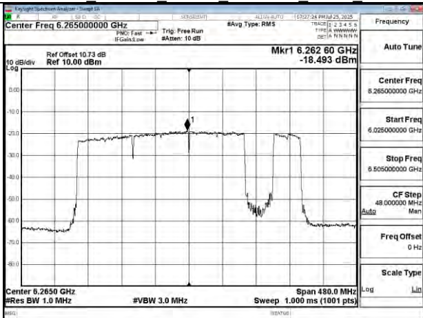
802.11be 320MHz Chain0 6265MHz 3x996+484 MRU7
