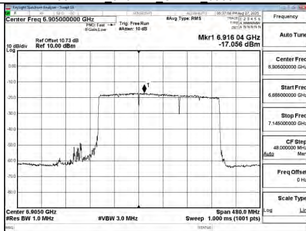
802.11be 320MHz Chain1 6905MHz 3x996 MRU1
