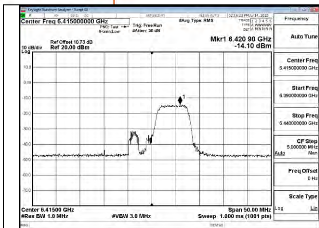
802.11be 20MHz Chain0 6415MHz 52+26 MRU3
