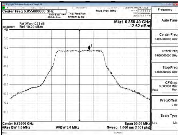
802.11a 20MHz Chain0 6855MHz
