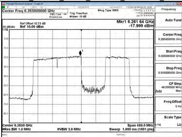
802.11be 320MHz Chain0 6265MHz 3x996 MRU3
