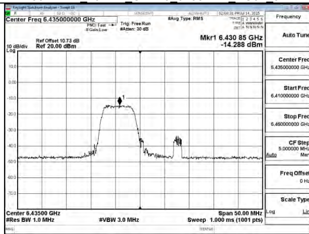
802.11be 20MHz Chain0 6435MHz 52+26 MRU1
