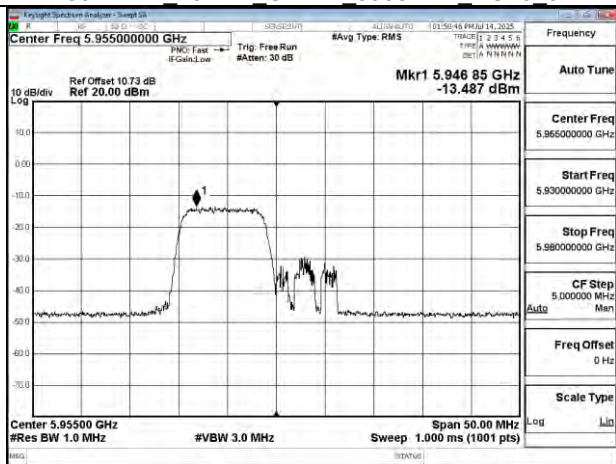
802.11be 20MHz Chain1 5955MHz RU106_53
