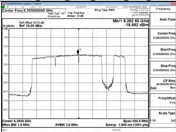
802.11be 320MHz Chain1 6265MHz 3x996+484 MRU7
