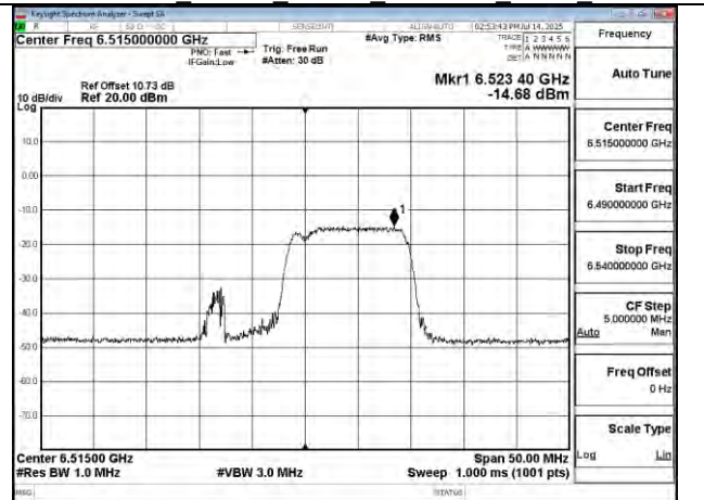
802.11be 20MHz Chain1 6515MHz 106+26 MRU2
