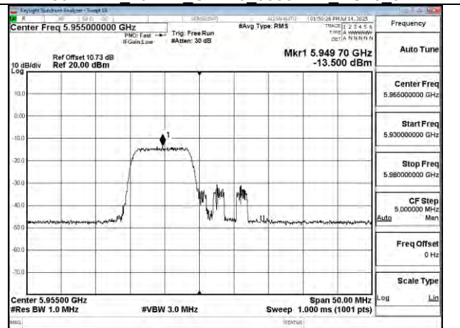
802.11be 20MHz Chain0 5955MHz RU106 53
