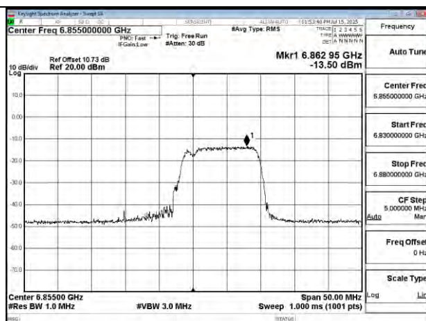
802.11be 20MHz Chain0 6855MHz 106+26 MRU2
