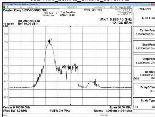
802.11be 20MHz Chain0 6895MHz RU26 0
