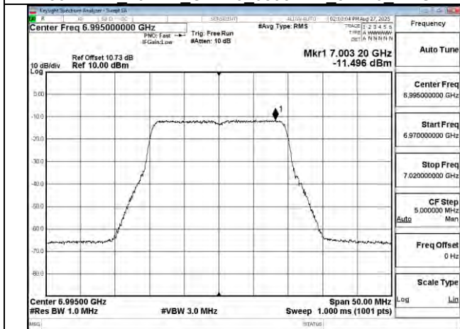
802.11be 20MHz Chain0 6995MHz
