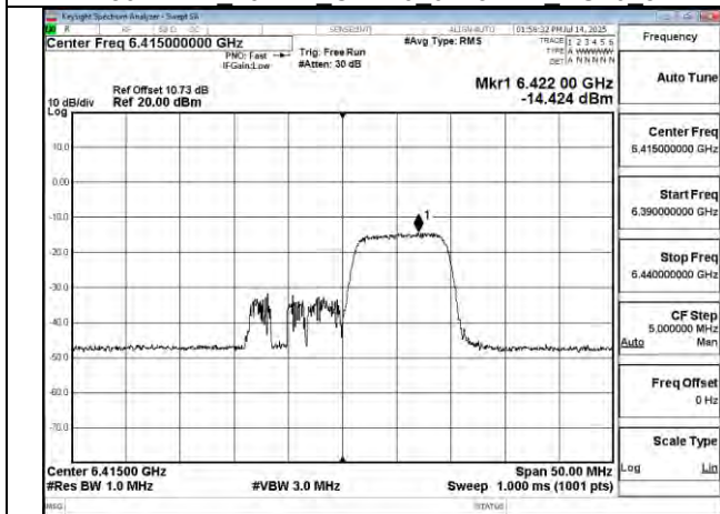
802.11be 20MHz Chain0 6415MHz RU106 54
