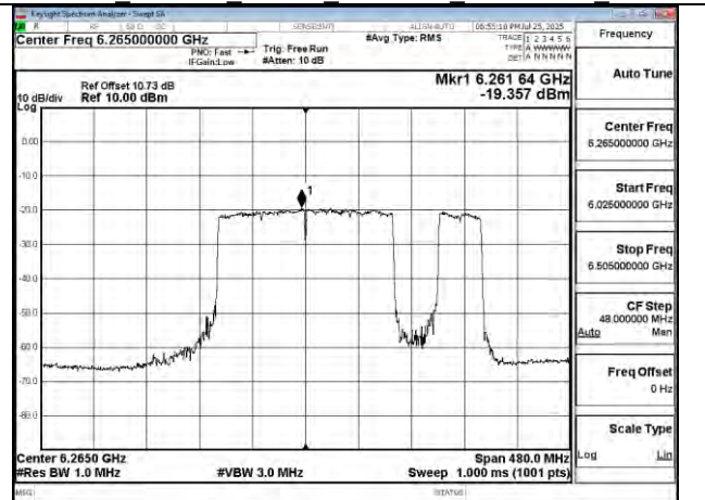
802.11be 320MHz Chain0 6265MHz 2x996+484 MRU11
