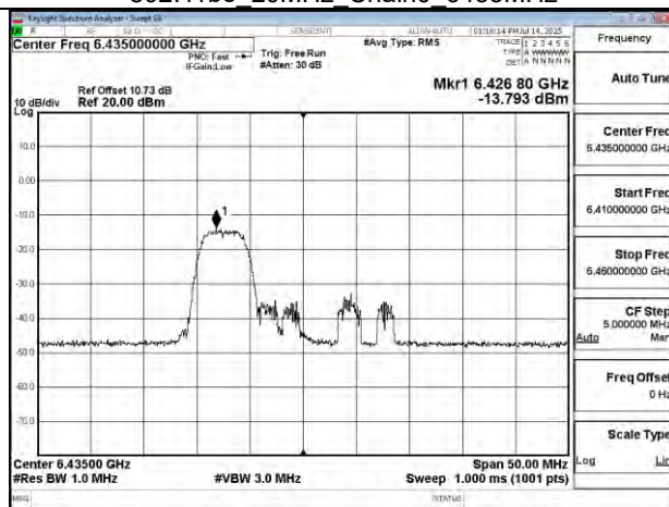
802.11be 20MHz Chain0 6435MHz RU52_37
