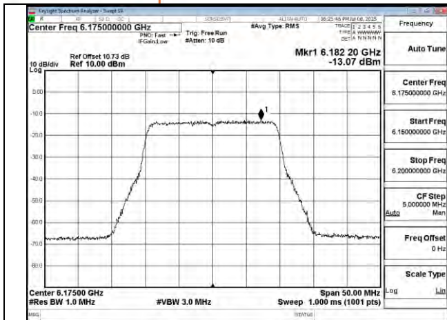
802.11be 20MHz Chain0 6175MHz
