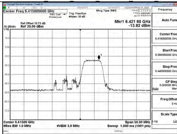
802.11be 20MHz Chain1 6415MHz 52+26 MRU3
