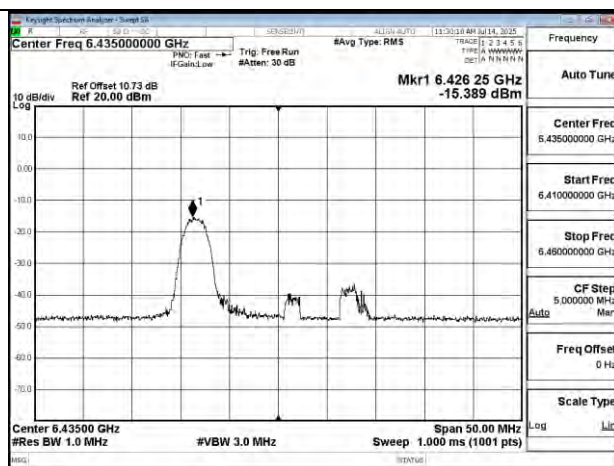
802.11be 20MHz Chain1 6435MHz RU26 0
