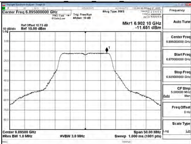
802.11a 20MHz Chain0 6895MHz
