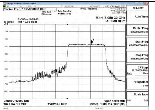
802.11be 80MHz Chain1 7025MHz RU484 66
