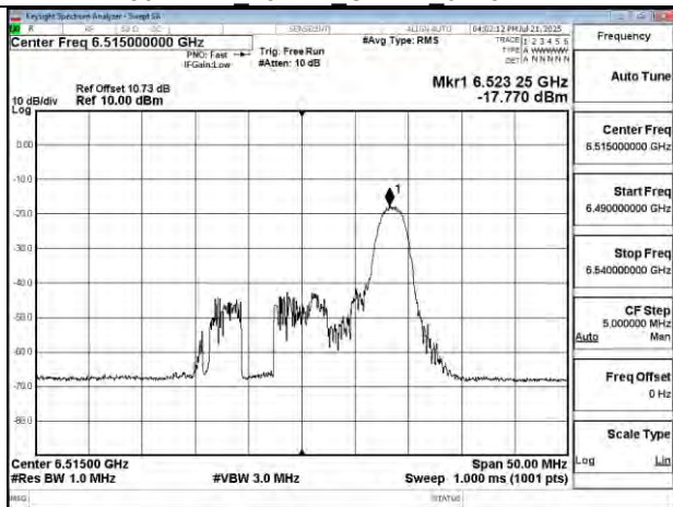
802.11be 20MHz Chain1 6515MHz RU26 8
