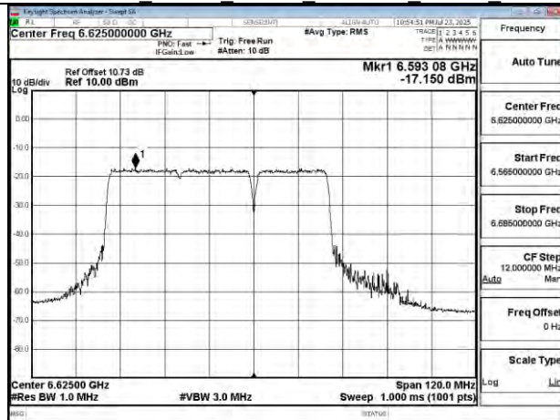
802.11be 80MHz Chain1 6625MHz 484+242 MRU4
