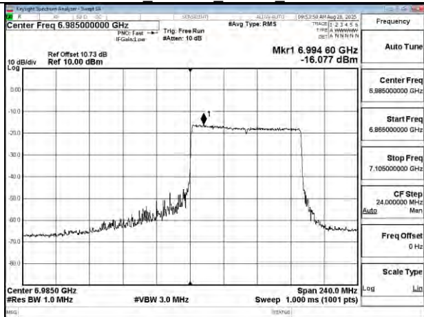
802.11be 160MHz Chain0 6985MHz RU996 S67
