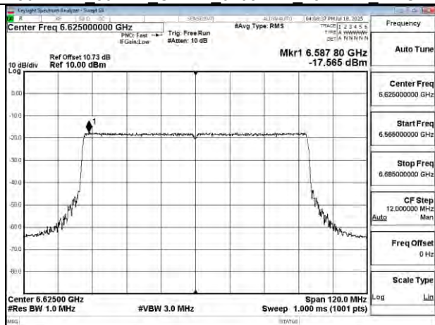
802.11be 80MHz Chain1 6625MHz
