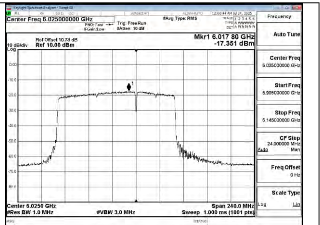
802.11be 160MHz Chain0 6025MHz 996+484 MRU4
