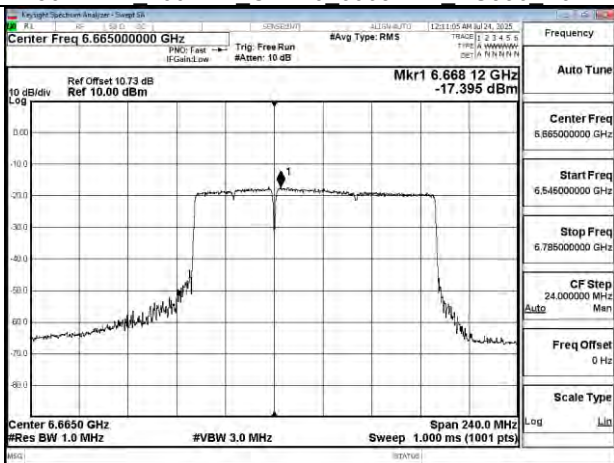
802.11be 160MHz Chain0 6665MHz 996+484 MRU1
