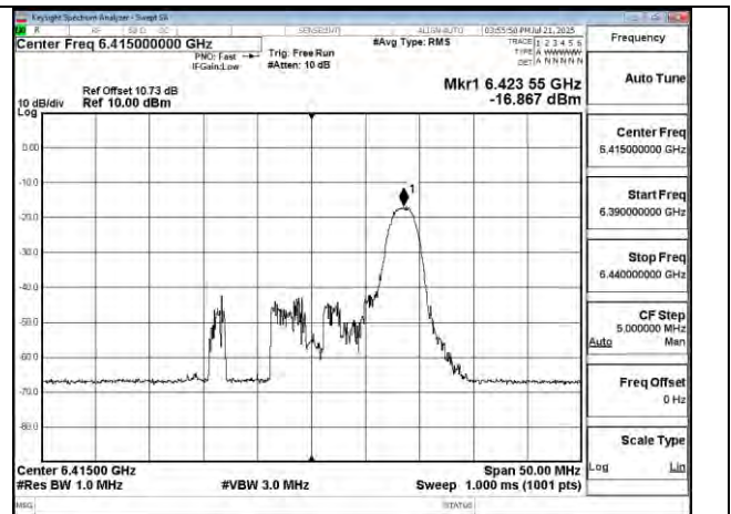
802.11be 20MHz Chain1 6415MHz RU26 8
