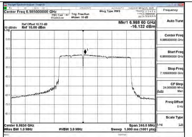
802.11be 160MHz Chain1 6985MHz 996+484 MRU1
