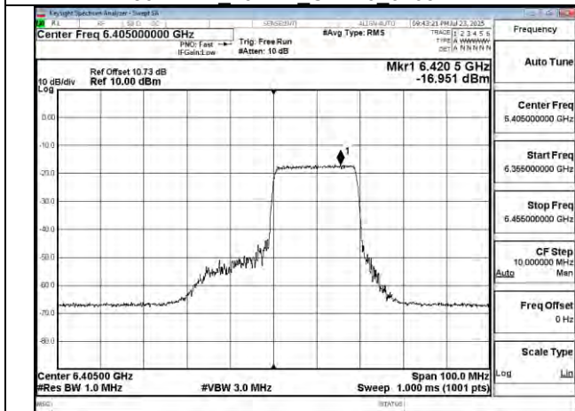
802.11be 40MHz Chain0 6405MHz RU242 62
