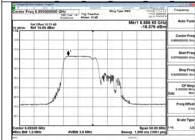
802.11be 20MHz Chain1 6895MHz 106+26 MRU1
