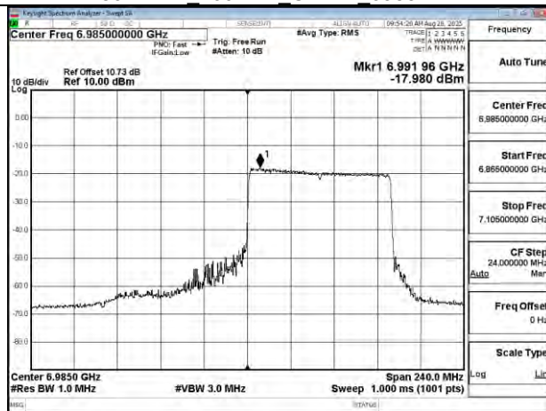
802.11be 160MHz Chain1 6985MHz RU996 S67
