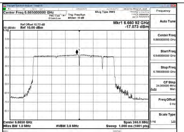
802.11be 160MHz Chain1 6665MHz 996+484+242 MRU8
