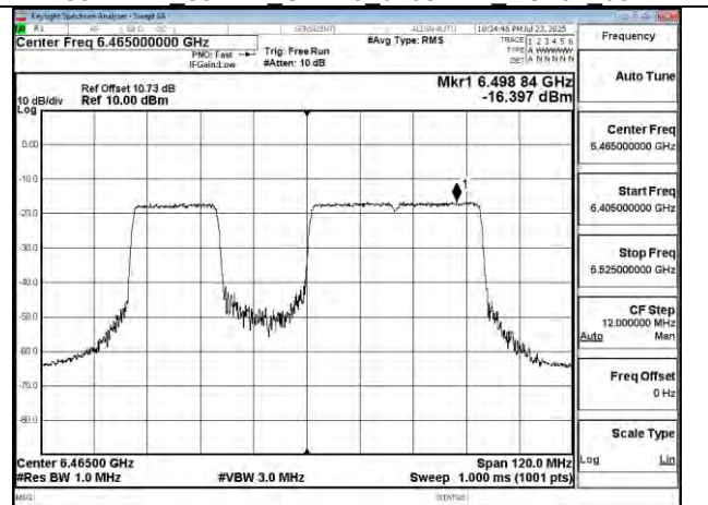
802.11be 80MHz Chain0 6465MHz 484+242 MRU2
