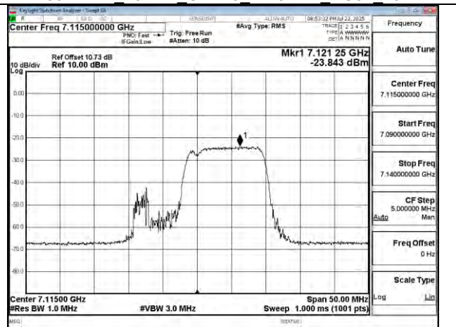
802.11be 20MHz Chain0 7115MHz 106+26 MRU2
