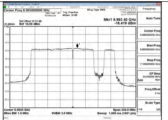
802.11be 160MHz Chain0 6985MHz 996+484+242 MRU7
