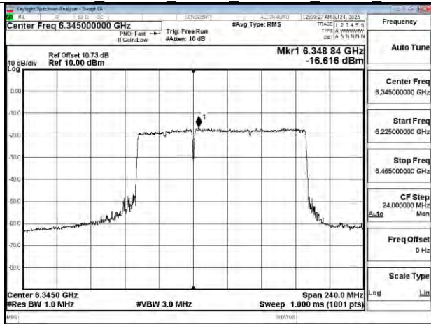
802.11be 160MHz Chain1 6345MHz 996+484 MRU1
