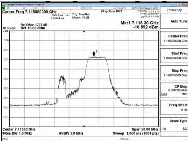
802.11be 20MHz Chain0 7115MHz 52+26 MRU3
