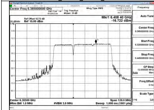
802.11be 80MHz Chain1 6385MHz 484+242 MRU1
