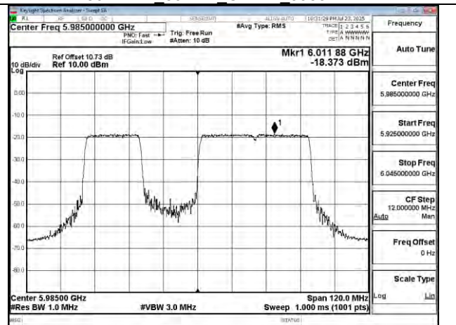
802.11be 80MHz Chain1 5985MHz 484+242 MRU2
