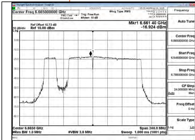
802.11be 160MHz Chain1 6665MHz 996+484+242 MRU2
