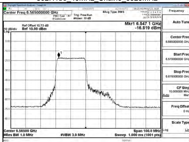
802.11be 40MHz Chain0 6565MHz RU242 61
