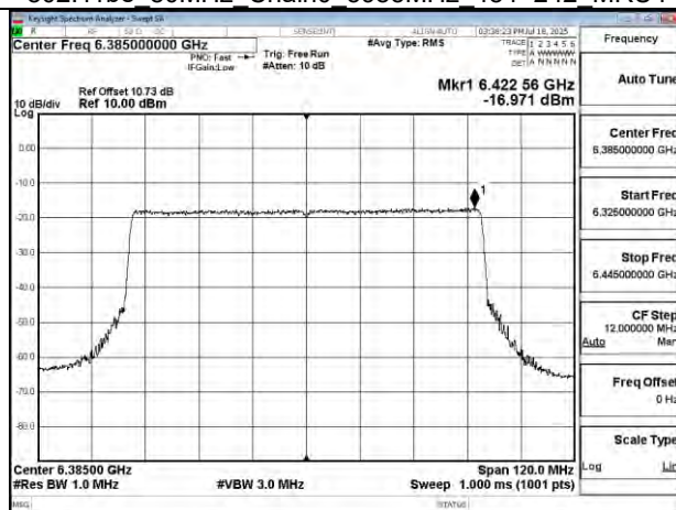
802.11be 80MHz Chain0 6385MHz
