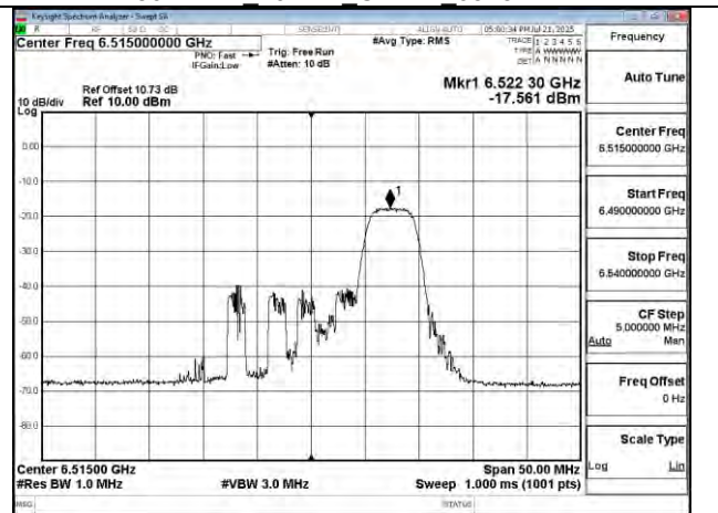
802.11be 20MHz Chain1 6515MHz RU52 40
