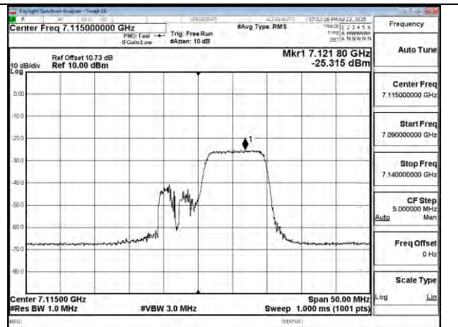
802.11be 20MHz Chain1 7115MHz RU106 54
