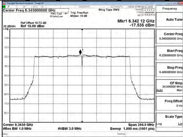
802.11be 160MHz Chain0 6345MHz
