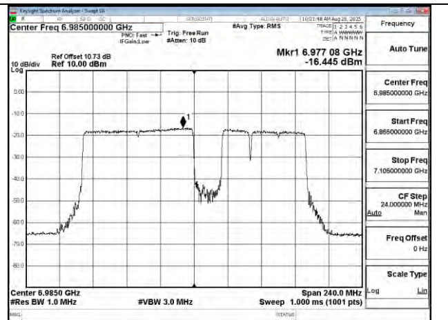
802.11be 160MHz Chain1 6985MHz 996+484+242 MRU5
