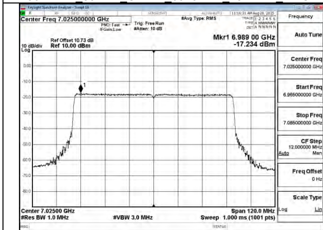
802.11be 80MHz Chain1 7025MHz
