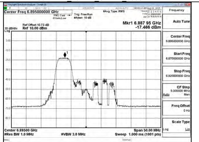
802.11be 20MHz Chain1 6895MHz RU52_37
