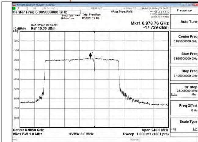
802.11be 160MHz Chain1 6985MHz 996+484 MRU4
