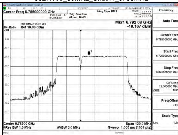
802.11be 80MHz Chain1 6785MHz 484+242 MRU1
