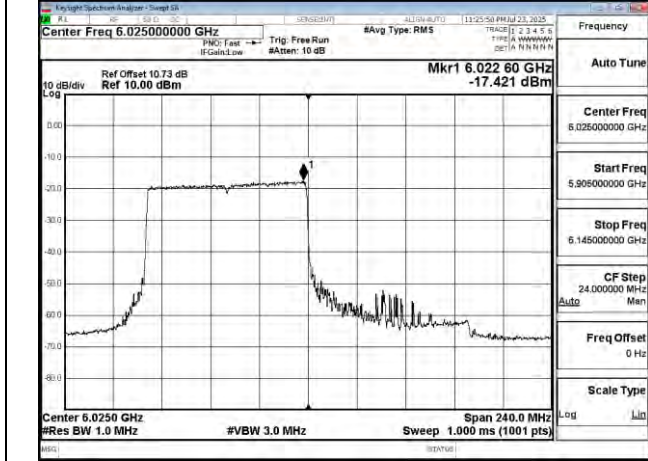
802.11be 160MHz Chain1 6025MHz RU996 67
