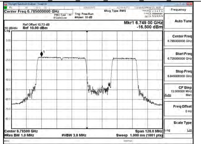
802.11be 80MHz Chain0 6785MHz 484+242 MRU3
