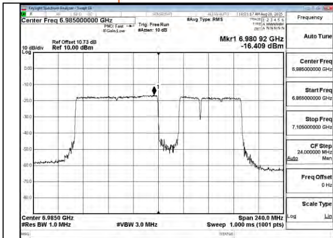
802.11be 160MHz Chain0 6985MHz 996+484+242 MRU5
