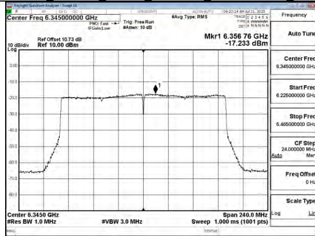
802.11be 160MHz Chain1 6345MHz
