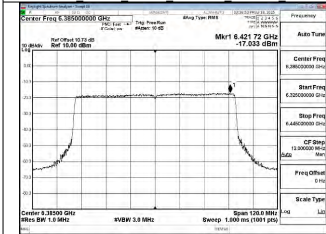
802.11be 80MHz Chain1 6385MHz
