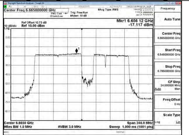
802.11be 160MHz Chain1 6665MHz 996+484+242 MRU5
