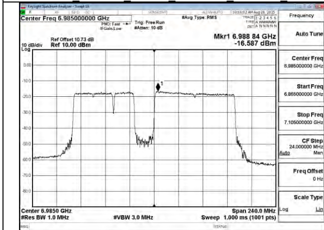
802.11be 160MHz Chain0 6985MHz 996+484+242 MRU4
