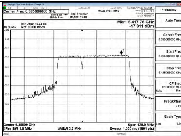
802.11be 80MHz Chain0 6385MHz 484+242 MRU1
