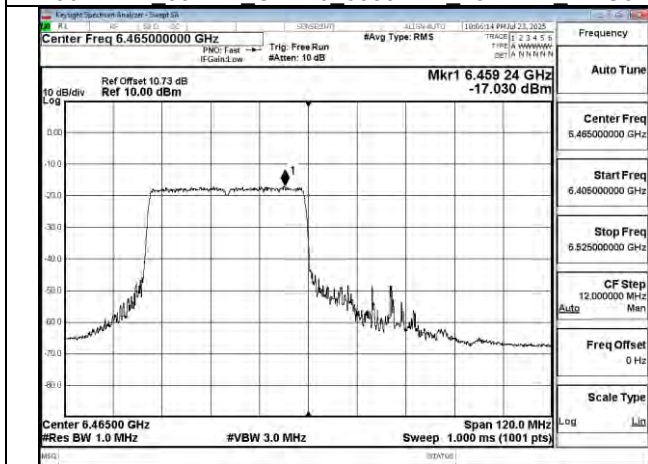
802.11be 80MHz Chain0 6465MHz RU484 65
