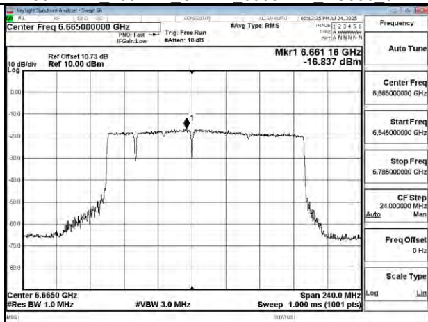
802.11be 160MHz Chain1 6665MHz 996+484+242 MRU1
