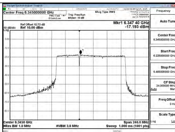
802.11be 160MHz Chain0 6345MHz 996+484 MRU1
