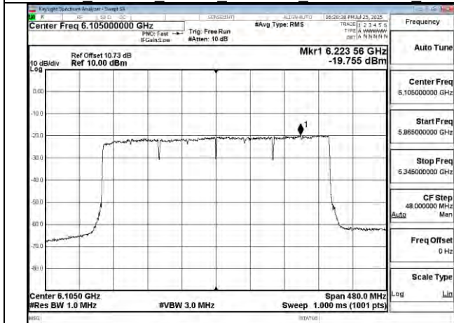
802.11be 320MHz Chain0 6105MHz
