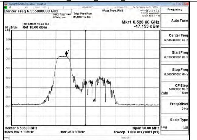
802.11be 20MHz Chain1 6535MHz RU52_37
