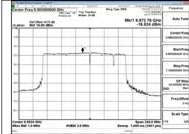
802.11be 160MHz Chain0 6985MHz 996+484+242 MRU8
