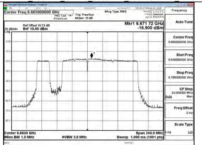
802.11be 160MHz Chain0 6665MHz 996+484+242 MRU2
