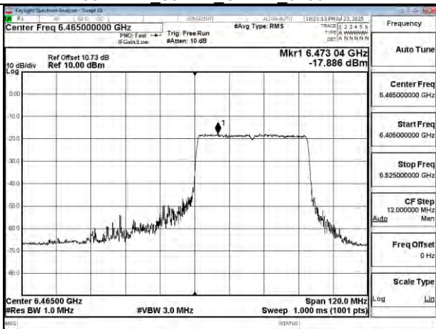
802.11be 80MHz Chain1 6465MHz RU484 66
