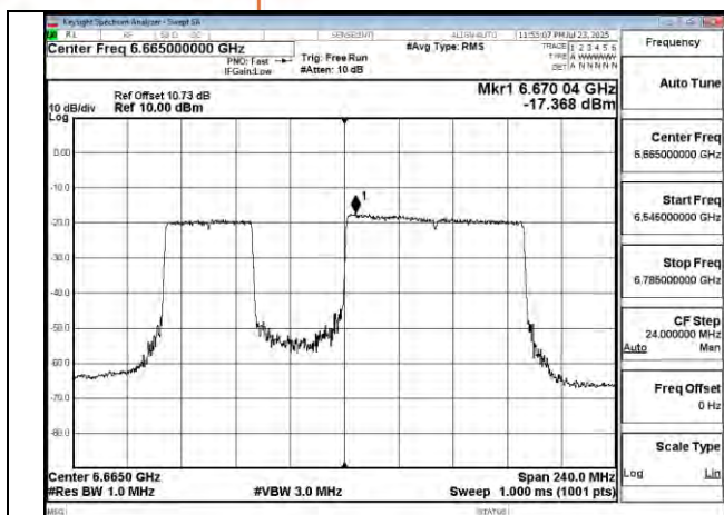
802.11be 160MHz Chain0 6665MHz 996+484 MRU2
