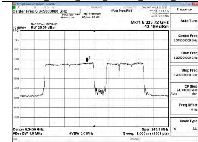
802.11be 160MHz Chain1 6345MHz 996+484+242 MRU5
