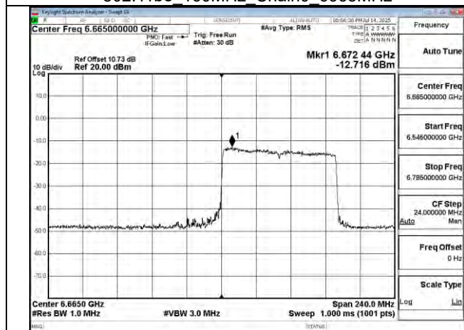
802.11be 160MHz Chain0 6665MHz RU996 S67
