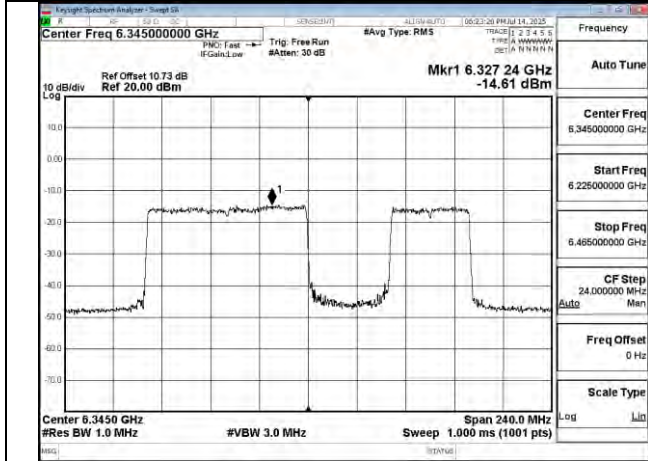
802.11be 160MHz Chain0 6345MHz 996+484 MRU3
