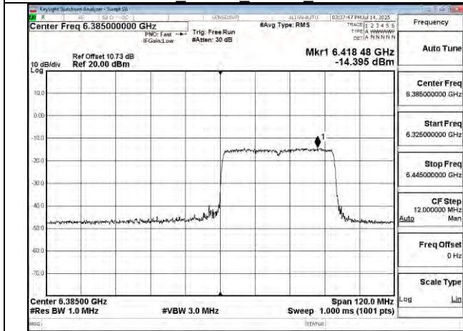
802.11be 80MHz Chain0 6385MHz RU484 66
