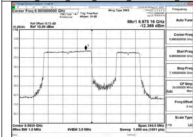
802.11be 160MHz Chain1 6985MHz 996+484 MRU3
