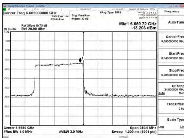
802.11be 160MHz Chain0 6665MHz RU996 67
