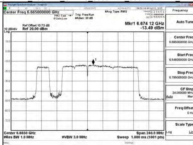
802.11be 160MHz Chain0 6665MHz 996+484+242 MRU2
