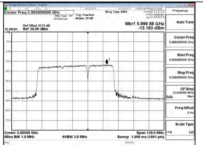
802.11be 80MHz Chain0 5985MHz 484+242 MRU4
