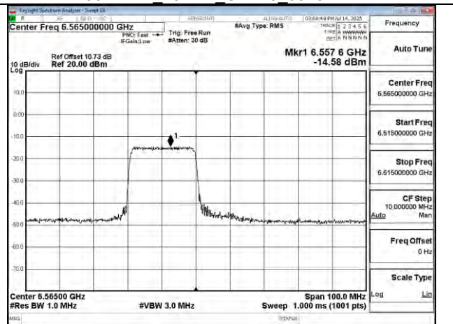
802.11be 40MHz Chain0 6565MHz RU242 61
