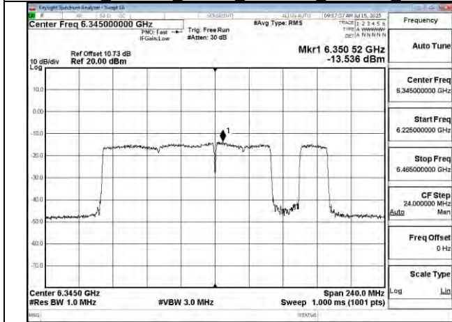
802.11be 160MHz Chain0 6345MHz 996+484+242 MRU7
