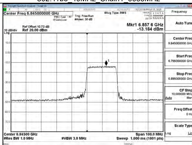
802.11be 40MHz Chain1 6845MHz RU242 62
