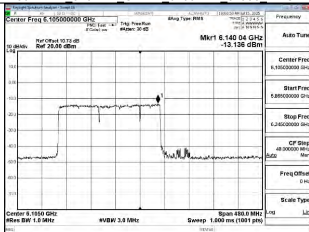
802.11be 320MHz Chain1 6105MHz 2x996+484 MRU6
