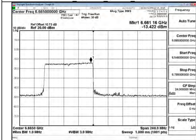
802.11be 160MHz Chain1 6665MHz RU996 67
