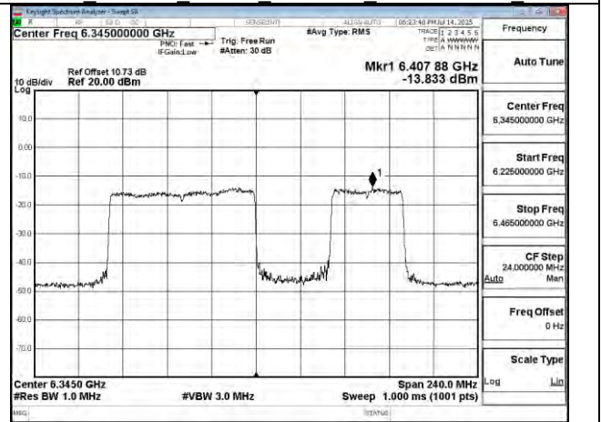
802.11be 160MHz Chain1 6345MHz 996+484 MRU3
