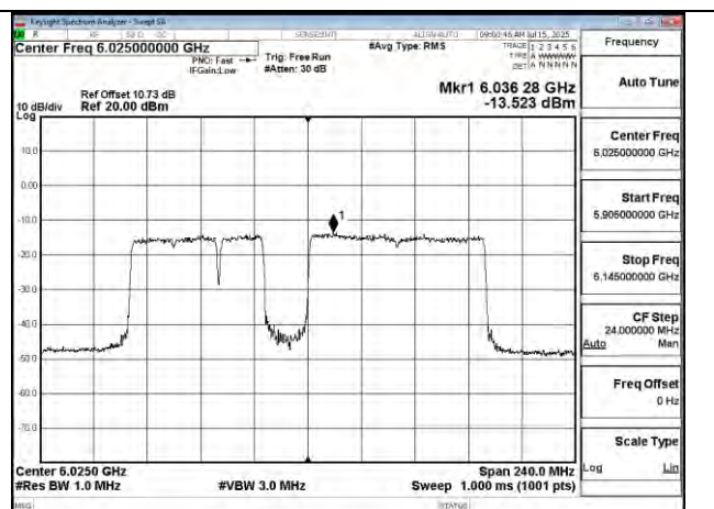
802.11be 160MHz Chain1 6025MHz 996+484+242 MRU4
