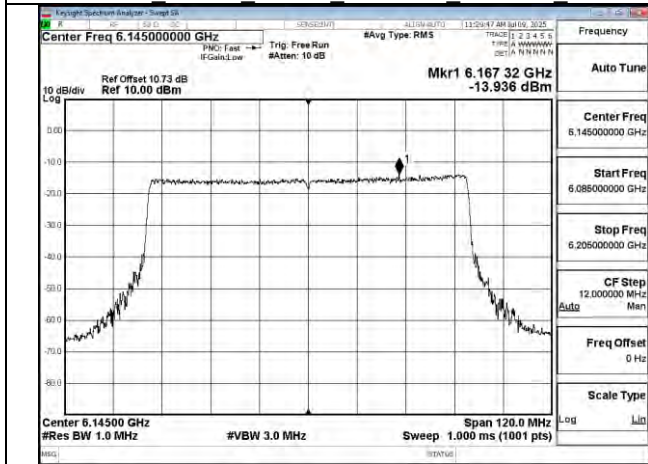
802.11be 80MHz Chain0 6145MHz
