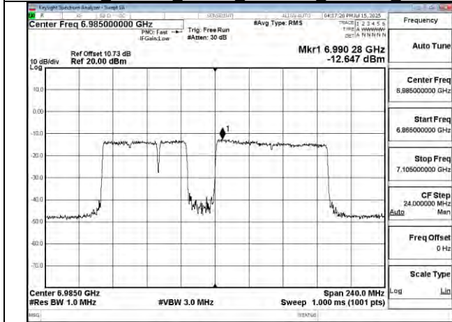
802.11be 160MHz Chain0 6985MHz 996+484+242 MRU4
