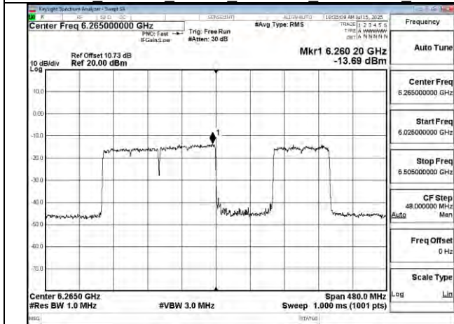
802.11be 320MHz Chain1 6265MHz 3x996 MRU3
