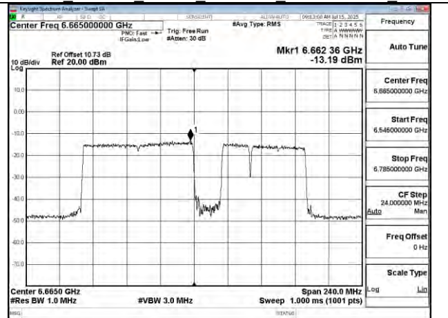
802.11be 160MHz Chain1 6665MHz 996+484+242 MRU5
