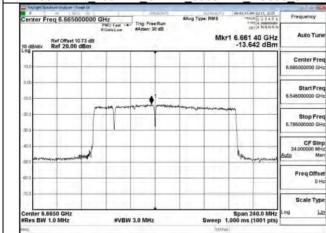
802.11be 160MHz Chain1 6665MHz 996+484+242 MRU1
