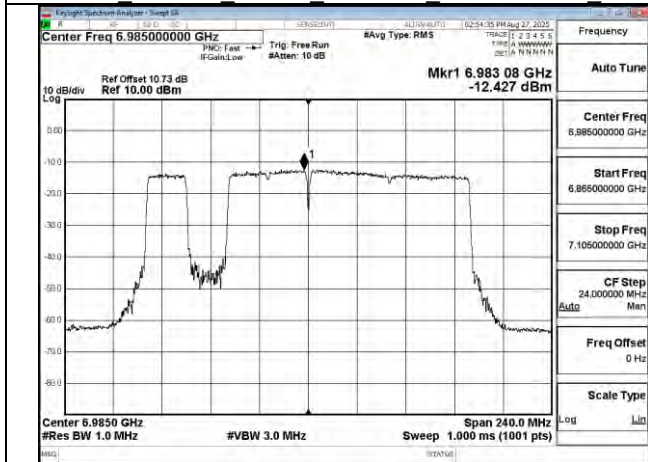
802.11be 160MHz Chain1 6985MHz 996+484+242 MRU2
