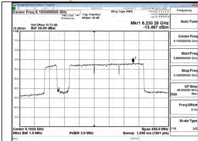
802.11be 320MHz Chain0 6105MHz 3x996+484 MRU2
