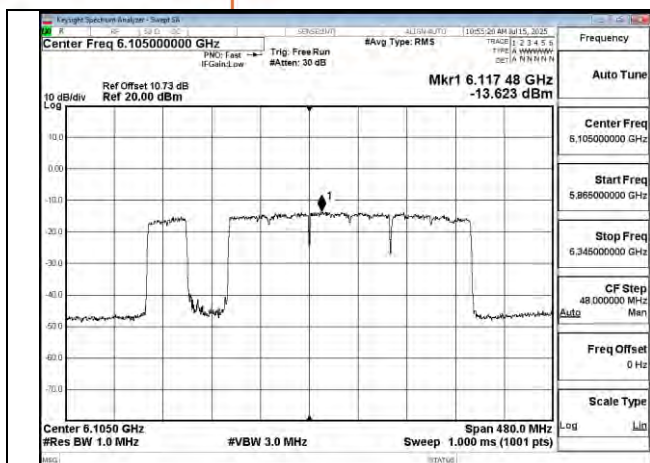
802.11be 320MHz Chain1 6105MHz 3x996+484 MRU2
