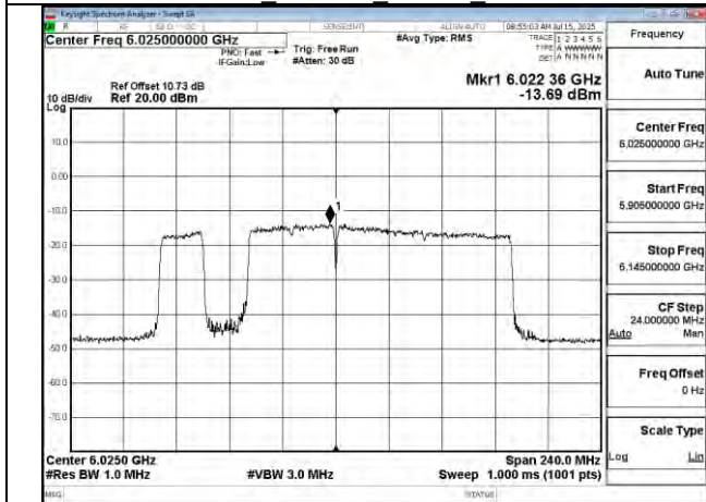
802.11be 160MHz Chain0 6025MHz 996+484+242 MRU2
