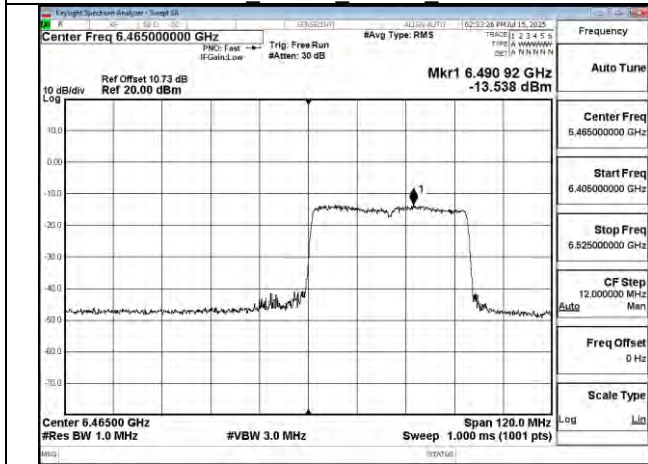
802.11be 80MHz Chain1 6465MHz RU484 66
