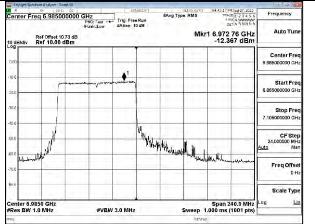
802.11be 160MHz Chain0 6985MHz RU996 67
