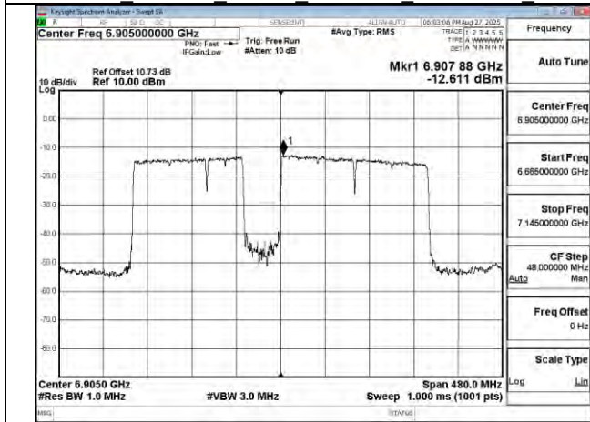
802.11be 320MHz Chain1 6905MHz 3x996+484 MRU4
