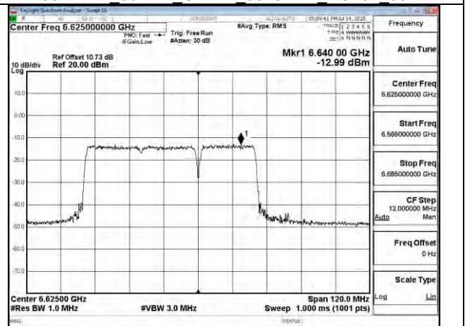
802.11be 80MHz Chain1 6625MHz 484+242 MRU4
