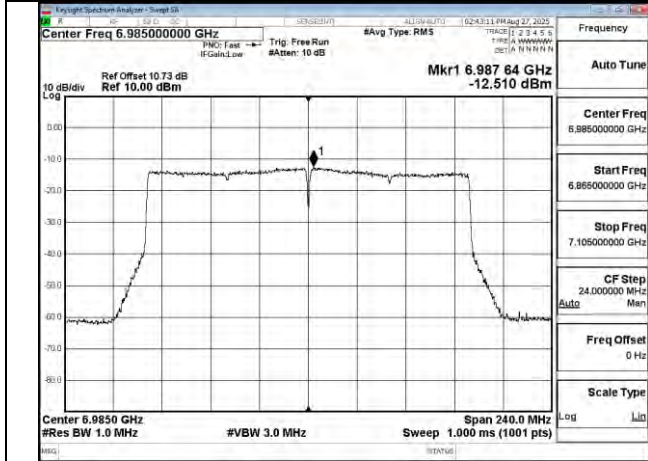
802.11be 160MHz Chain0 6985MHz
