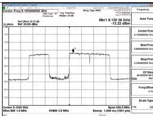
802.11be 320MHz Chain1 6105MHz 3x996 MRU2
