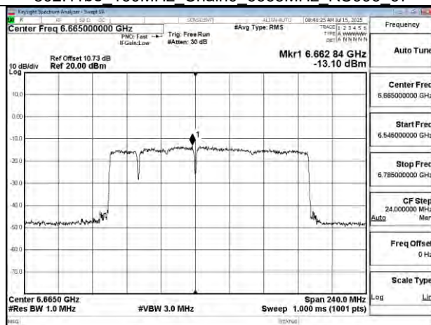
802.11be 160MHz Chain0 6665MHz 996+484+242 MRU1
