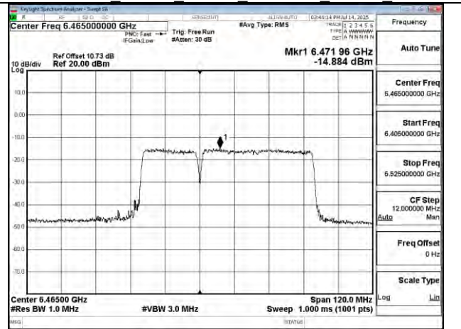
802.11be 80MHz Chain1 6465MHz 484+242 MRU1
