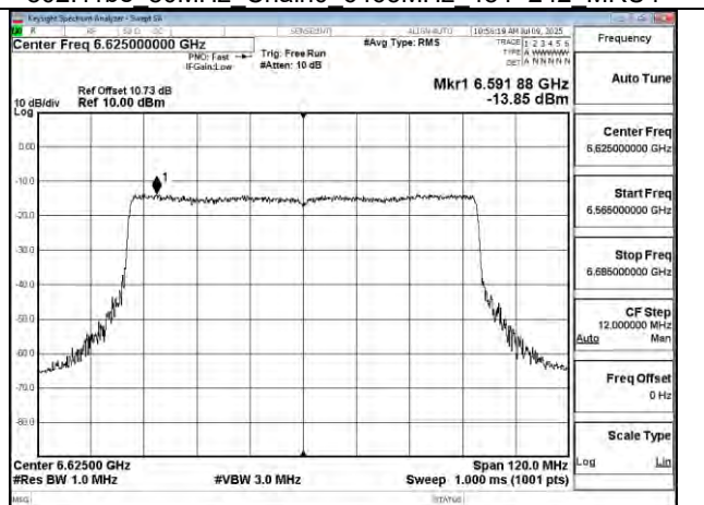
802.11be 80MHz Chain0 6625MHz
