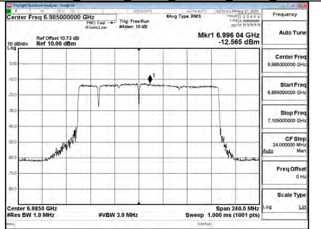
802.11be 160MHz Chain0 6985MHz 996+484+242 MRU1
