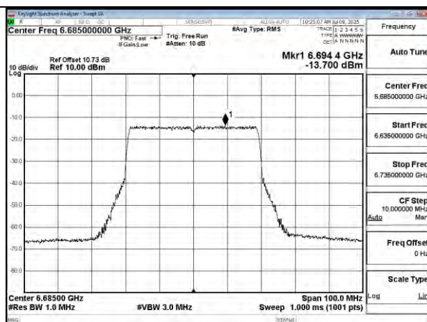
802.11be 40MHz Chain1 6685MHz
