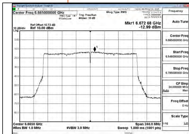
802.11be 160MHz Chain0 6665MHz
