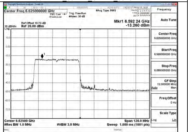
802.11be 80MHz Chain1 6625MHz RU484 65
