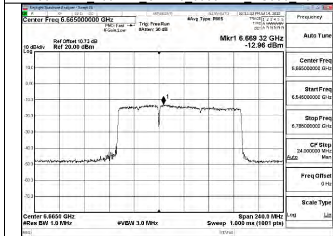
802.11be 160MHz Chain0 6665MHz 996+484 MRU1
