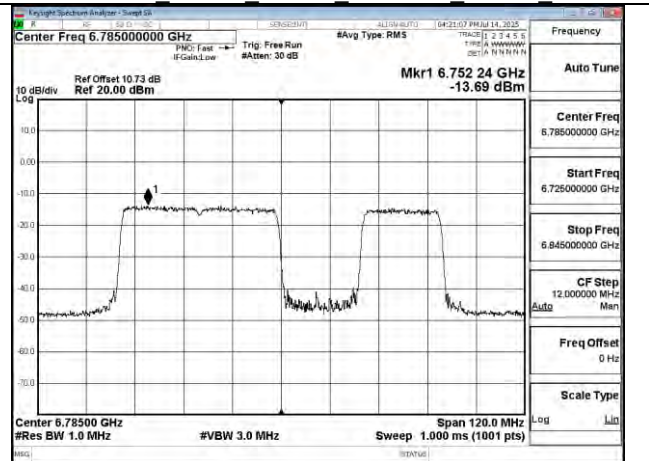
802.11be 80MHz Chain0 6785MHz 484+242 MRU3
