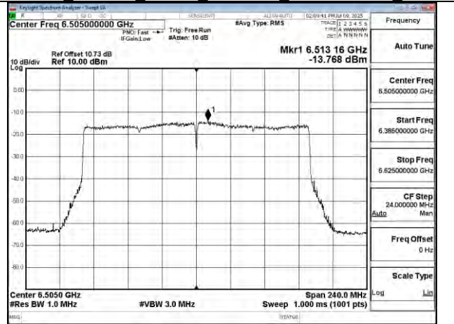
802.11be 160MHz Chain0 6505MHz
