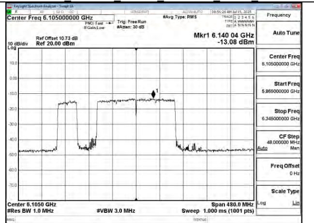
802.11be 320MHz Chain1 6105MHz 2x996+484 MRU2
