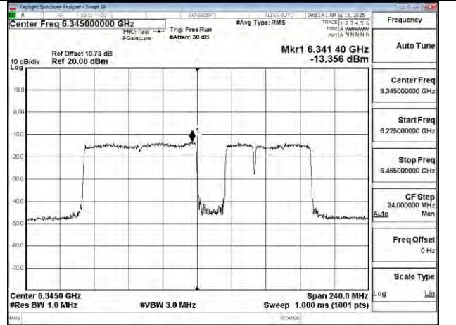
802.11be 160MHz Chain0 6345MHz 996+484+242 MRU5
