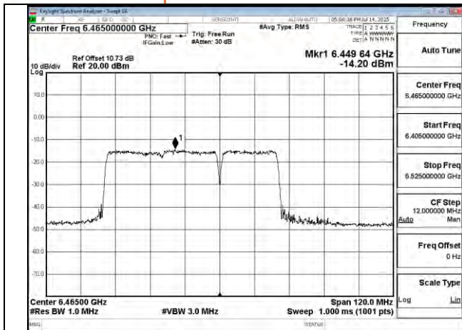
802.11be 80MHz Chain1 6465MHz 484+242 MRU4
