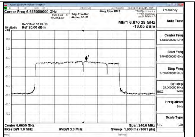
802.11be 160MHz Chain1 6665MHz 996+484+242 MRU8
