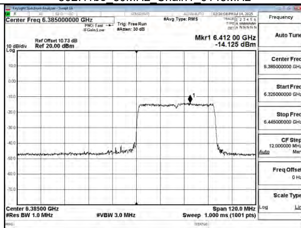
802.11be 80MHz Chain1 6385MHz RU484 66
