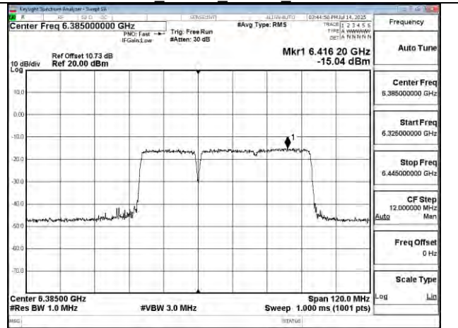
802.11be 80MHz Chain0 6385MHz 484+242 MRU1
