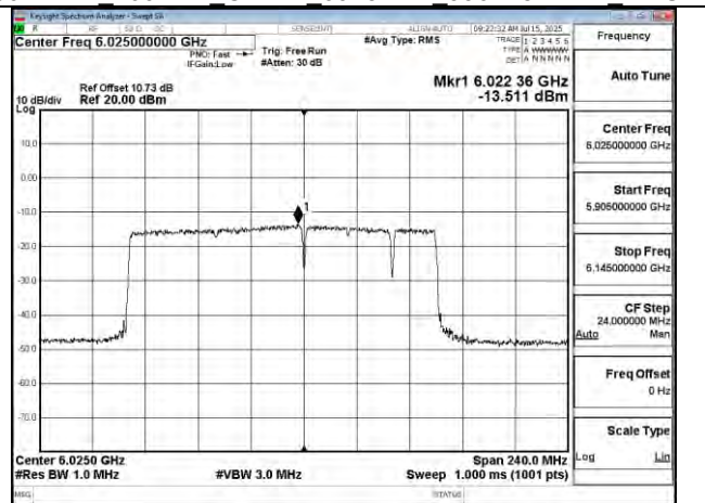
802.11be_160MHz_Chain1_6025MHz_996+484+242_MR08
