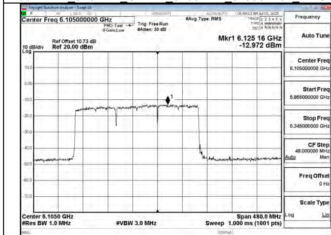
802.11be 320MHz Chain1 6105MHz 3x996 MRU4
