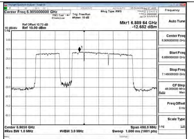
802.11be 320MHz Chain1 6905MHz 3x996+484 MRU3
