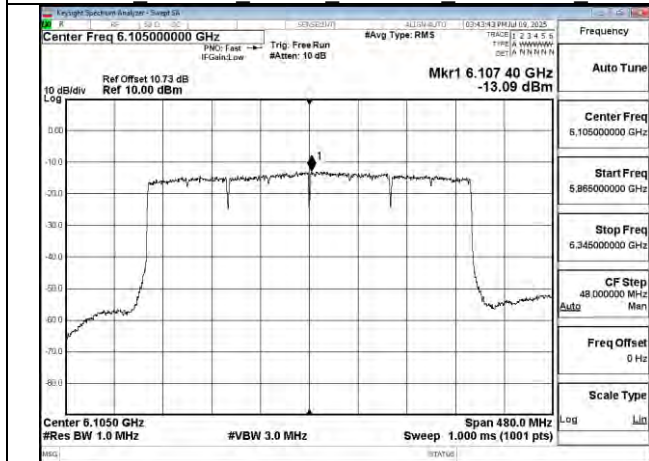
802.11be 320MHz Chain1 6105MHz
