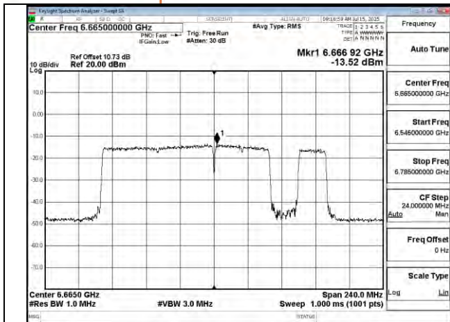
802.11be 160MHz Chain1 6665MHz 996+484+242 MRU7
