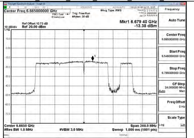
802.11be 160MHz Chain0 6665MHz 996+484+242 MRU7
