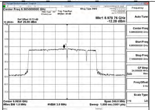
802.11be 160MHz Chain1 6985MHz 996+484+242 MRU8
