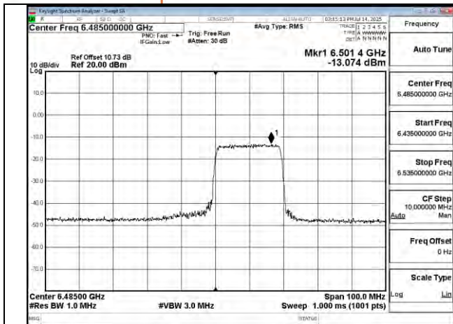
802.11be 40MHz Chain0 6485MHz RU242 62
