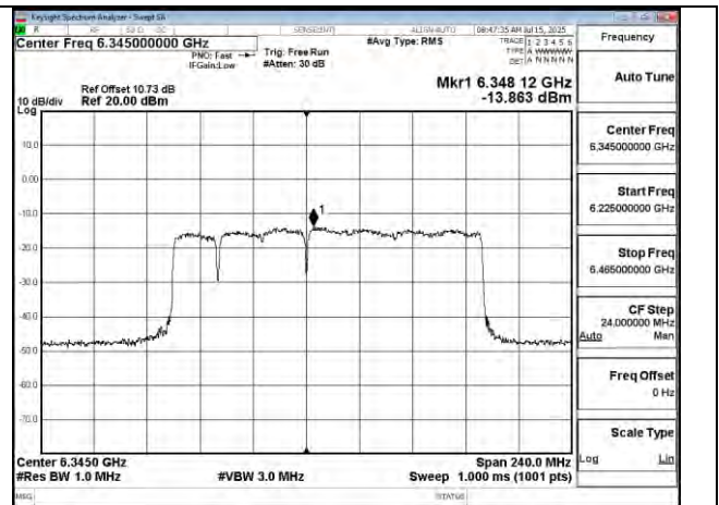
802.11be 160MHz Chain1 6345MHz 996+484+242 MRU1
