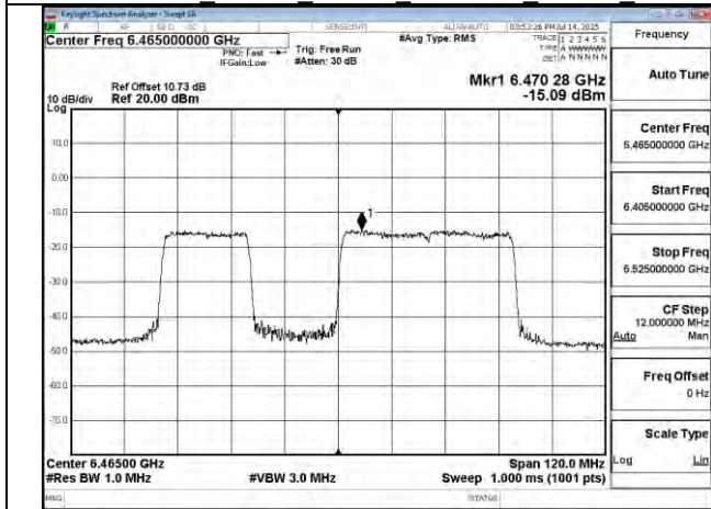
802.11be 80MHz Chain1 6465MHz 484+242 MRU2
