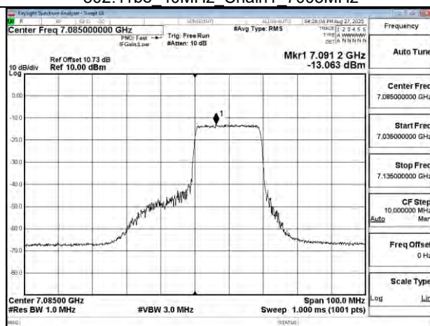
802.11be 40MHz Chain1 7085MHz RU242 62
