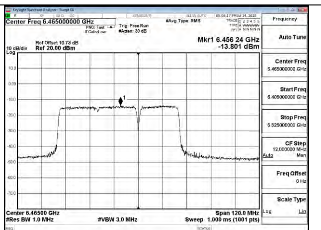
802.11be 80MHz Chain0 6465MHz 484+242 MRU4
