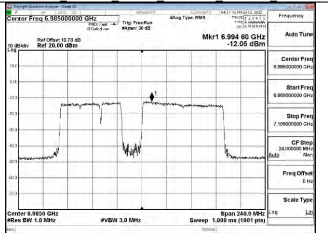
802.11be 160MHz Chain1 6985MHz 996+484+242 MRU4
