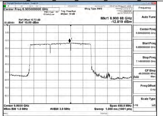
802.11be 320MHz Chain1 6905MHz 3x996 MRU4
