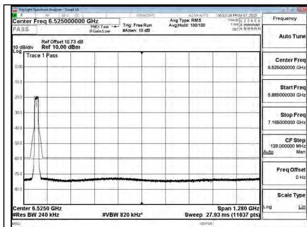
802.11a 20MHz Chain0 5955MHz
