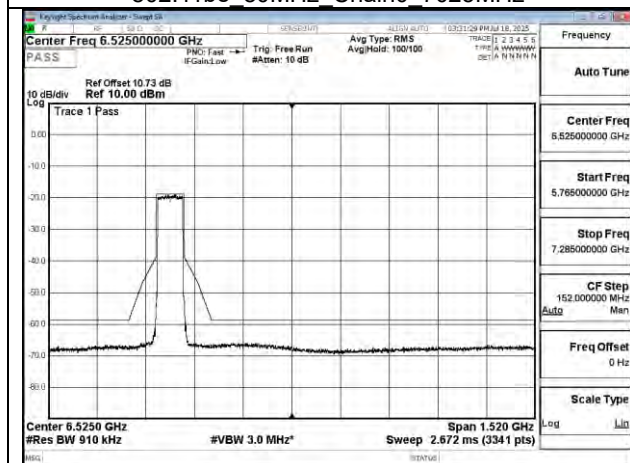
802.11be 80MHz Chain1 6145MHz
