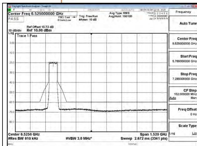
802.11ac 80MHz Chain1 6145MHz
