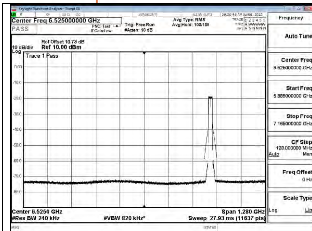
802.11n 20MHz Chain1 6875MHz
