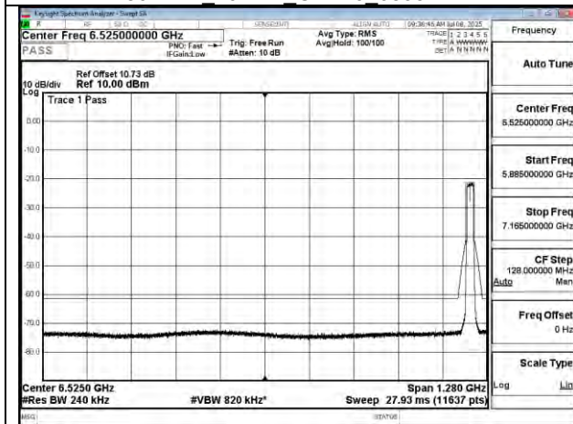
802.11n 20MHz Chain0 7115MHz
