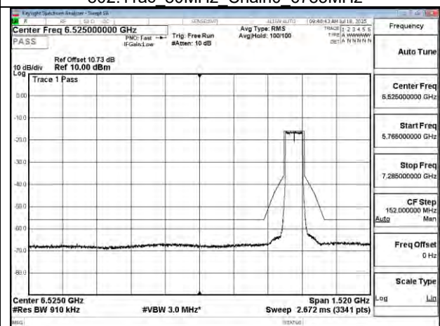
802.11ac 80MHz Chain0 6945MHz
