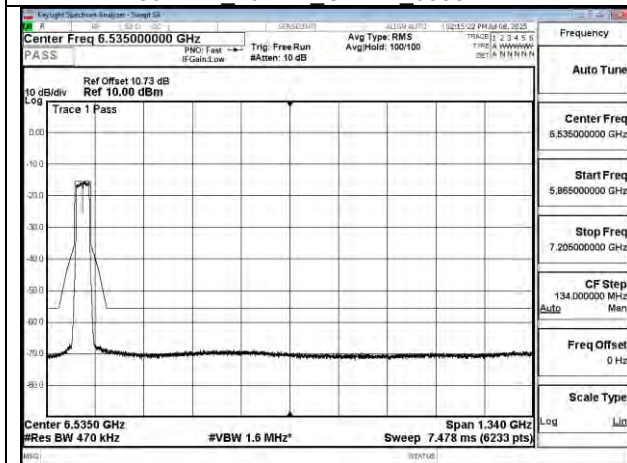
802.11n 40MHz Chain0 5965MHz
