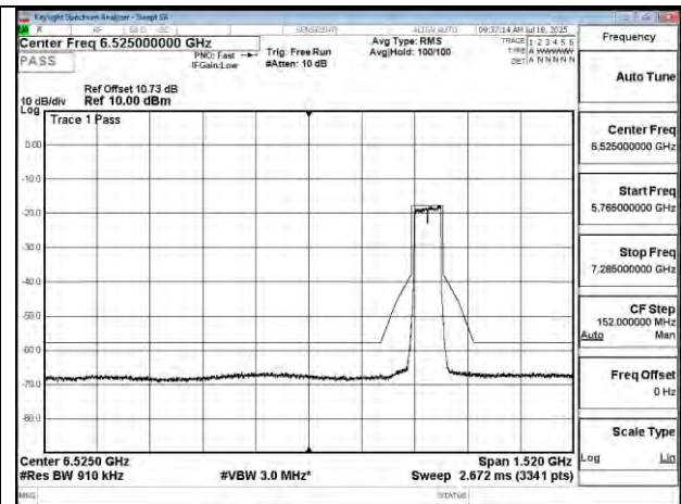
802.11ac 80MHz Chain1 6865MHz
