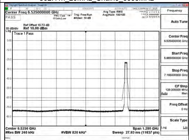
802.11n 20MHz Chain0 6875MHz
