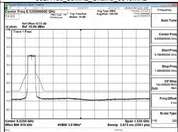
802.11ac 80MHz Chain1 5985MHz
