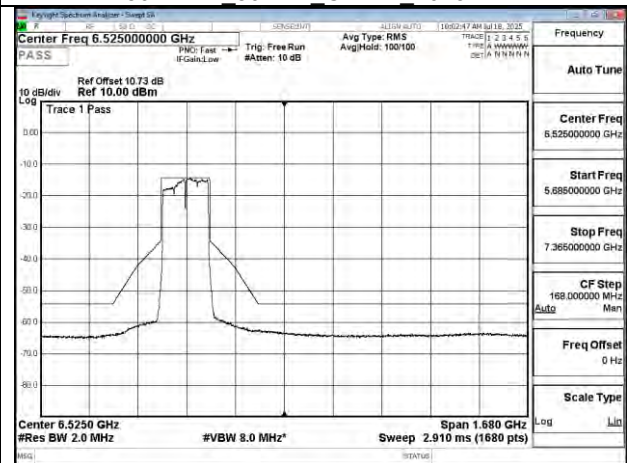
802.11ac 160MHz Chain0 6185MHz
