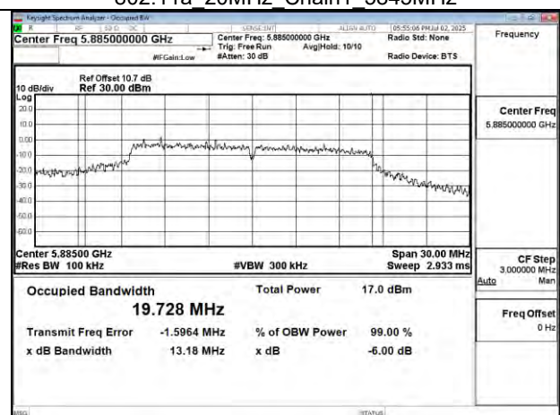
802.11a 20MHz Chain1 5885MHz
