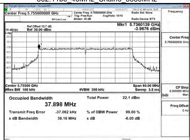
802.11be 40MHz Chain0 5755MHz
