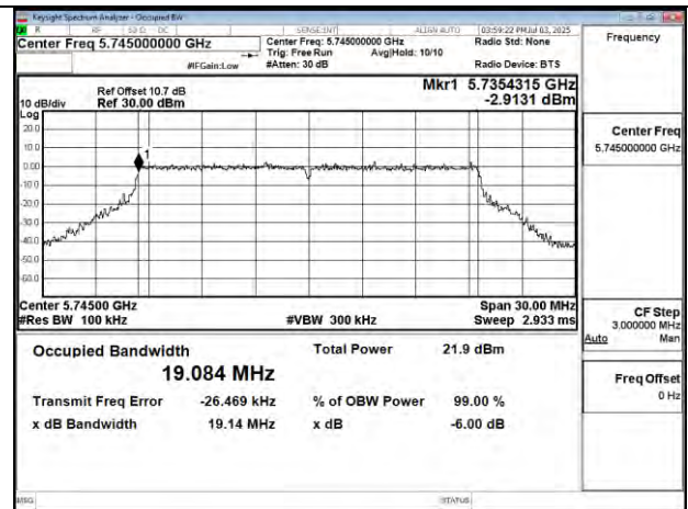
802.11be 20MHz Chain0 5745MHz
