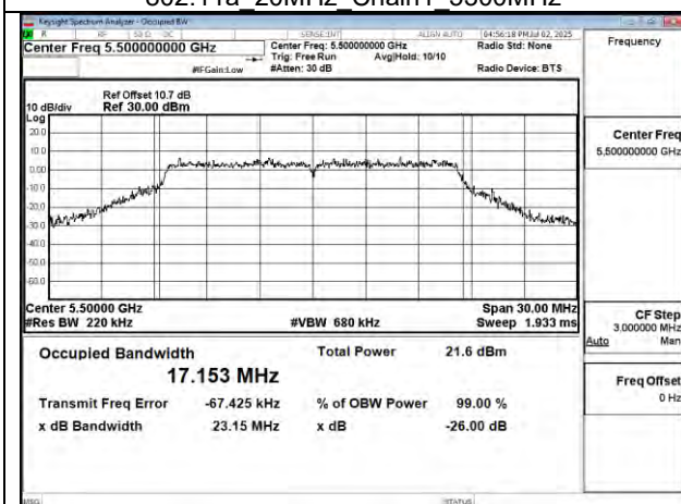
802.11a 20MHz Chain1 5500MHz
