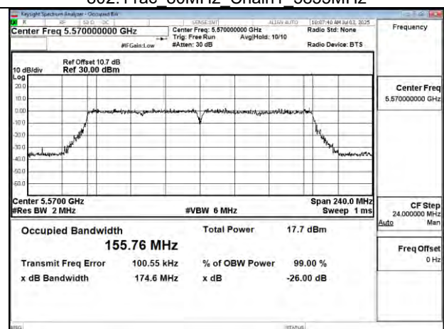
802.11ac 160MHz Chain0 5570MHz
