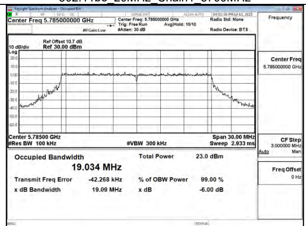
802.11be 20MHz Chain1 5785MHz
