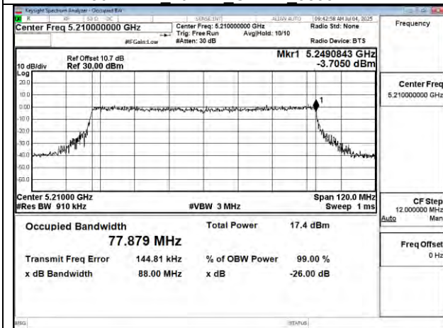
802.11be 80MHz Chain0 5210MHz
