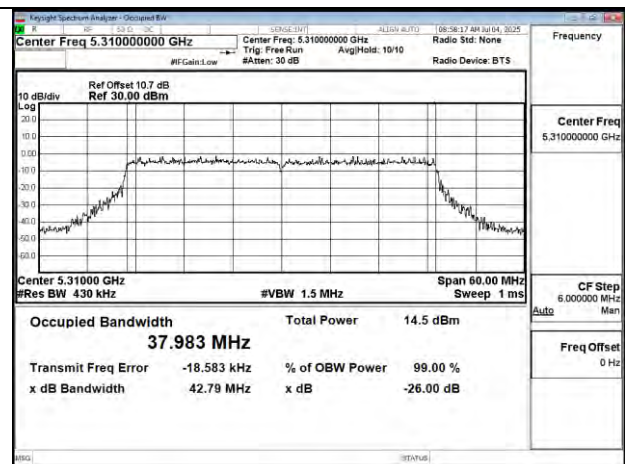
802.11be 40MHz Chain0 5310MHz
