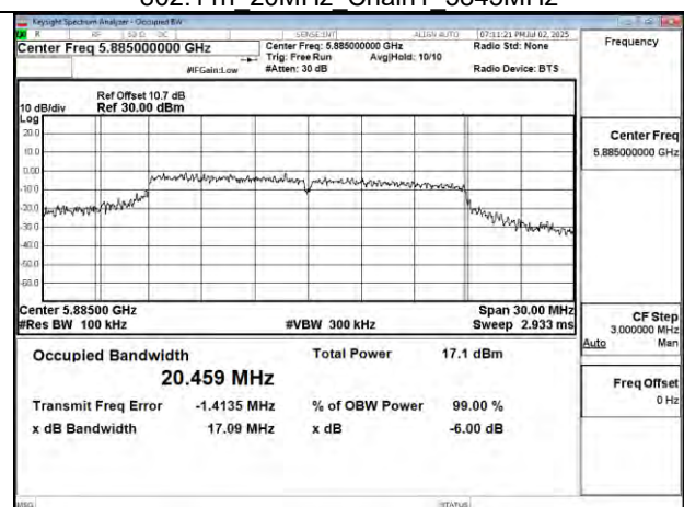
802.11n 20MHz Chain1 5885MHz
