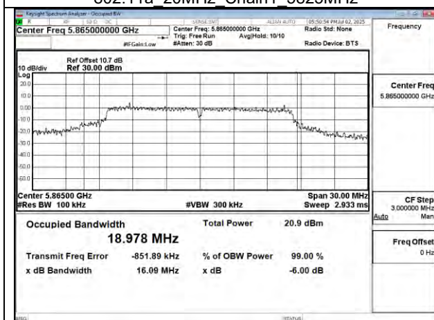
802.11a 20MHz Chain1 5865MHz
