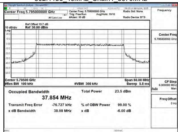
802.11be 40MHz Chain1 5795MHz
