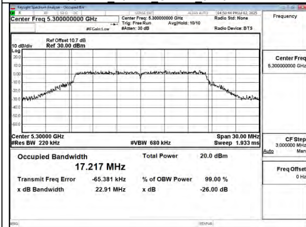
802.11a 20MHz Chain1 5300MHz
