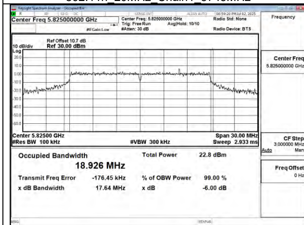
802.11n 20MHz Chain1 5825MHz
