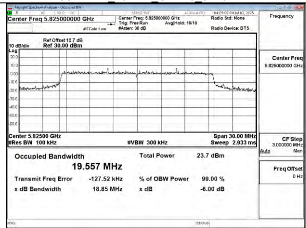
802.11be 20MHz Chain0 5825MHz
