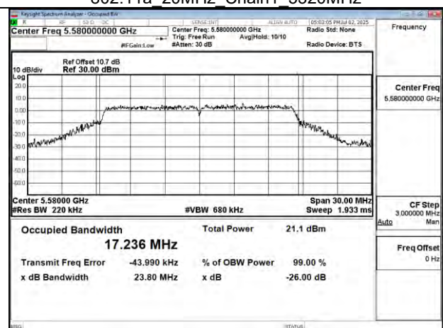
802.11a 20MHz Chain1 5580MHz
