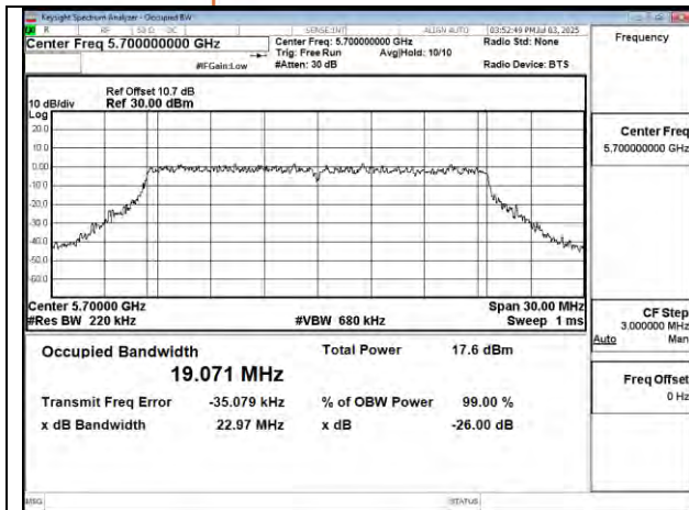
802.11be 20MHz Chain0 5700MHz
