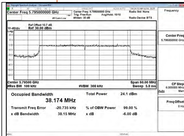
802.11be 40MHz Chain0 5795MHz
