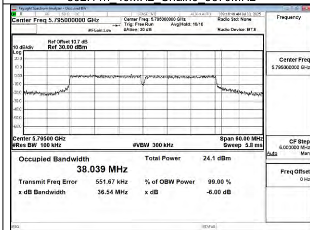
802.11n 40MHz Chain0 5795MHz
