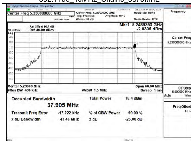
802.11be 40MHz Chain1 5230MHz
