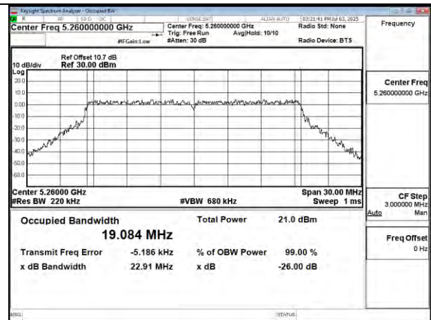
802.11be 20MHz Chain0 5260MHz
