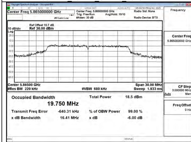
802.11a 20MHz Chain0 5865MHz
