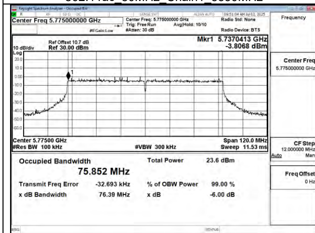
802.11ac 80MHz Chain1 5775MHz
