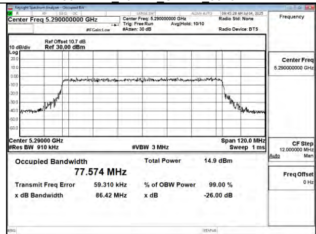
802.11be 80MHz Chain0 5290MHz
