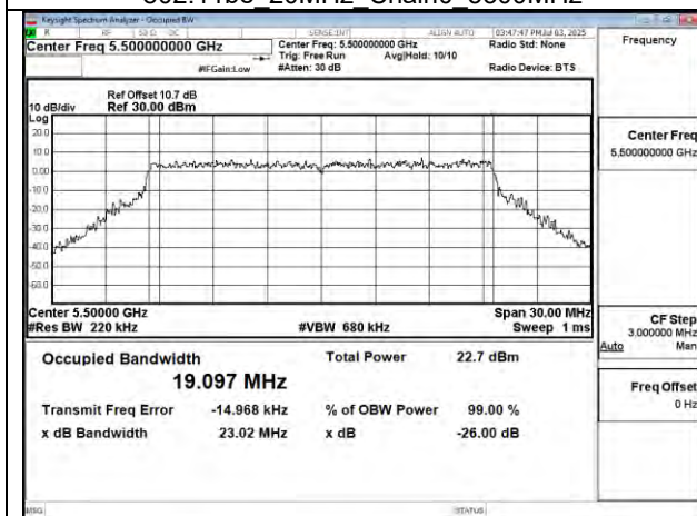
802.11be 20MHz Chain0 5500MHz
