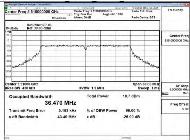
802.11n 40MHz Chain1 5510MHz
