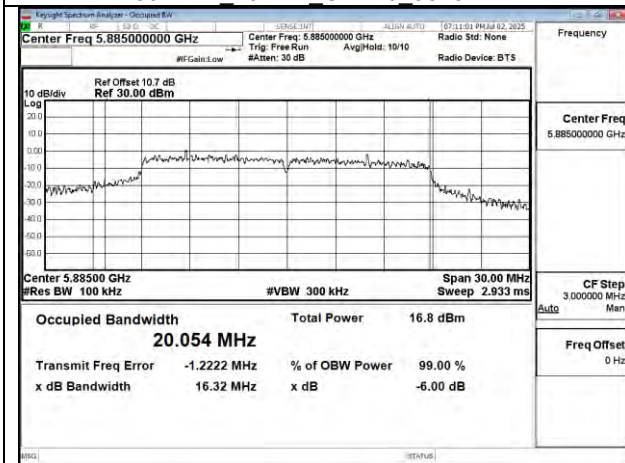
802.11n 20MHz Chain0 5885MHz
