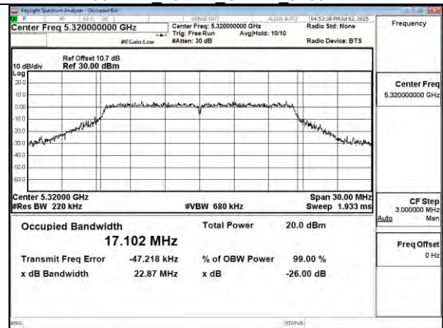
802.11a 20MHz Chain1 5320MHz
