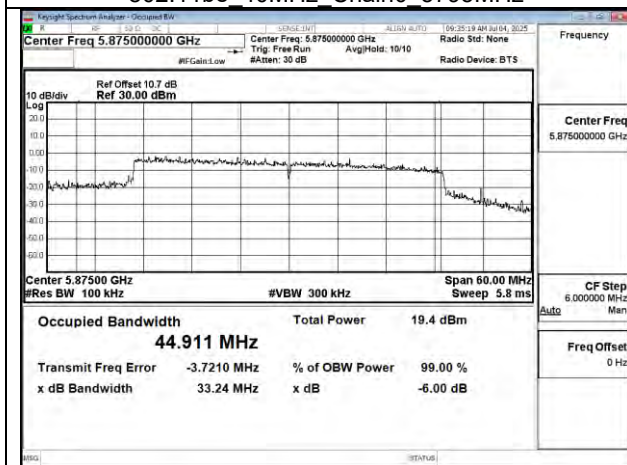
802.11be 40MHz Chain0 5875MHz
