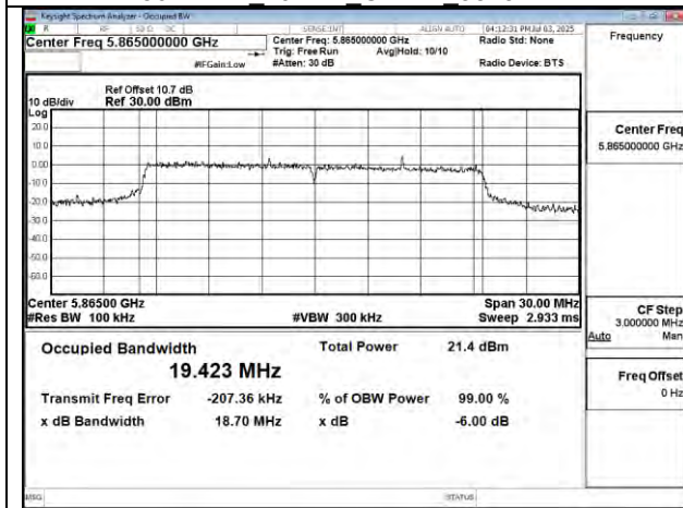
802.11be 20MHz Chain1 5865MHz
