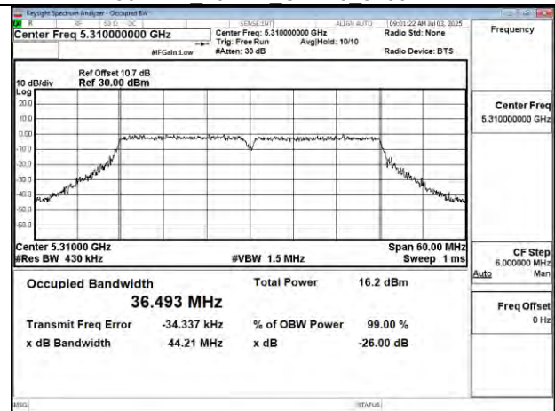
802.11n 40MHz Chain0 5310MHz
