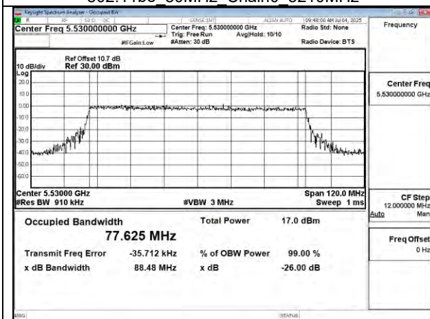
802.11be 80MHz Chain0 5530MHz
