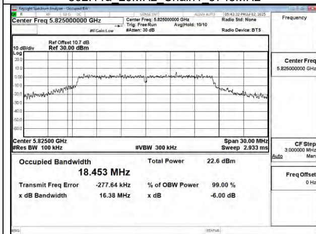
802.11a 20MHz Chain1 5825MHz
