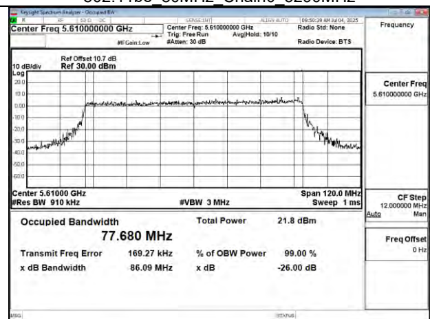
802.11be 80MHz Chain0 5610MHz
