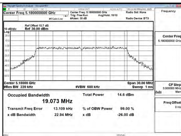
802.11be 20MHz Chain1 5180MHz
