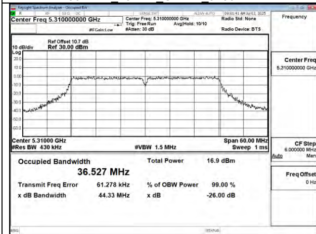
802.11n 40MHz Chain1 5310MHz
