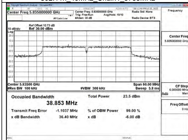
802.11n 40MHz Chain1 5835MHz
