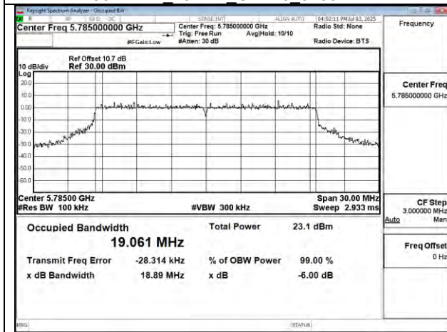
802.11be 20MHz Chain0 5785MHz
