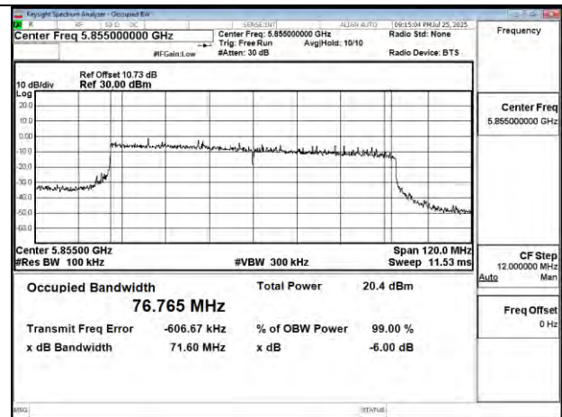
802.11be 80MHz Chain0 5855MHz
