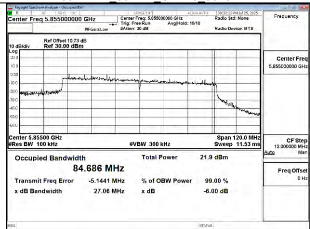
802.11ac 80MHz Chain0 5855MHz
