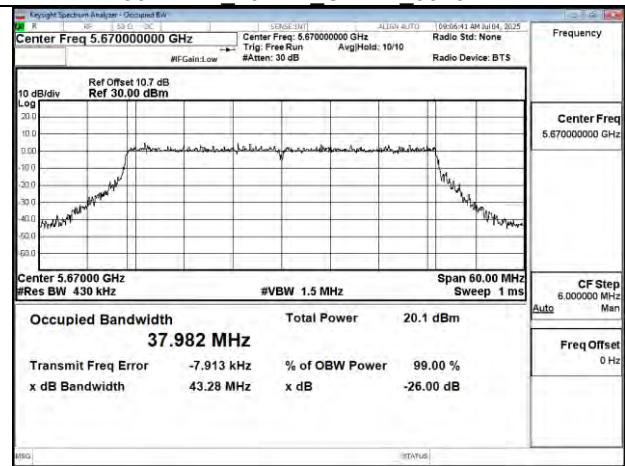
802.11be 40MHz Chain1 5670MHz
