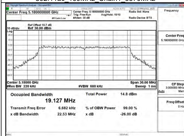
802.11be 20MHz Chain0 5180MHz
