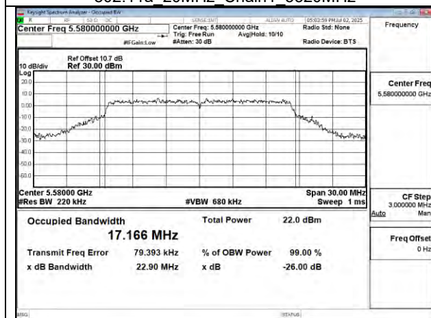
802.11a 20MHz Chain1 5580MHz
