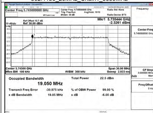
802.11be 20MHz Chain1 5745MHz
