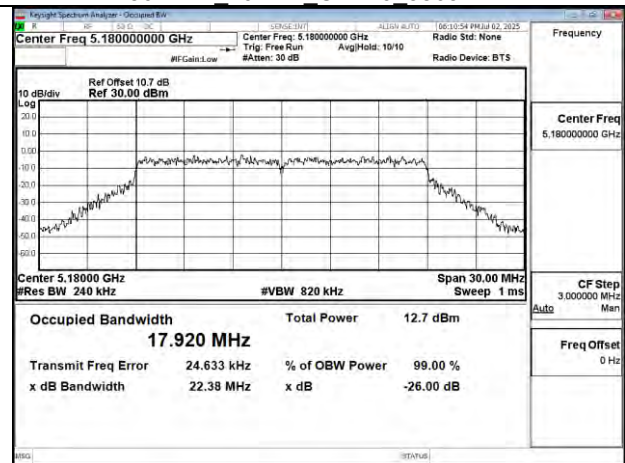
802.11n 20MHz Chain1 5180MHz
