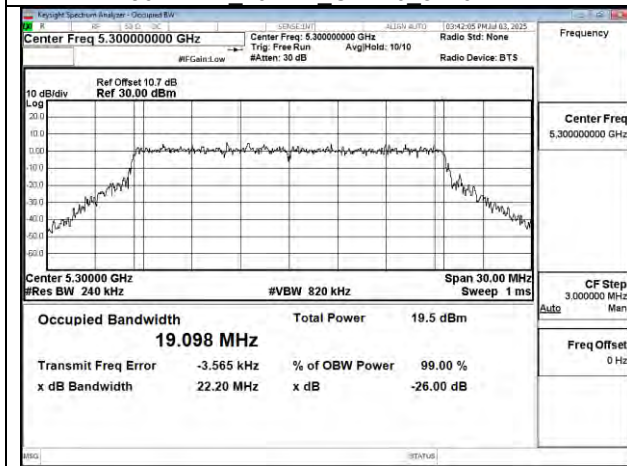
802.11be 20MHz Chain0 5300MHz
