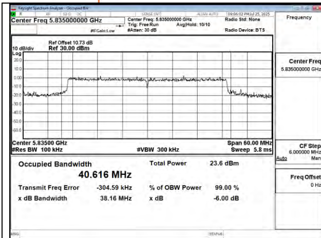
802.11be 40MHz Chain1 5835MHz
