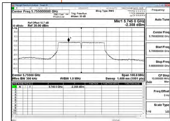
802.11n 40MHz Chain1 5755MHz
