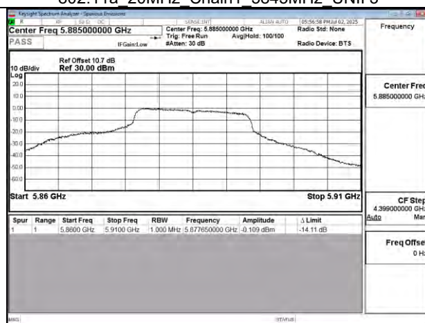
802.11a 20MHz Chain1 5885MHz
