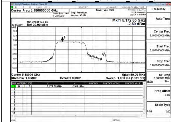
802.11be 20MHz Chain1 5180MHz 106+26 MRU1
