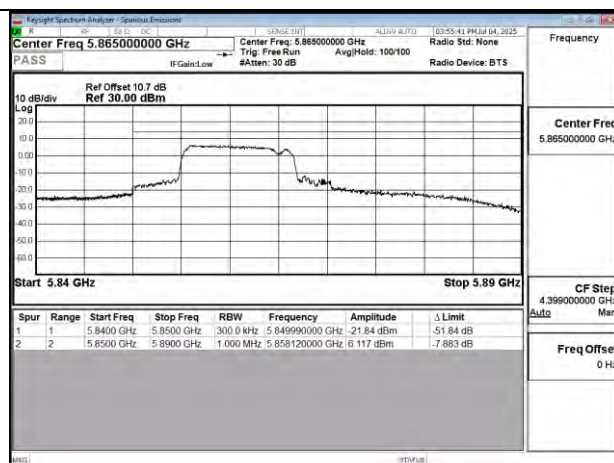
802.11be 20MHz Chain1 5865MHz 106+26 MRU1
