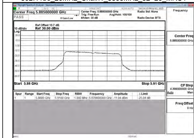
802.11be 20MHz Chain1 5885MHz
