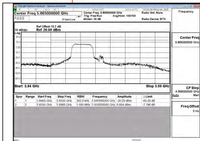
802.11be 20MHz Chain1 5865MHz 52+26 MRU1
