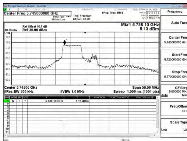
802.11be 20MHz Chain0 5745MHz 52+26 MRU1
