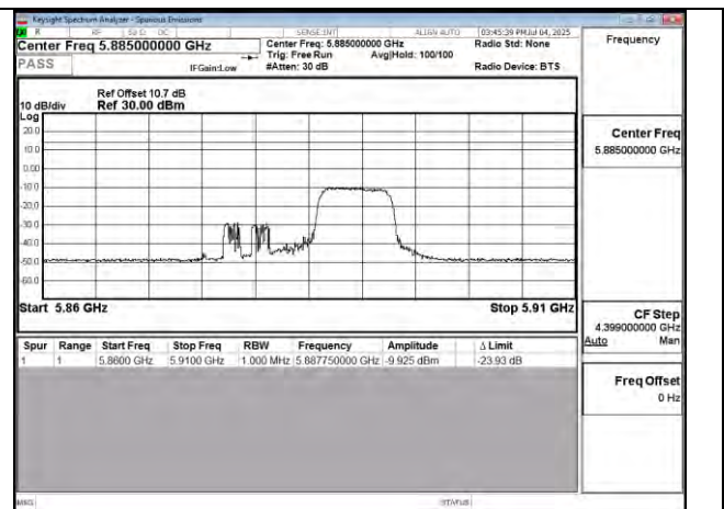
802.11be 20MHz Chain1 5885MHz 52+26 MRU3
