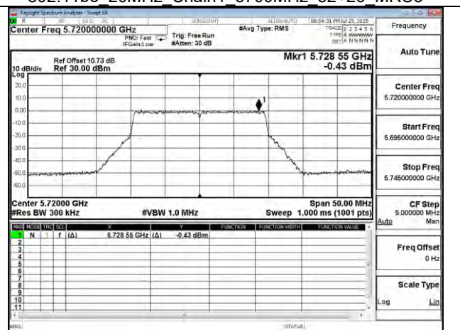
802.11be 20MHz Chain1 5720MHz UNII 3
