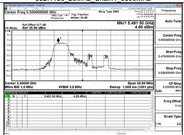
802.11be 20MHz Chain1 5500MHz RU52_37
