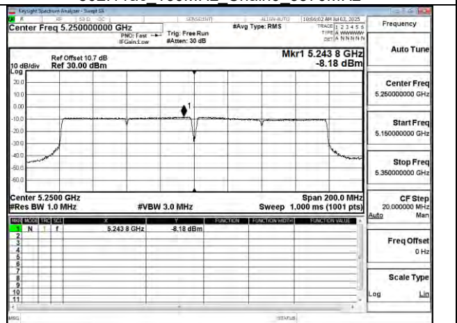
802.11ac 160MHz Chain1 5250MHz
