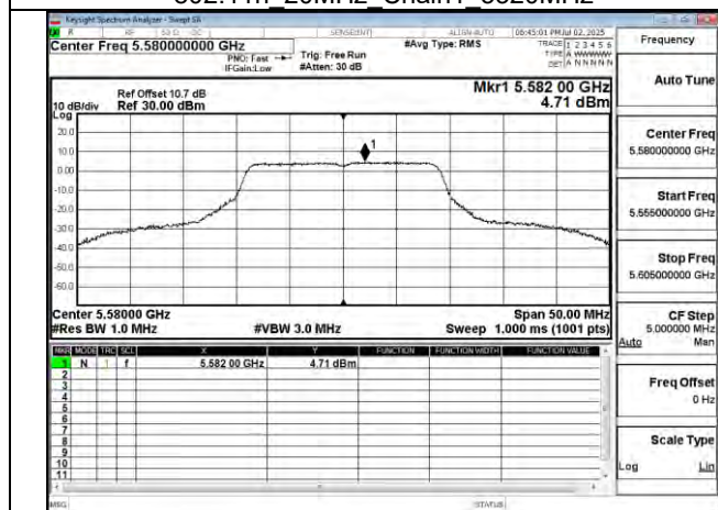
802.11n 20MHz Chain1 5580MHz
