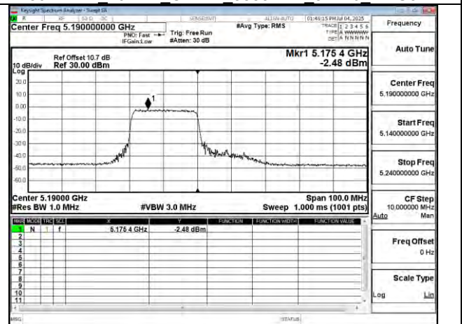
802.11be 40MHz Chain0 5190MHz RU242 61
