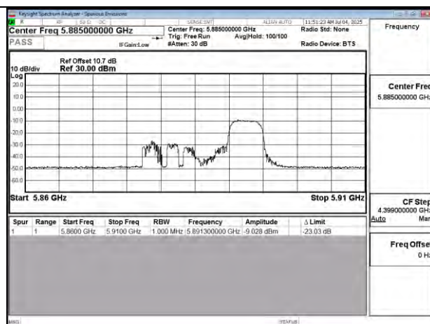
802.11be 20MHz Chain0 5885MHz RU52_40
