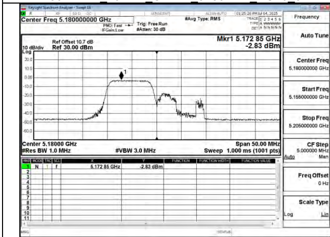
802.11be 20MHz Chain1 5180MHz RU106_53
