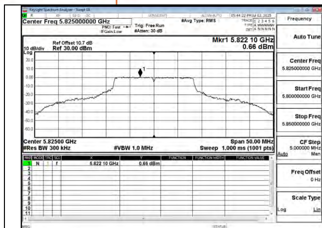
802.11a 20MHz Chain1 5825MHz
