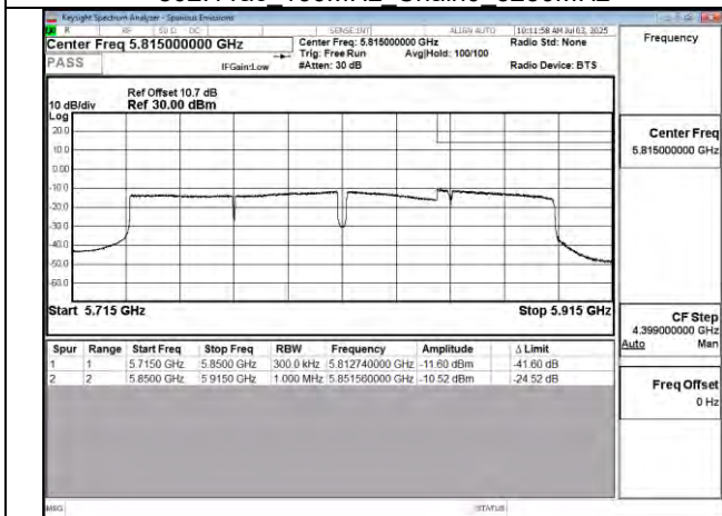
802.11ac 160MHz Chain0 5815MHz UNII 3
