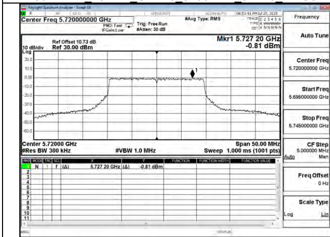
802.11be 20MHz Chain0 5720MHz UNII 3
