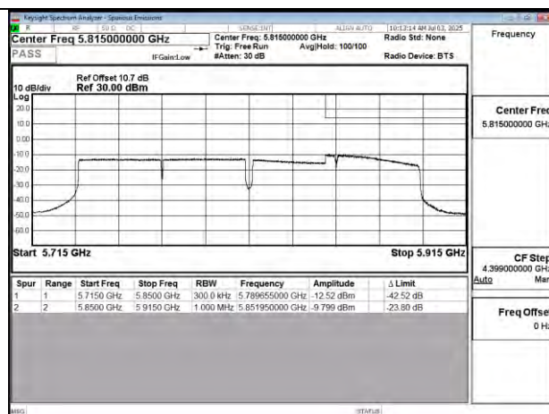
802.11ac 160MHz Chain1 5815MHz UNII 3
