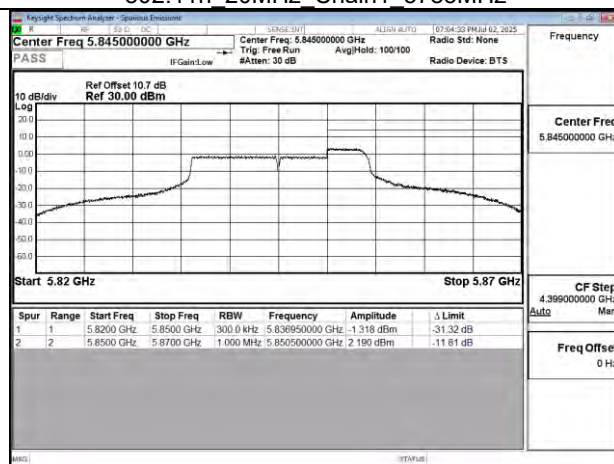
802.11n 20MHz Chain1 5845MHz UNII 3
