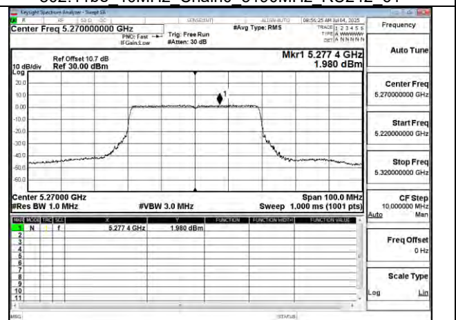
802.11be 40MHz Chain0 5270MHz
