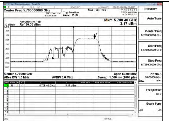
802.11be 20MHz Chain1 5700MHz RU106 54
