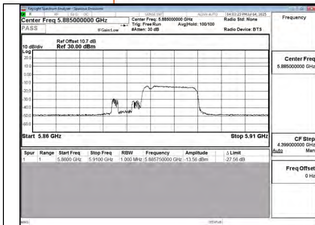
802.11be 20MHz Chain1 5885MHz 106+26 MRU2
