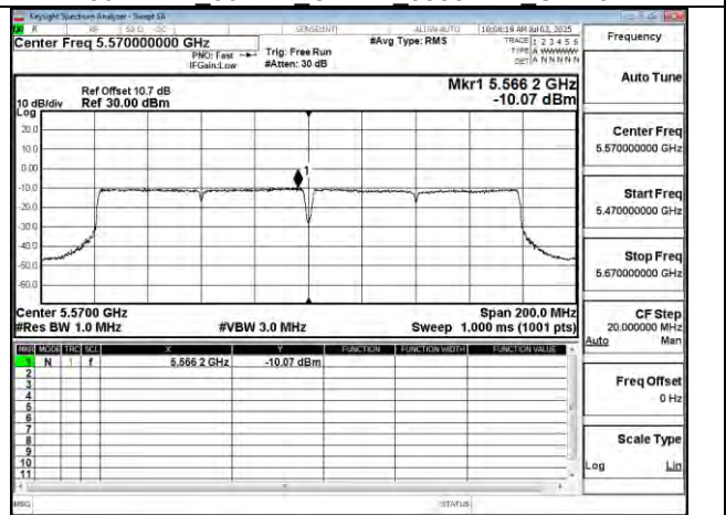
802.11ac 160MHz Chain0 5570MHz
