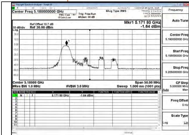
802.11be 20MHz Chain1 5180MHz RU26_0
