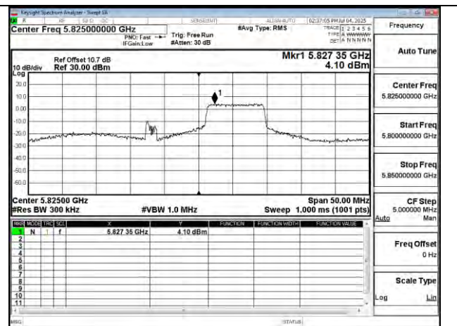
802.11be 20MHz Chain0 5825MHz RU106 54
