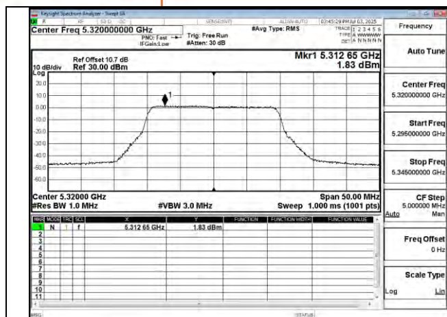
802.11be 20MHz Chain0 5320MHz
