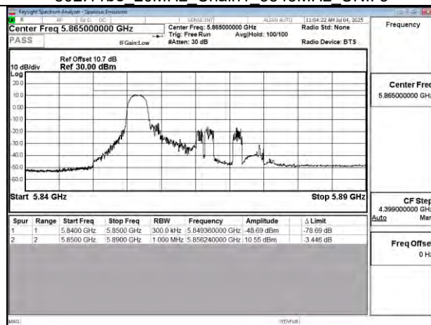
802.11be 20MHz Chain1 5865MHz RU26 0
