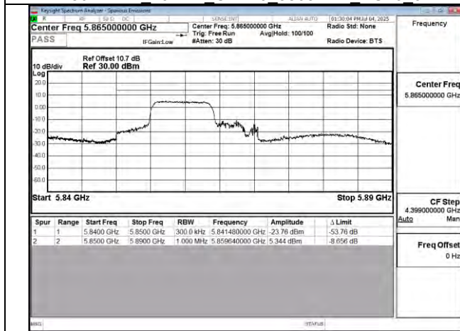
802.11be 20MHz Chain0 5865MHz RU106_53
