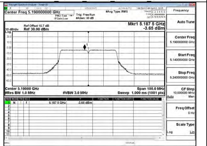
802.11n 40MHz Chain1 5190MHz
