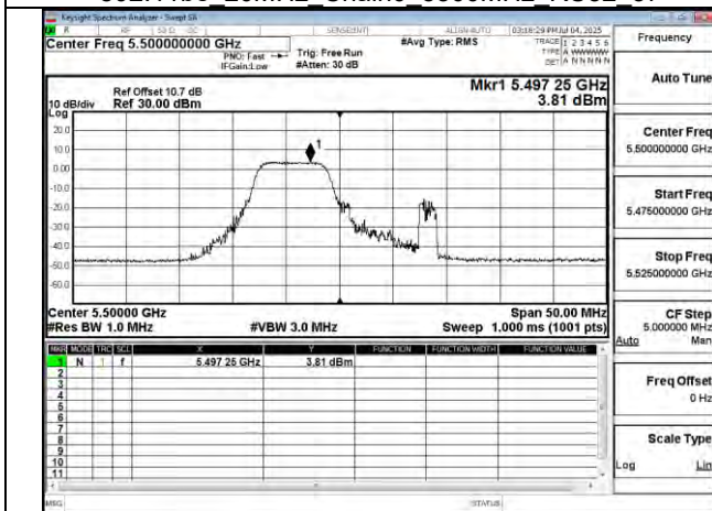
802.11be 20MHz Chain0 5500MHz 52+26 MRU1
