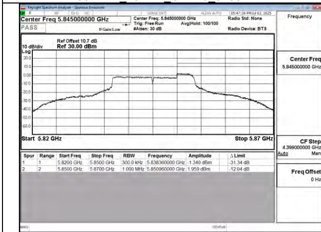
802.11a 20MHz Chain0 5845MHz UNII 3
