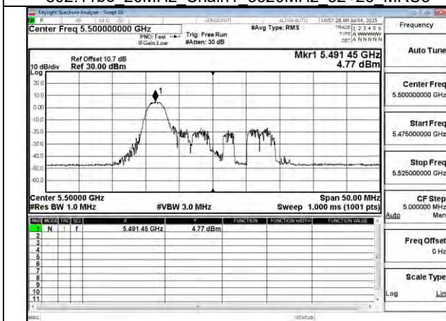
802.11be 20MHz Chain1 5500MHz RU26_0
