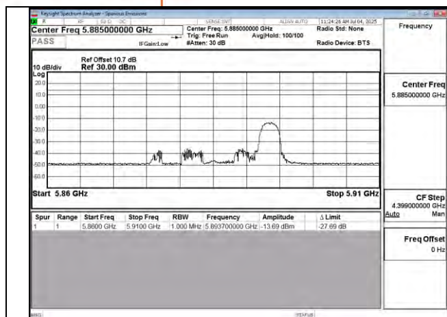
802.11be 20MHz Chain0 5885MHz RU26_8
