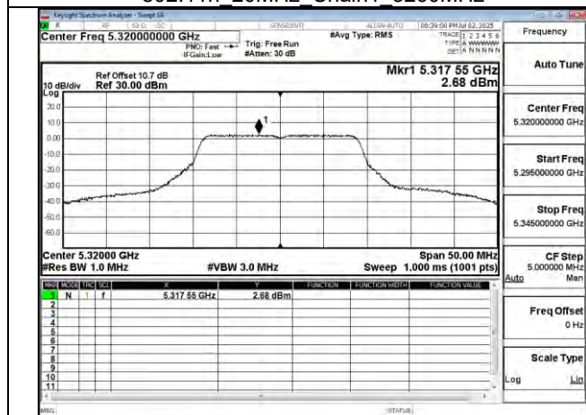
802.11n 20MHz Chain1 5320MHz
