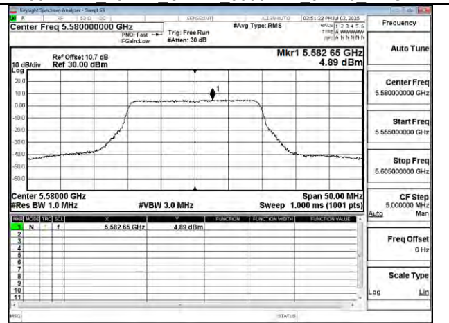
802.11be 20MHz Chain1 5580MHz
