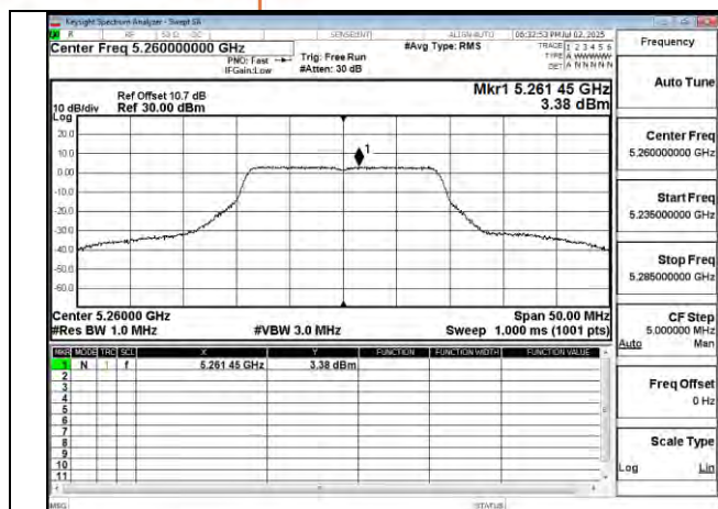
802.11n 20MHz Chain1 5260MHz
