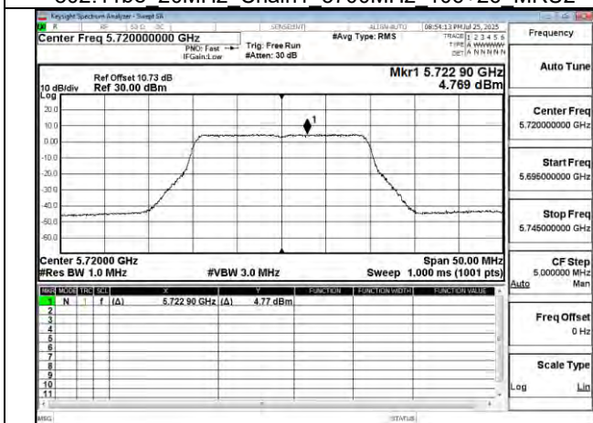
802.11be 20MHz Chain1 5720MHz UNII 2C
