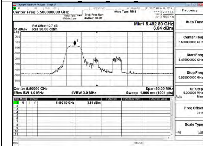
802.11be 20MHz Chain0 5500MHz RU52 37
