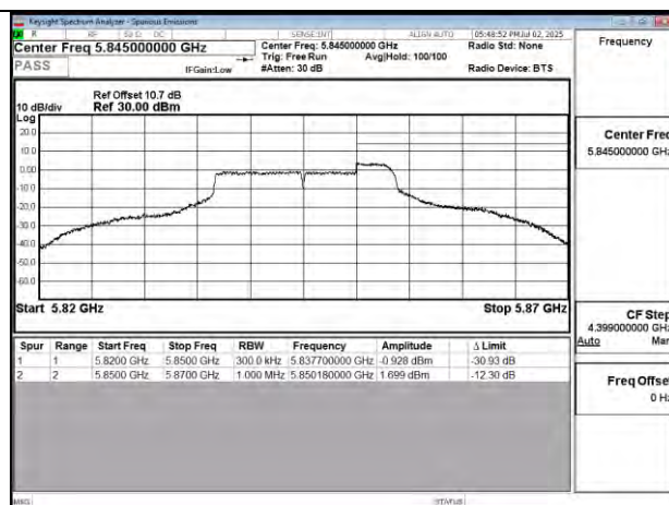
802.11a 20MHz Chain1 5845MHz UNII 3
