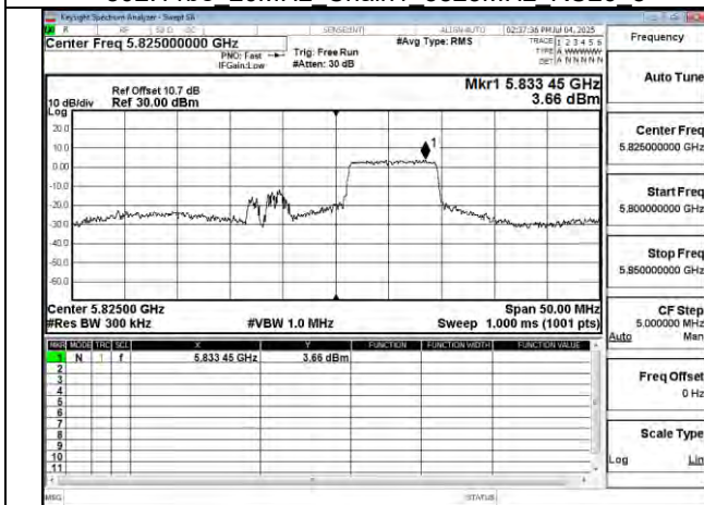
802.11be 20MHz Chain1 5825MHz RU106 54
