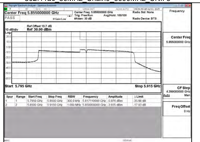
802.11ac 80MHz Chain0 5855MHz UNII 3
