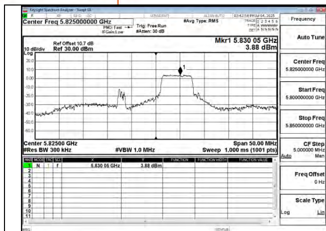
802.11be 20MHz Chain1 5825MHz 52+26 MRU3
