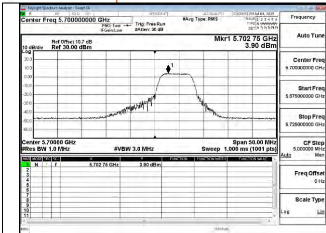
802.11be 20MHz Chain0 5700MHz 52+26 MRU3
