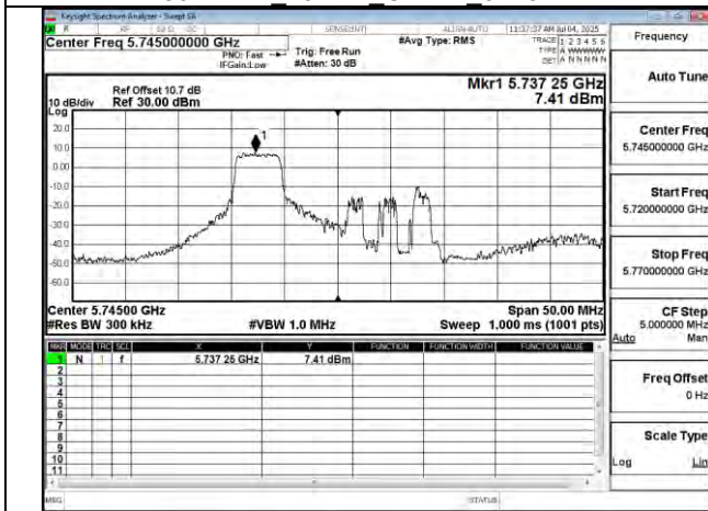
802.11be 20MHz Chain1 5745MHz RU52 37
