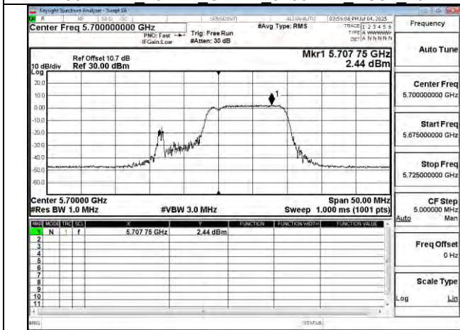
802.11be 20MHz Chain1 5700MHz 106+26 MRU2
