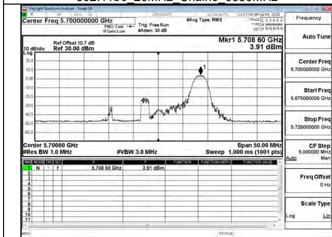
802.11be 20MHz Chain0 5700MHz RU26 8
