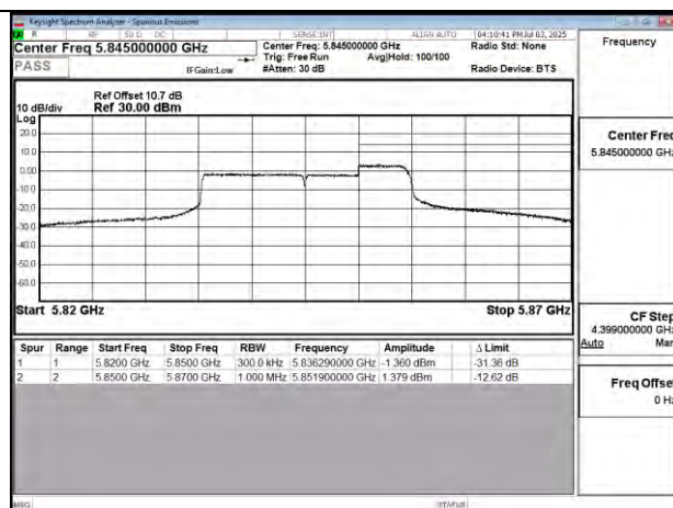
802.11be 20MHz Chain1 5845MHz UNII 3
