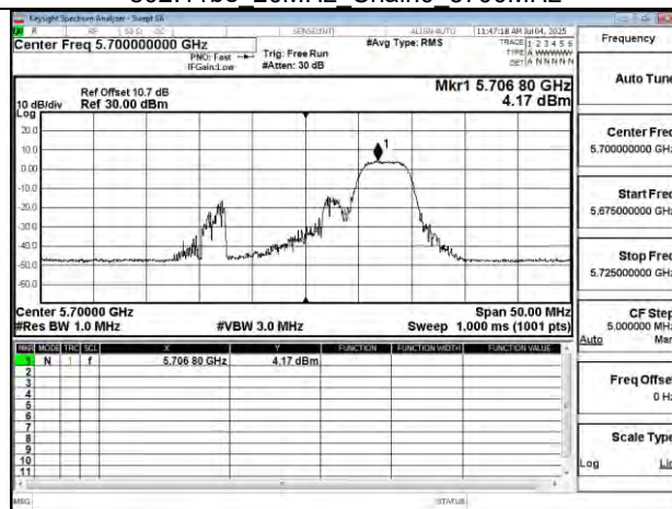
802.11be 20MHz Chain0 5700MHz RU52 40
