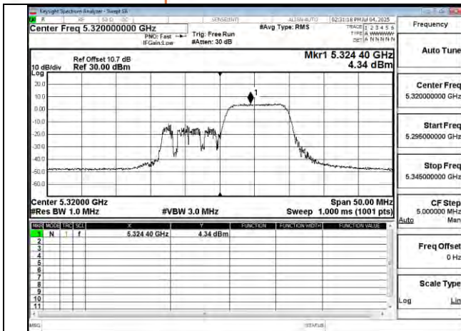
802.11be 20MHz Chain1 5320MHz RU106_54
