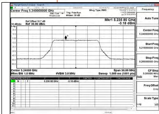
802.11be 20MHz Chain1 5240MHz
