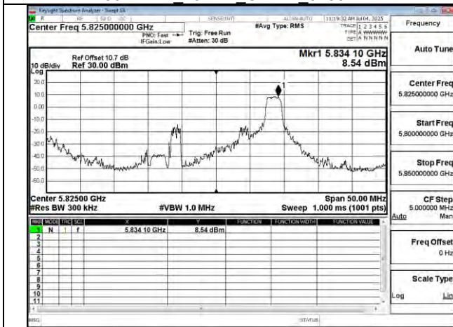
802.11be 20MHz Chain1 5825MHz RU26 8
