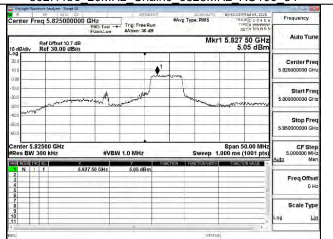
802.11be 20MHz Chain0 5825MHz 52+26 MRU3
