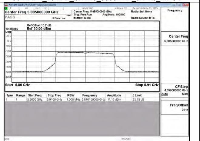
802.11be 20MHz Chain0 5885MHz
