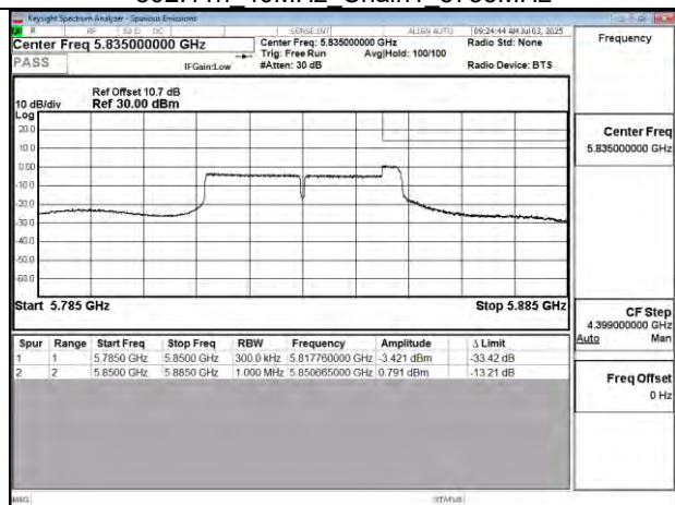
802.11n 40MHz Chain1 5835MHz UNII 3
