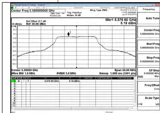
802.11a 20MHz Chain1 5580MHz
