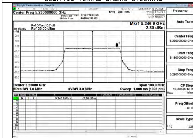
802.11be 40MHz Chain0 5230MHz
