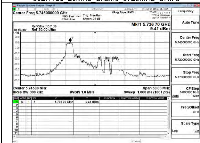
802.11be 20MHz Chain0 5745MHz RU26_0
