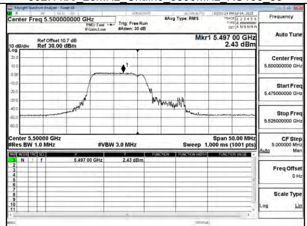
802.11be 20MHz Chain0 5500MHz 106+26 MRU1
