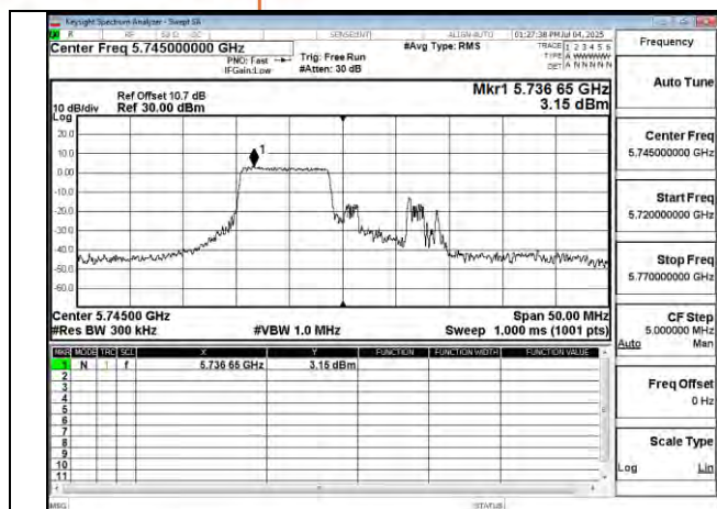
802.11be 20MHz Chain0 5745MHz RU106_53
