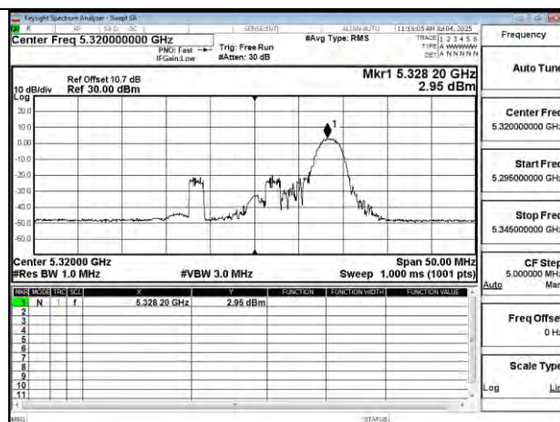
802.11be 20MHz Chain0 5320MHz RU26 8
