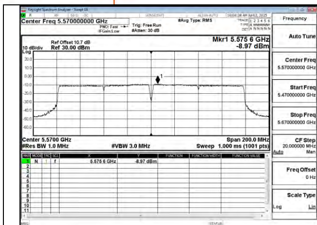
802.11ac 160MHz Chain1 5570MHz
