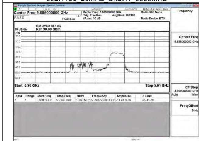
802.11be 20MHz Chain1 5885MHz RU52 40
