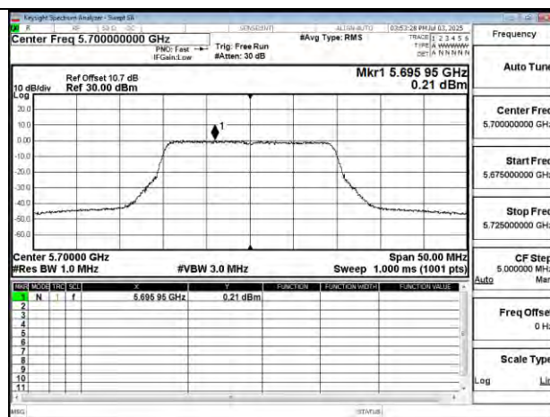
802.11be 20MHz Chain0 5700MHz
