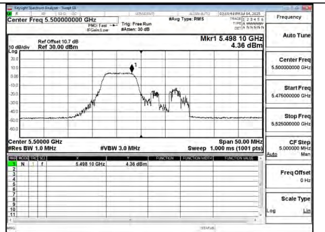
802.11be 20MHz Chain1 5500MHz 52+26 MRU1
