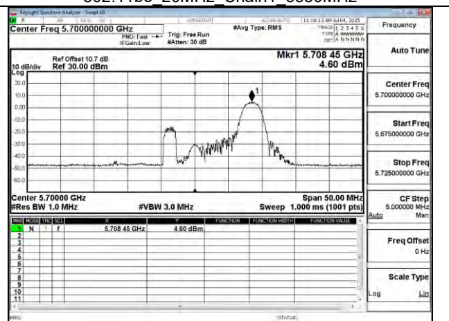
802.11be 20MHz Chain1 5700MHz RU26_8
