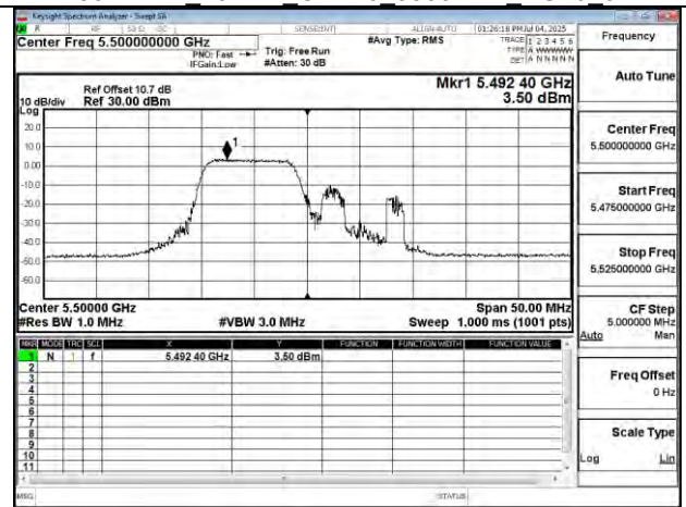
802.11be 20MHz Chain0 5500MHz RU106 53
