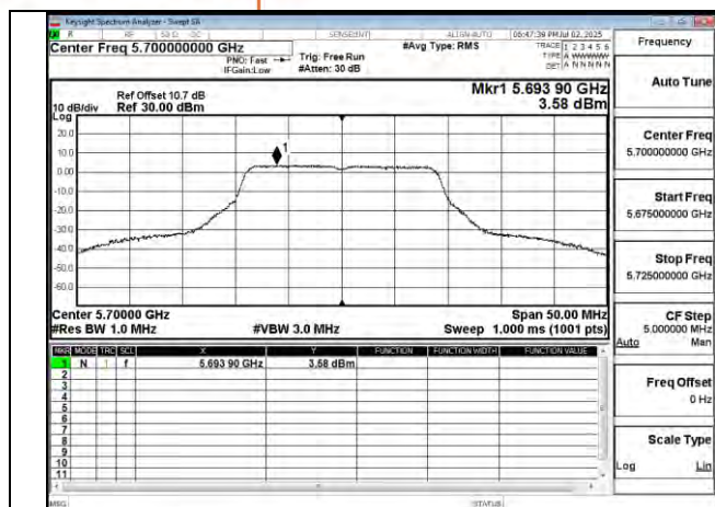
802.11n 20MHz Chain0 5700MHz
