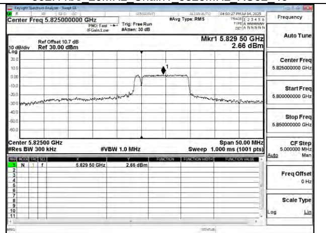
802.11be 20MHz Chain1 5825MHz 106+26 MRU2
