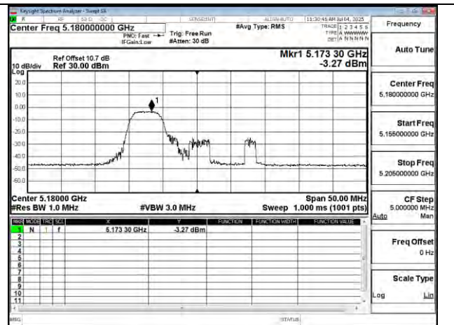
802.11be 20MHz Chain1 5180MHz RU52_37
