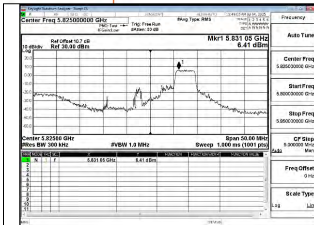
802.11be 20MHz Chain0 5825MHz RU52 40
