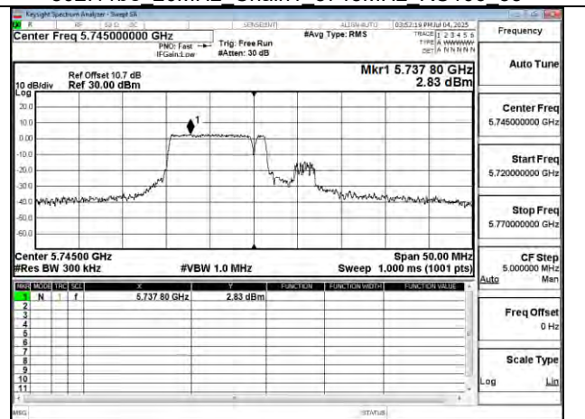
802.11be 20MHz Chain1 5745MHz 106+26 MRU1
