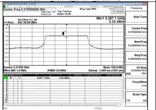
802.11n 40MHz Chain1 5270MHz
