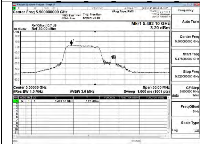
802.11be 20MHz Chain1 5500MHz 106+26 MRU1
