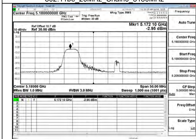
802.11be 20MHz Chain0 5180MHz RU52 37
