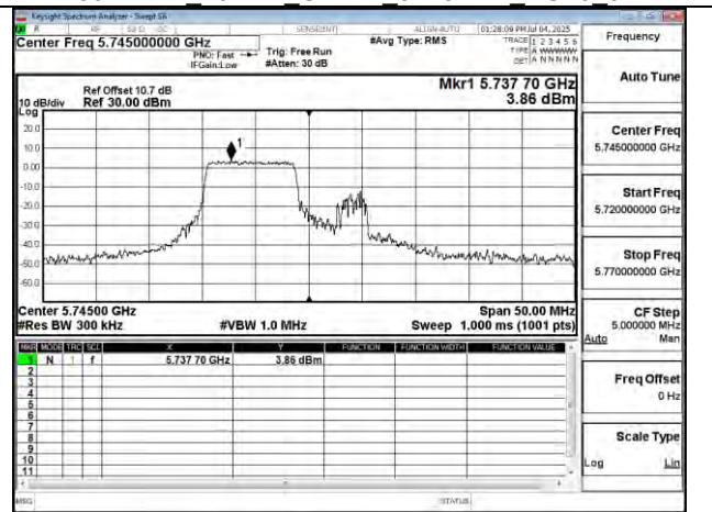
802.11be 20MHz Chain1 5745MHz RU106 53
