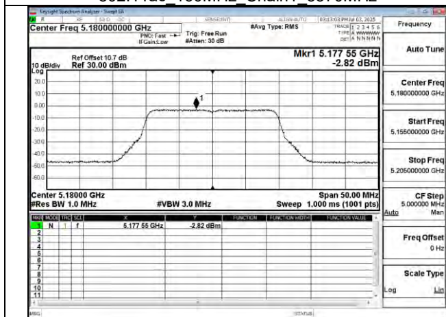
802.11be 20MHz Chain0 5180MHz
