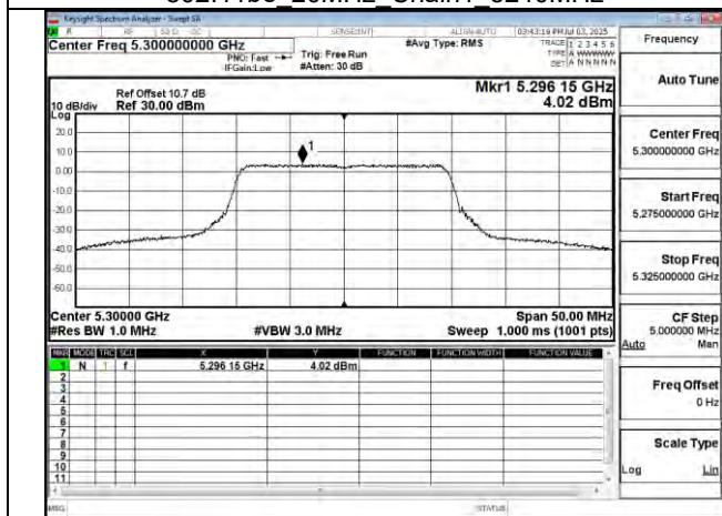
802.11be 20MHz Chain1 5300MHz
