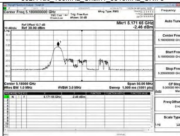
802.11be 20MHz Chain0 5180MHz RU26 0
