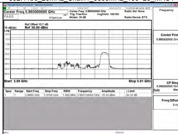
802.11be 20MHz Chain1 5885MHz RU26 8
