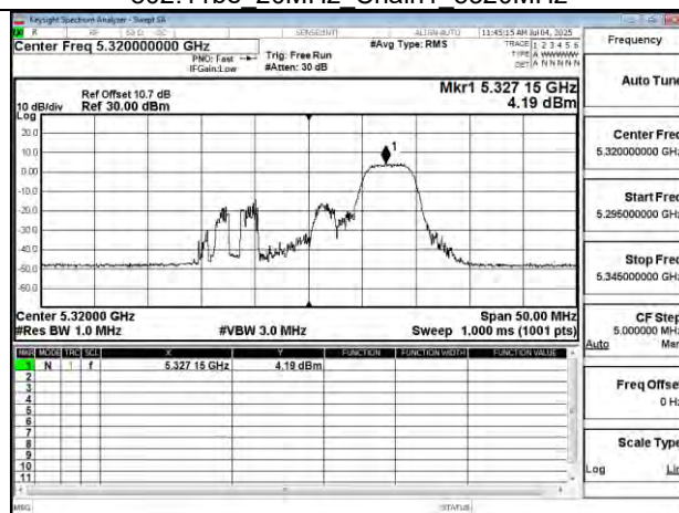
802.11be 20MHz Chain1 5320MHz RU52_40
