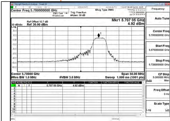
802.11be 20MHz Chain1 5700MHz RU52 40
