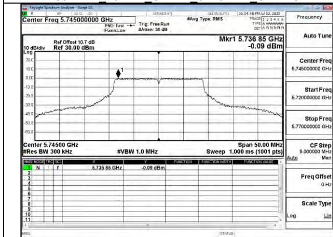
802.11n 20MHz Chain1 5745MHz
