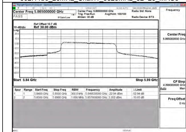
802.11be 20MHz Chain1 5865MHz
