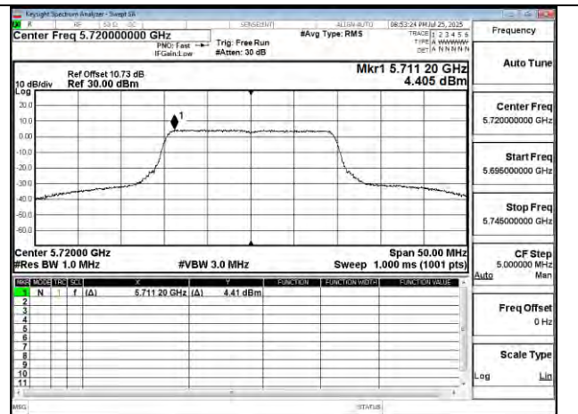
802.11be 20MHz Chain0 5720MHz UNII 2C
