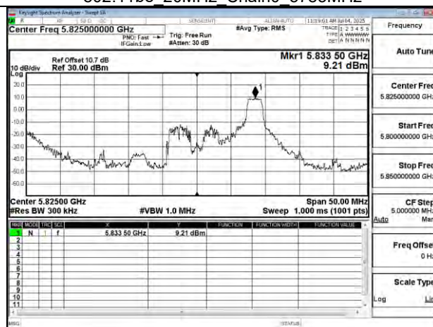
802.11be 20MHz Chain0 5825MHz RU26_8
