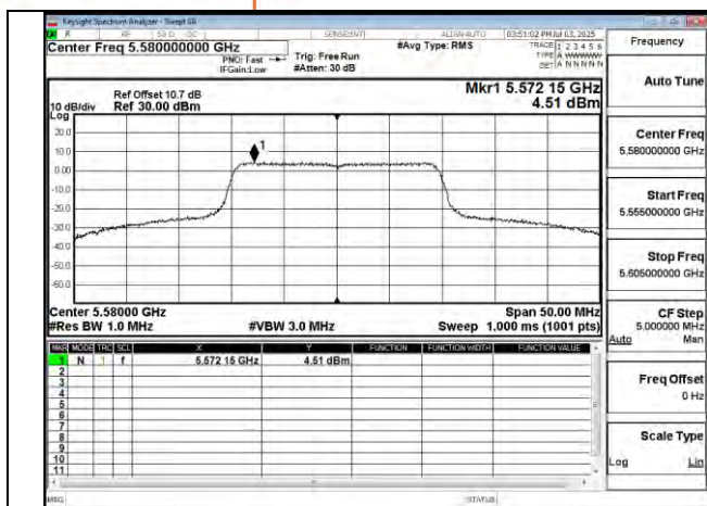
802.11be 20MHz Chain0 5580MHz
