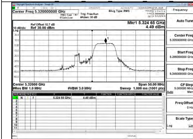
802.11be 20MHz Chain1 5320MHz 52+26 MRU3
