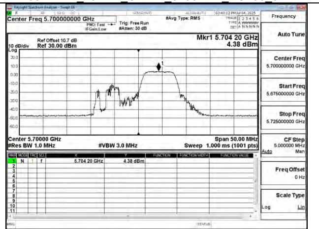
802.11be 20MHz Chain1 5700MHz 52+26 MRU3
