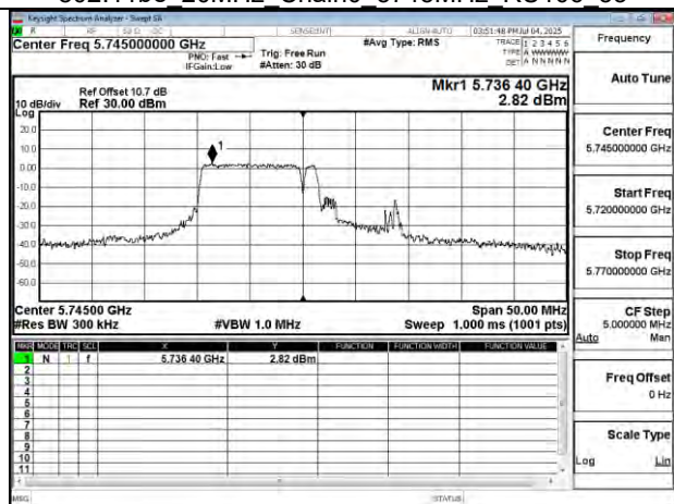
802.11be 20MHz Chain0 5745MHz 106+26 MRU1
