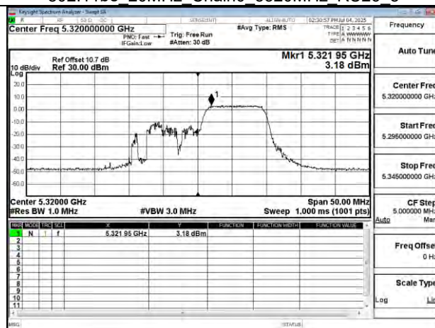
802.11be 20MHz Chain0 5320MHz RU106 54
