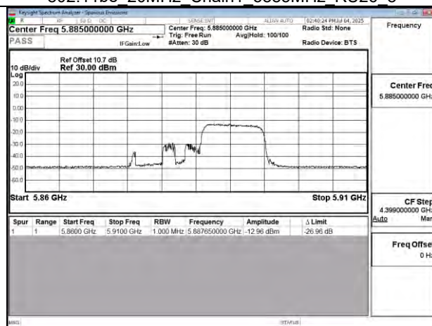
802.11be 20MHz Chain1 5885MHz RU106 54
