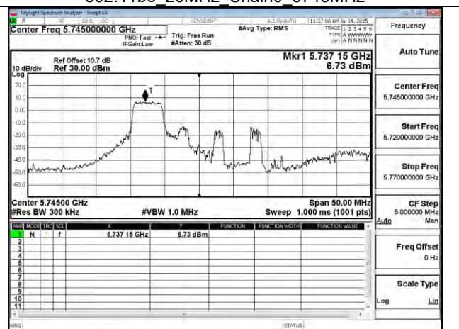
802.11be 20MHz Chain0 5745MHz RU52_37
