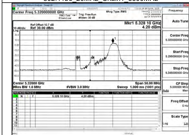
802.11be 20MHz Chain1 5320MHz RU26_8
