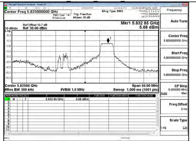
802.11be 20MHz Chain1 5825MHz RU52 40
