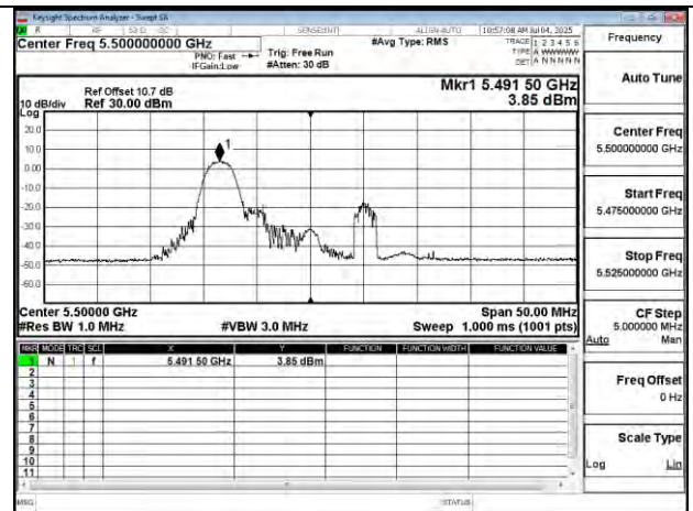
802.11be 20MHz Chain0 5500MHz RU26 0
