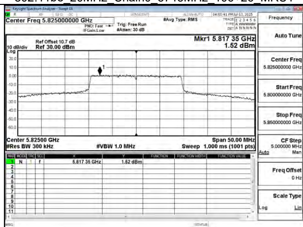
802.11be 20MHz Chain0 5825MHz
