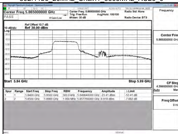
802.11be 20MHz Chain1 5865MHz RU106 53
