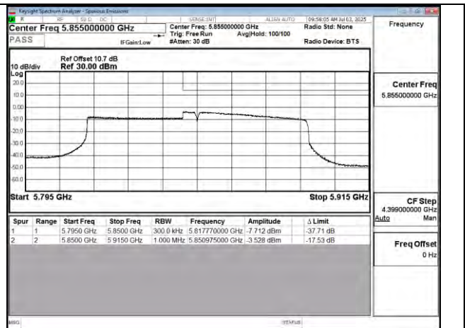
802.11ac 80MHz Chain1 5855MHz UNII 3
