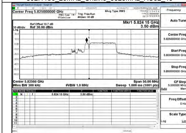
802.11be 20MHz Chain0 5825MHz 106+26 MRU2
