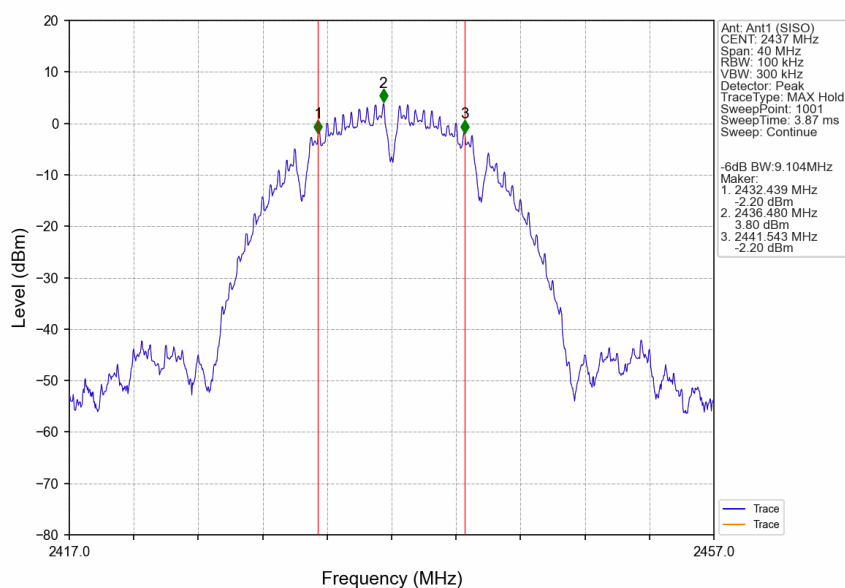
802.11b_MCH_2437MHz_Ant1 (SISO)_NTNV
