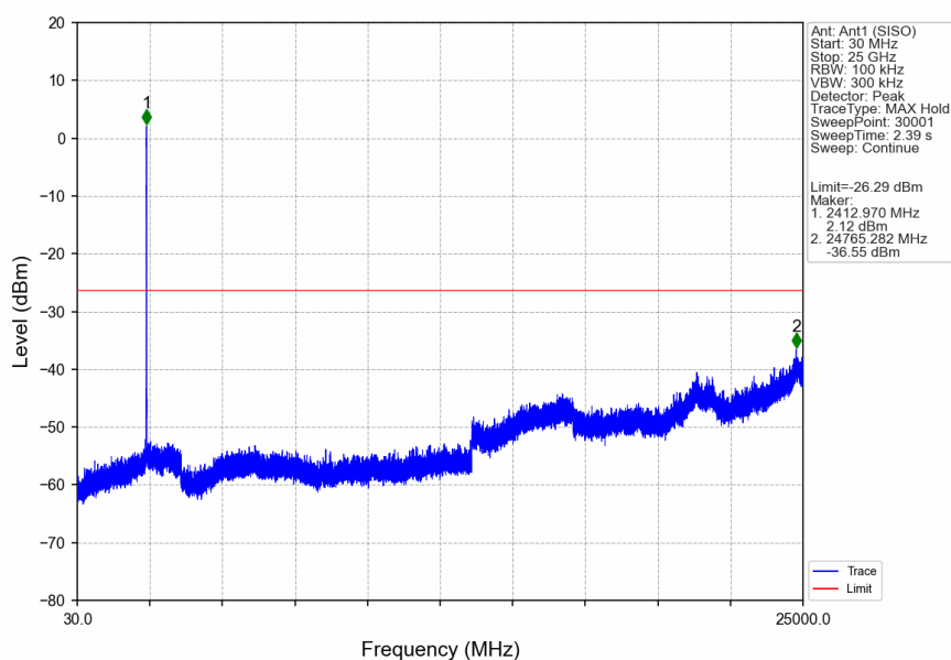
802.11b_LCH_2412MHz_Ant1 (SISO)_NTNV
